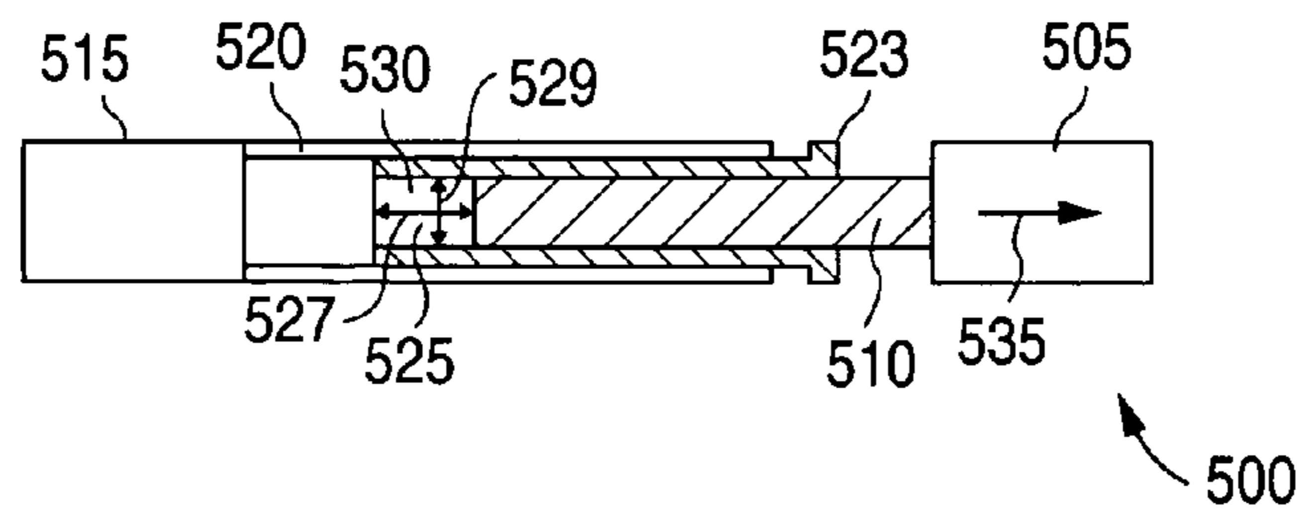
FIG. 12A
