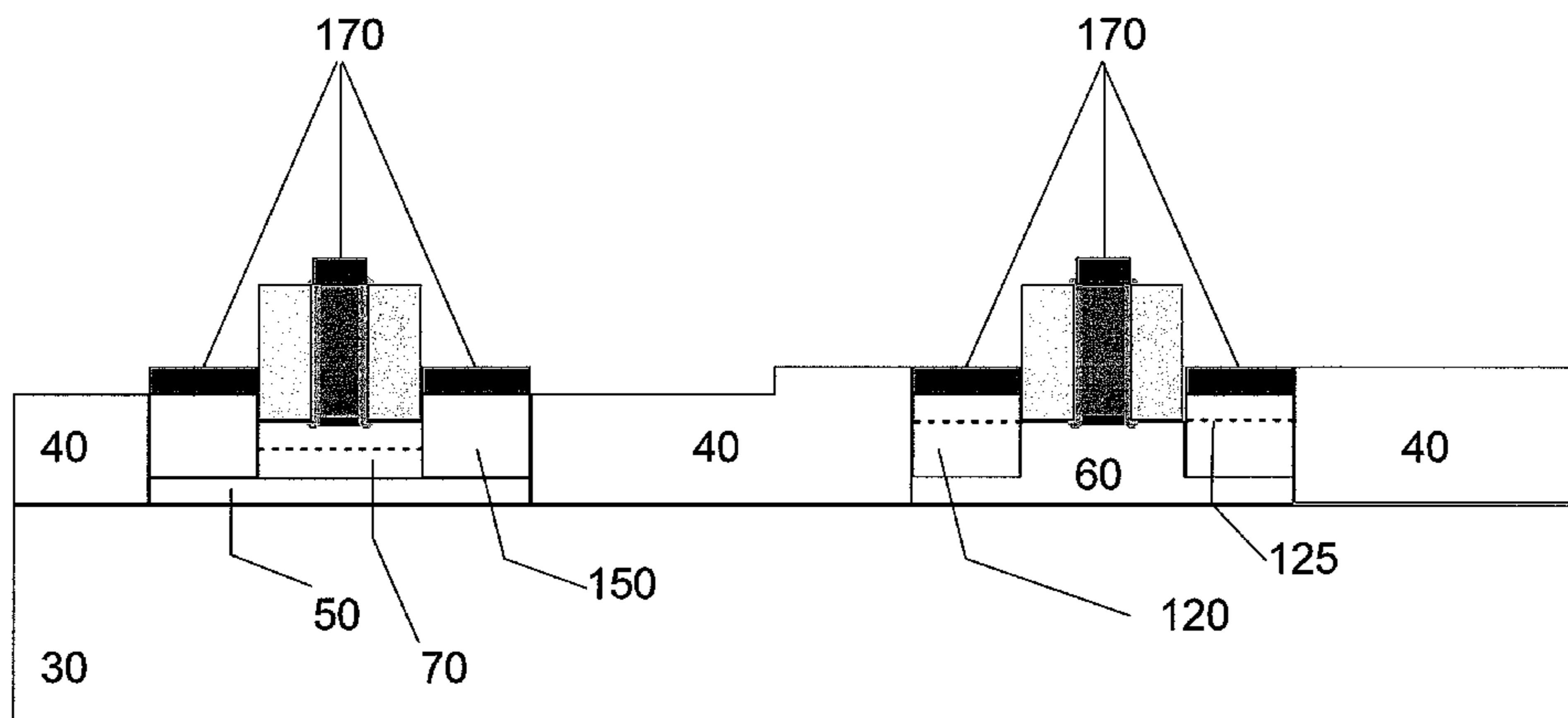
PFET 20
