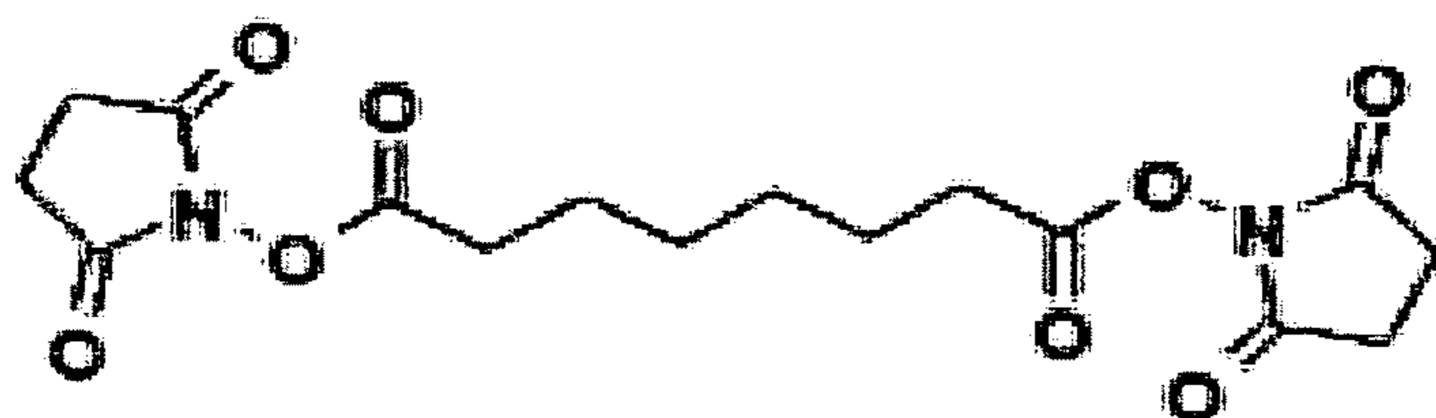
DSS (disuccinimidylsuberate)
