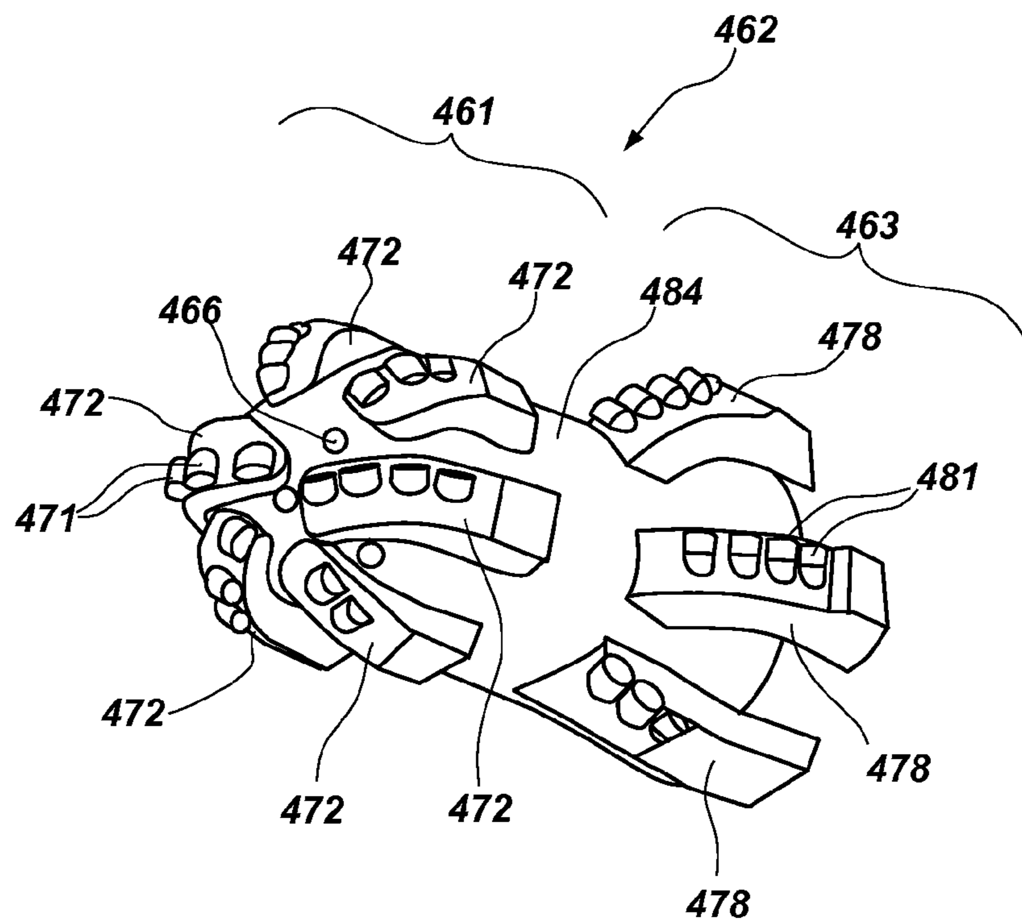
FIG. 13B
