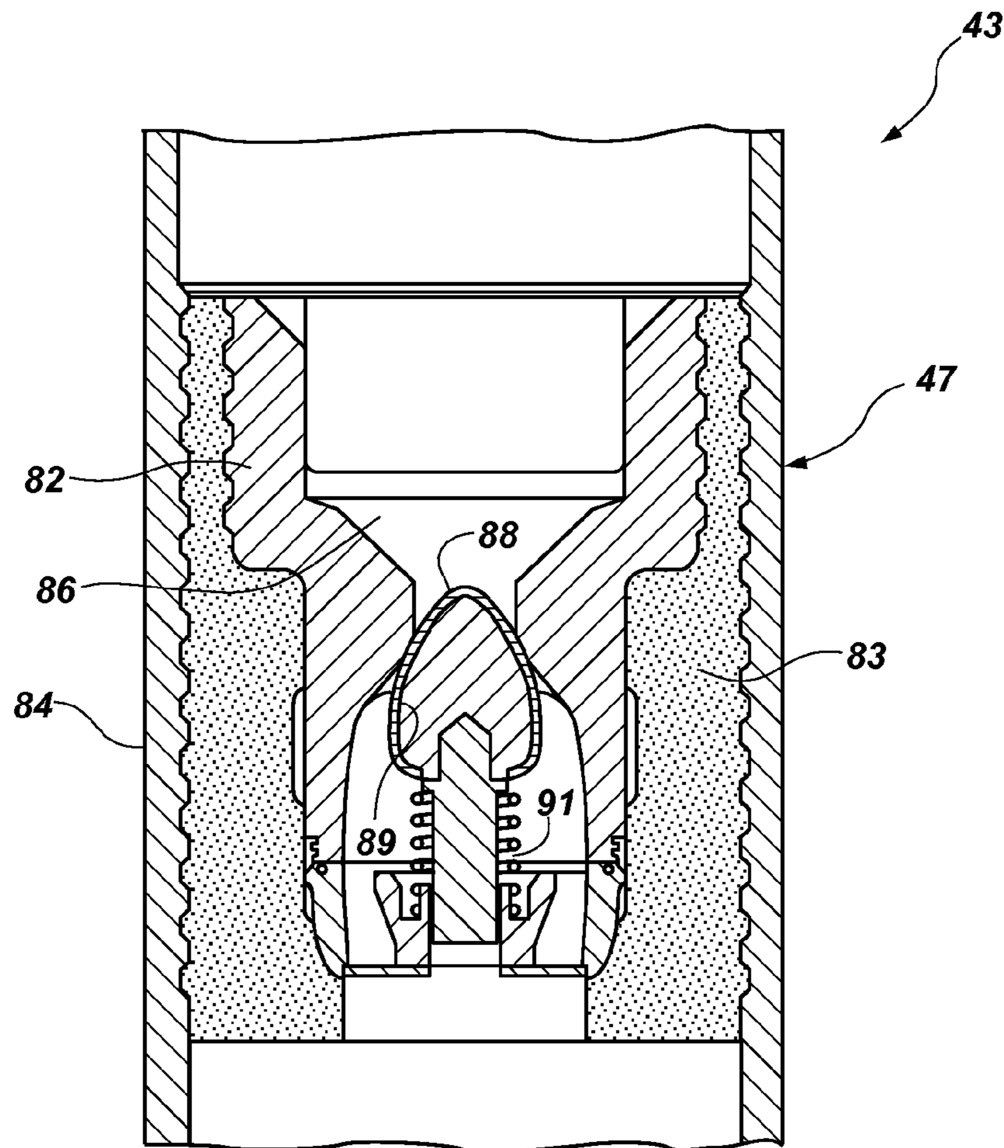
FIG. 1G
