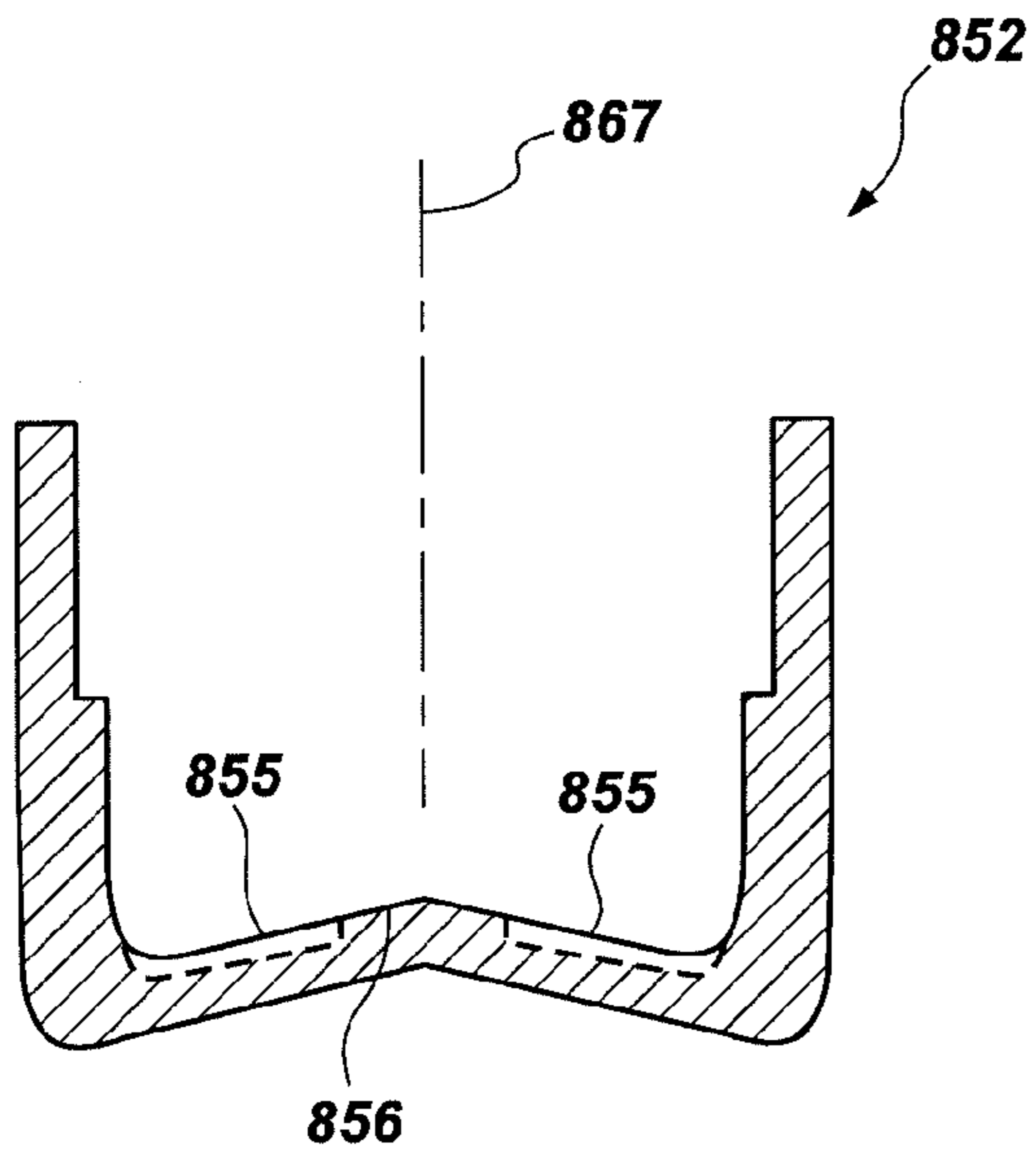
FIG. 21A
