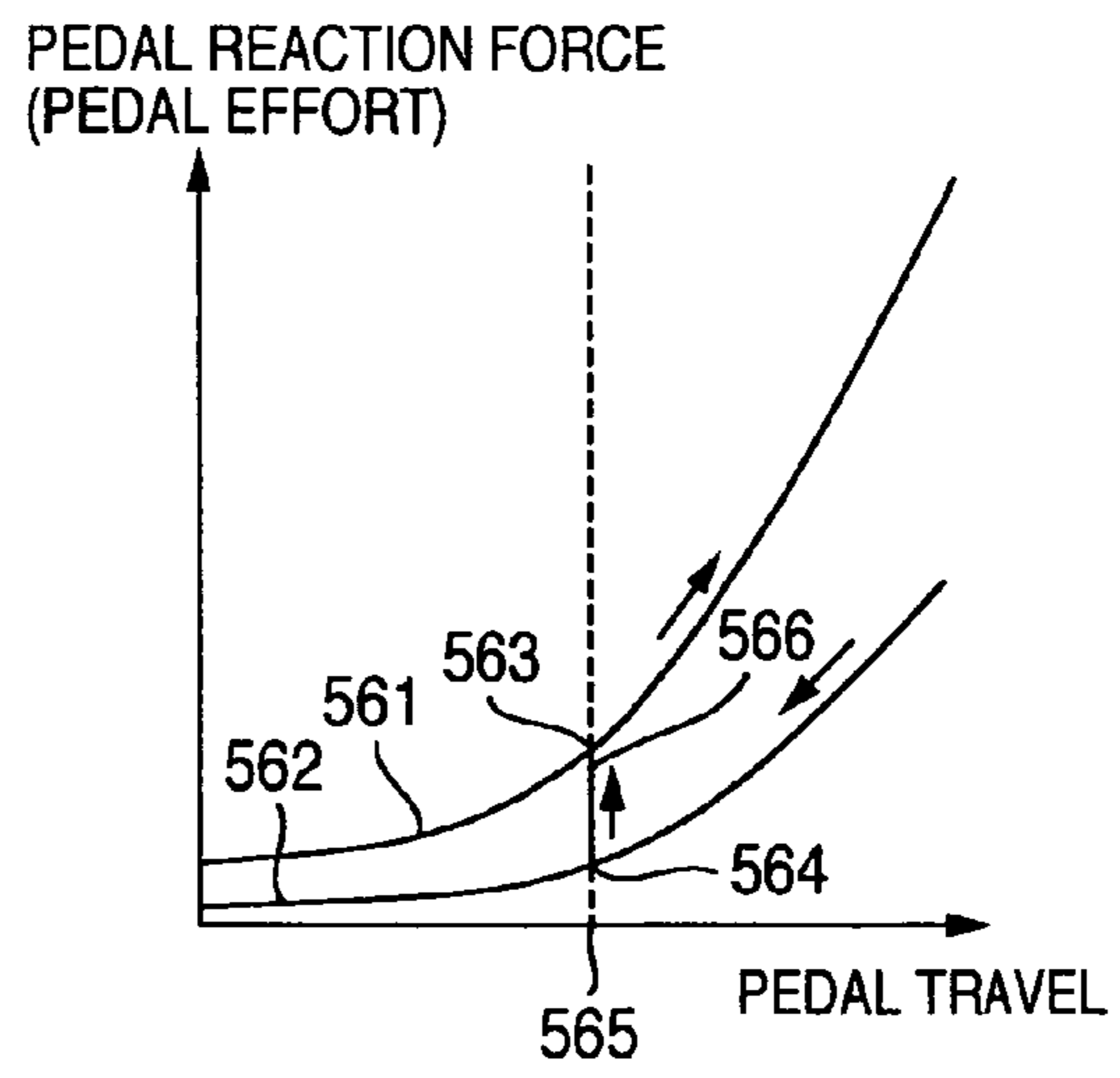
FIG.14b
