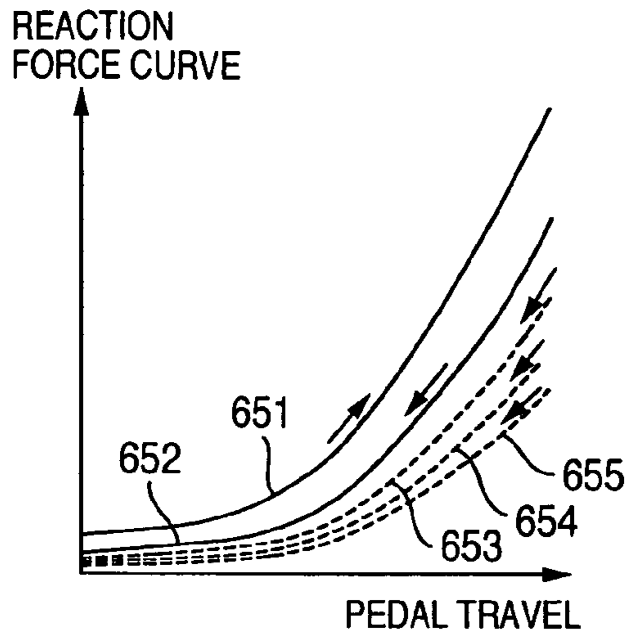
FIG.16a
