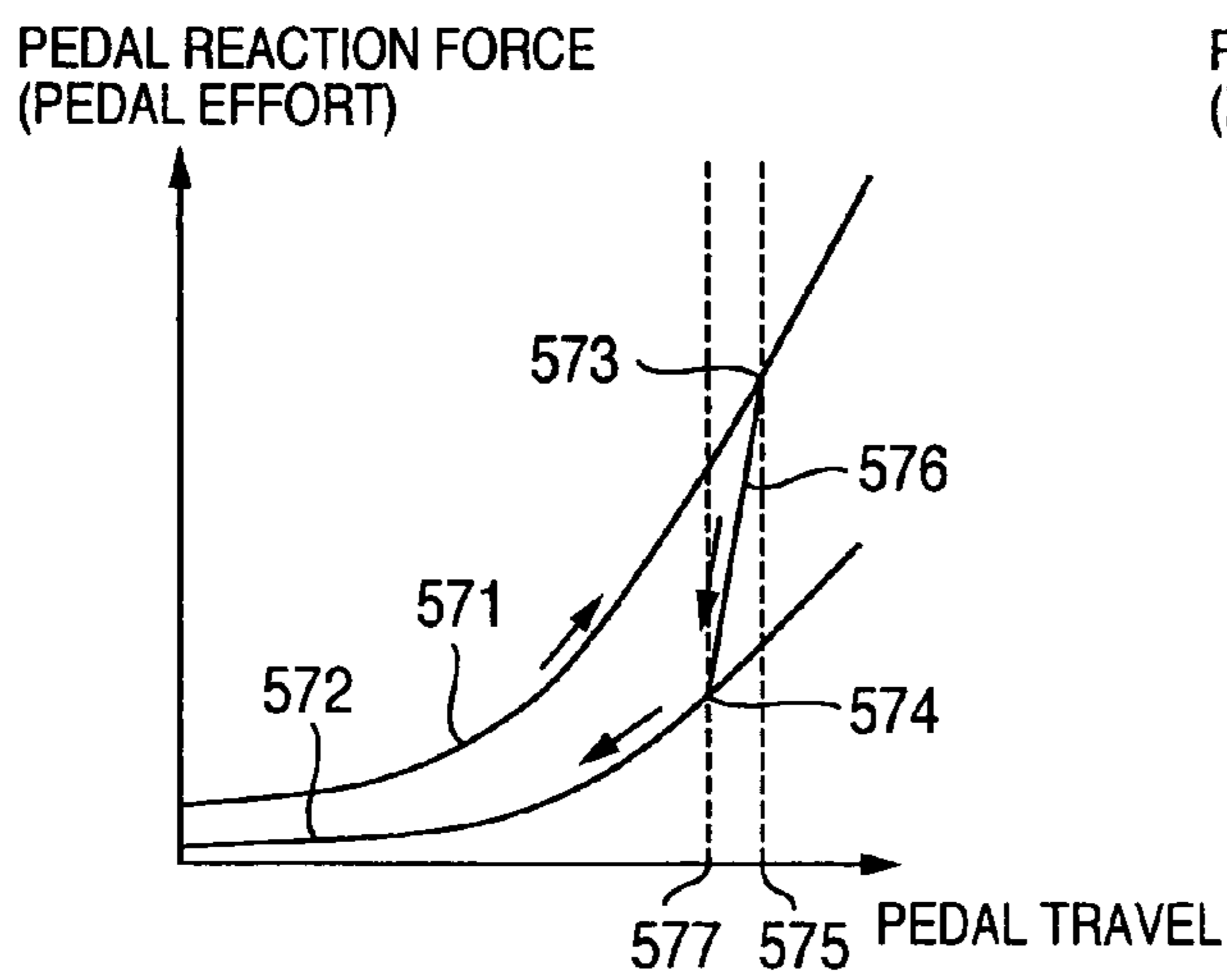
FIG.14c
