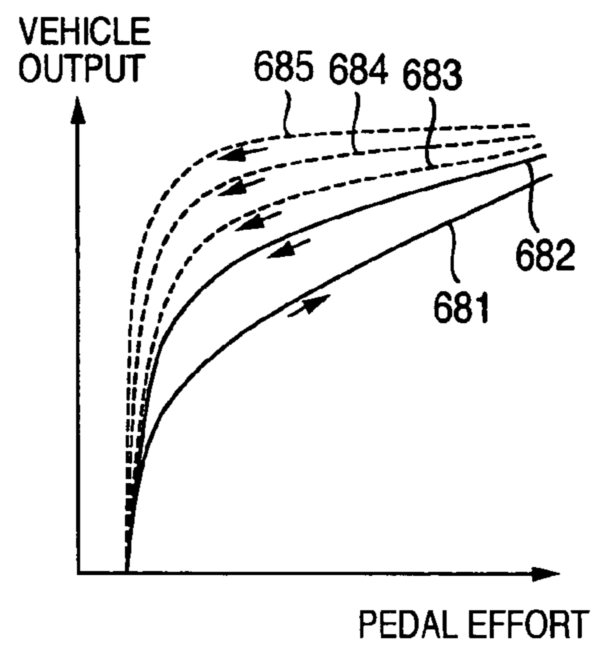
FIG.16d
