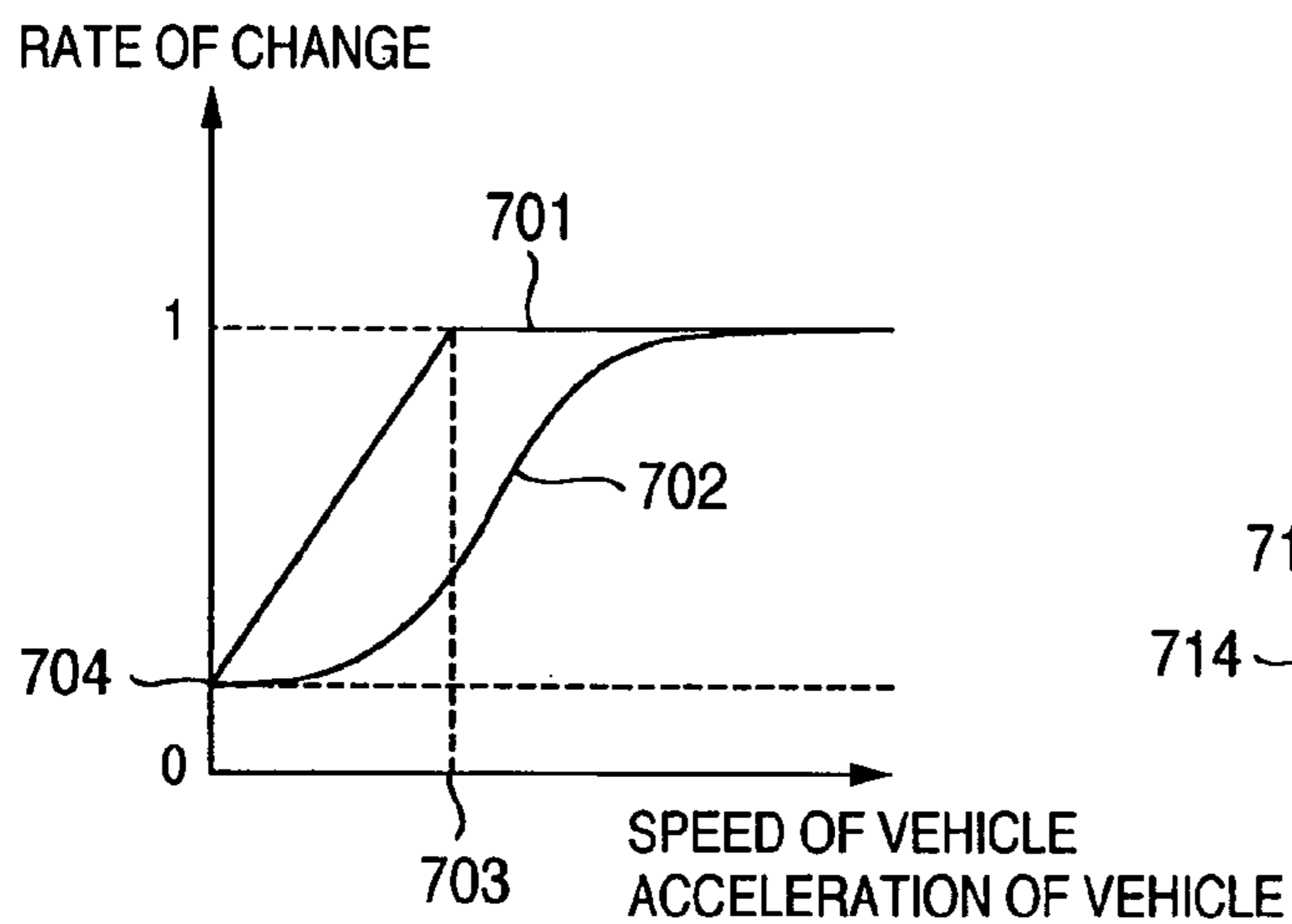
FIG.17a
