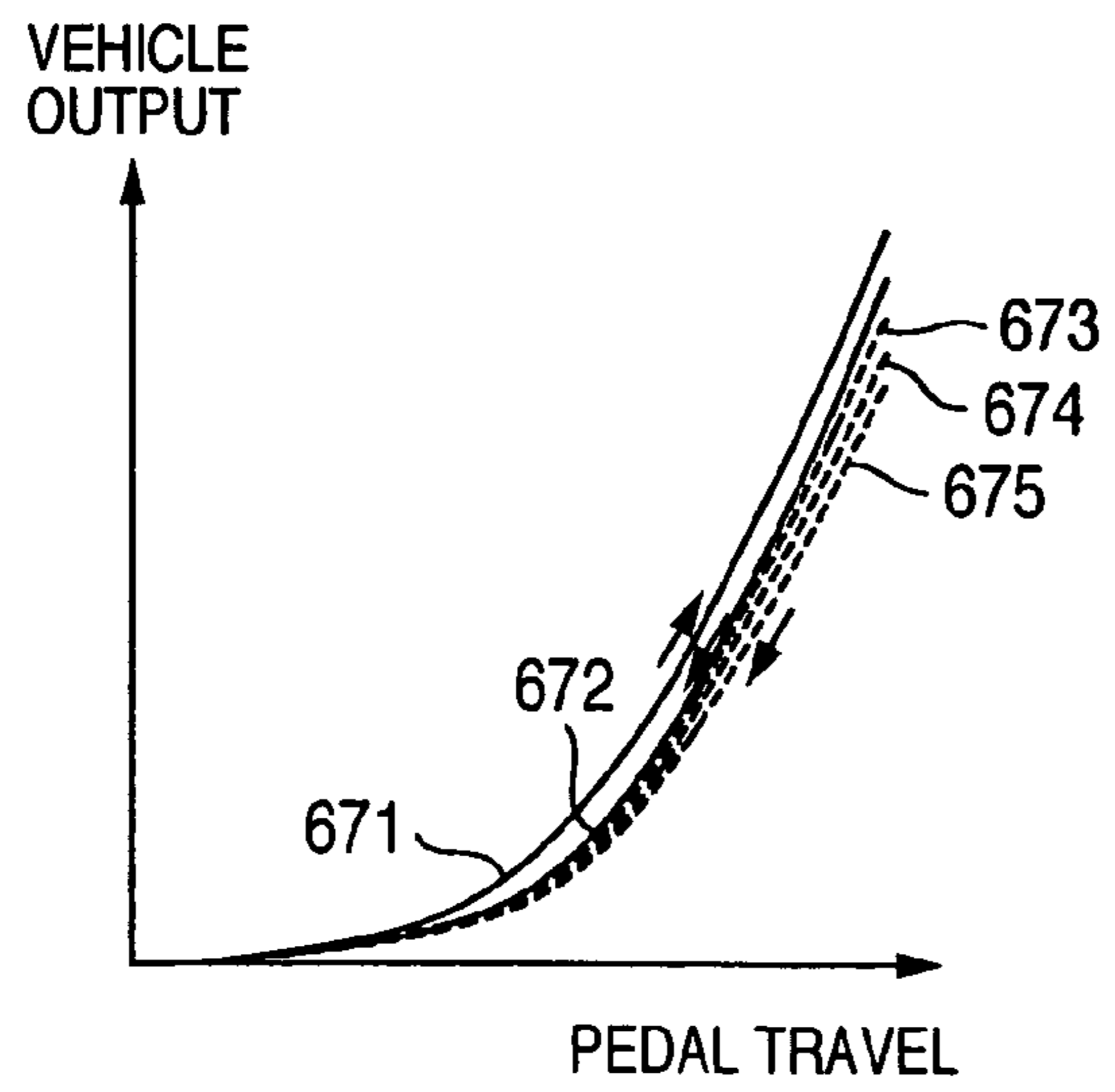
FIG.16c
