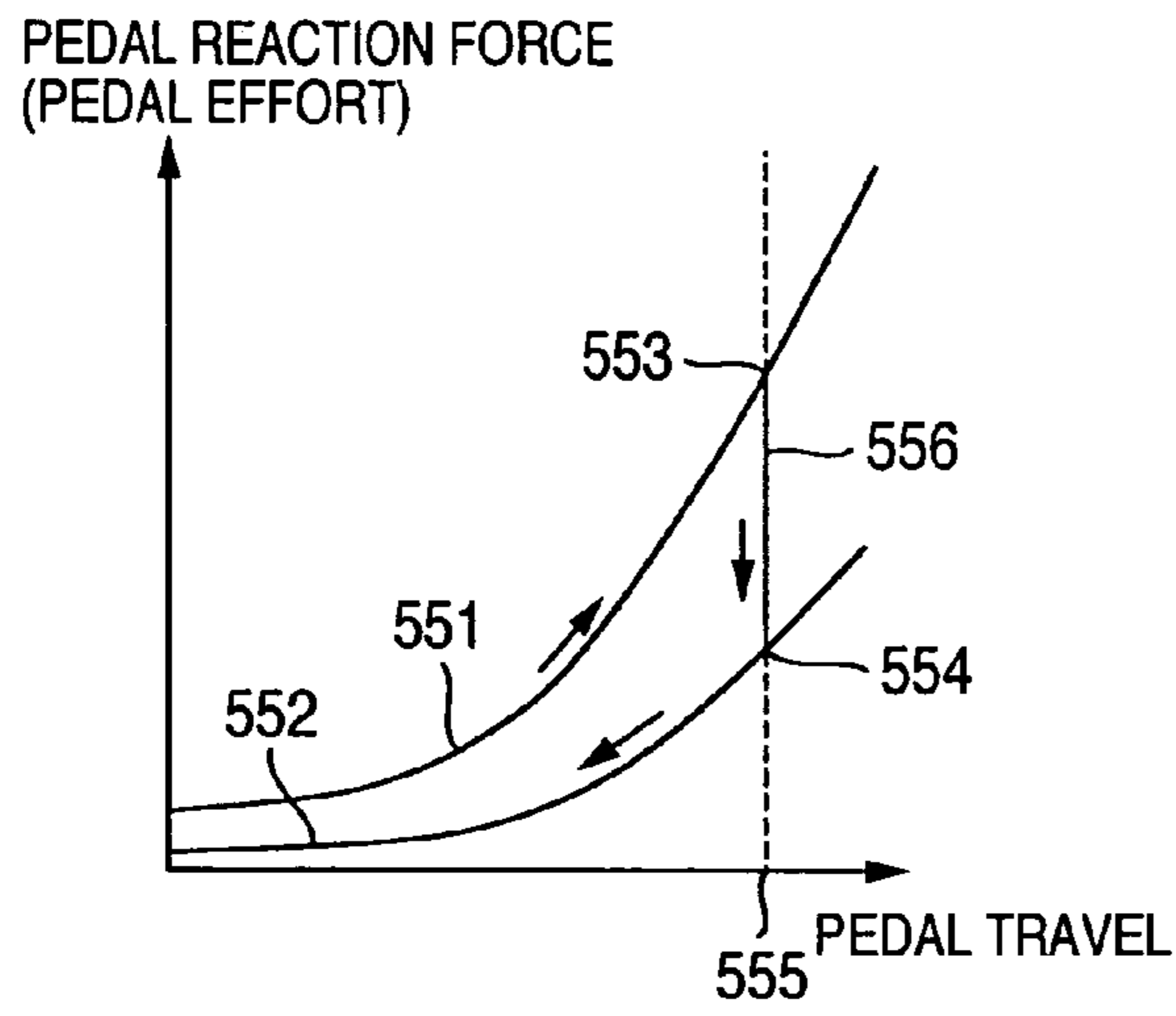
FIG.14a
