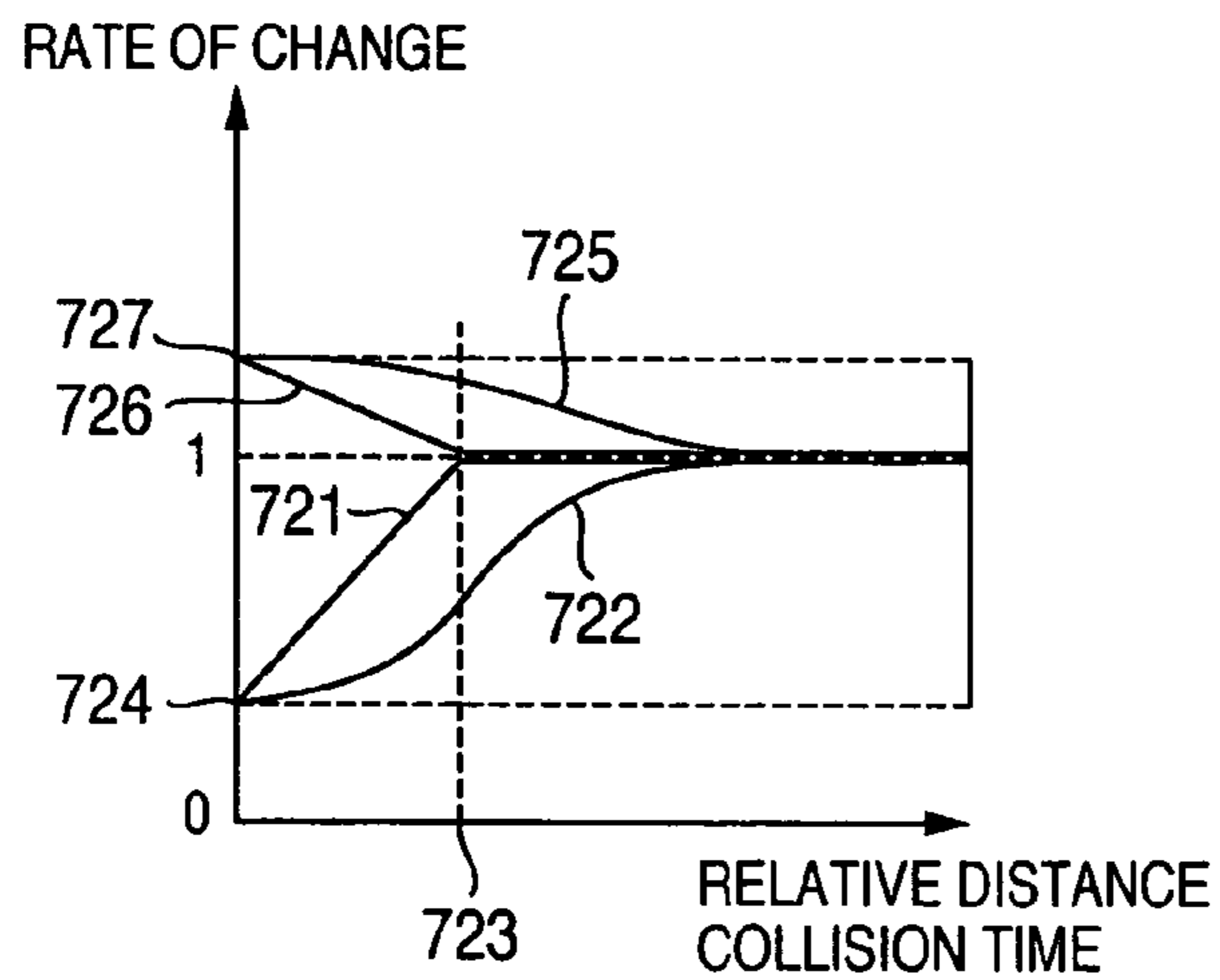
FIG.17c
