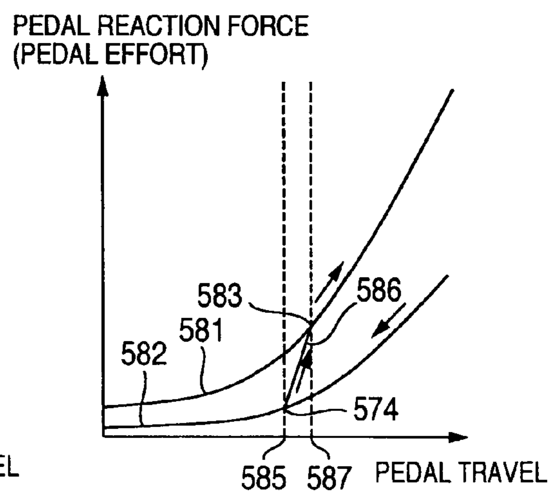
FIG.14d
