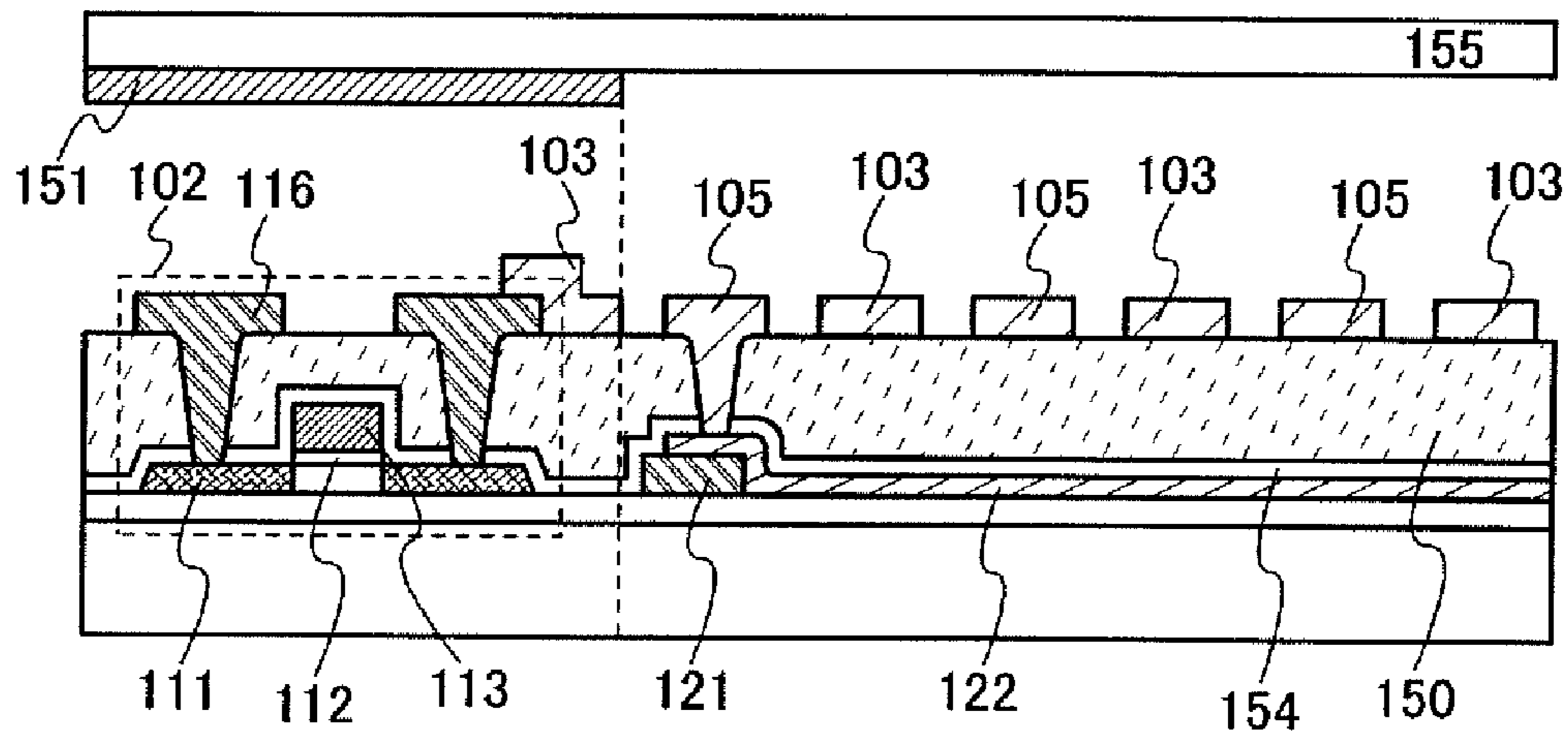
FIG. 10C
