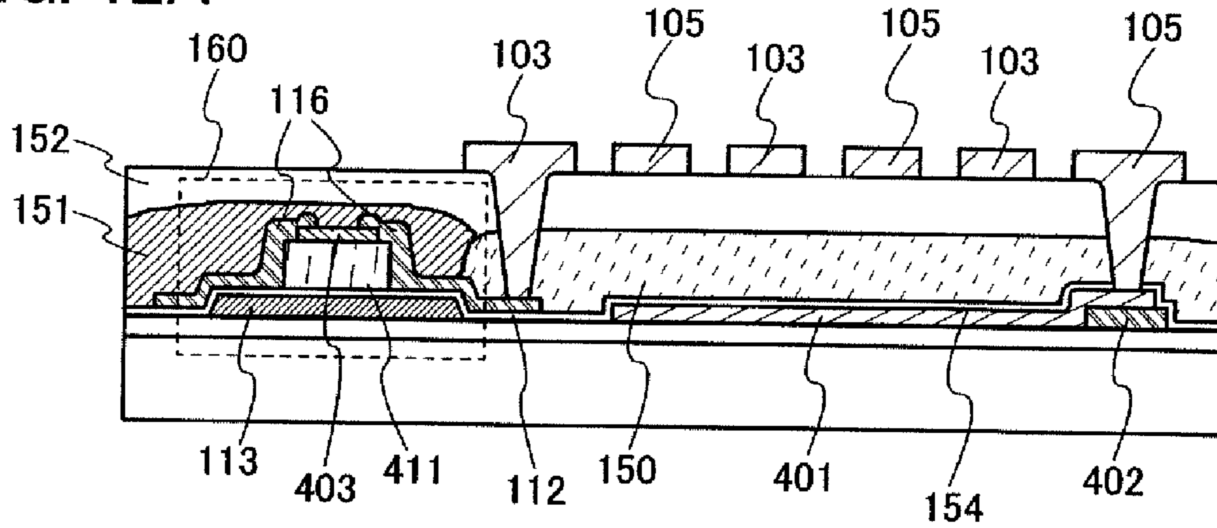
FIG. 12A
