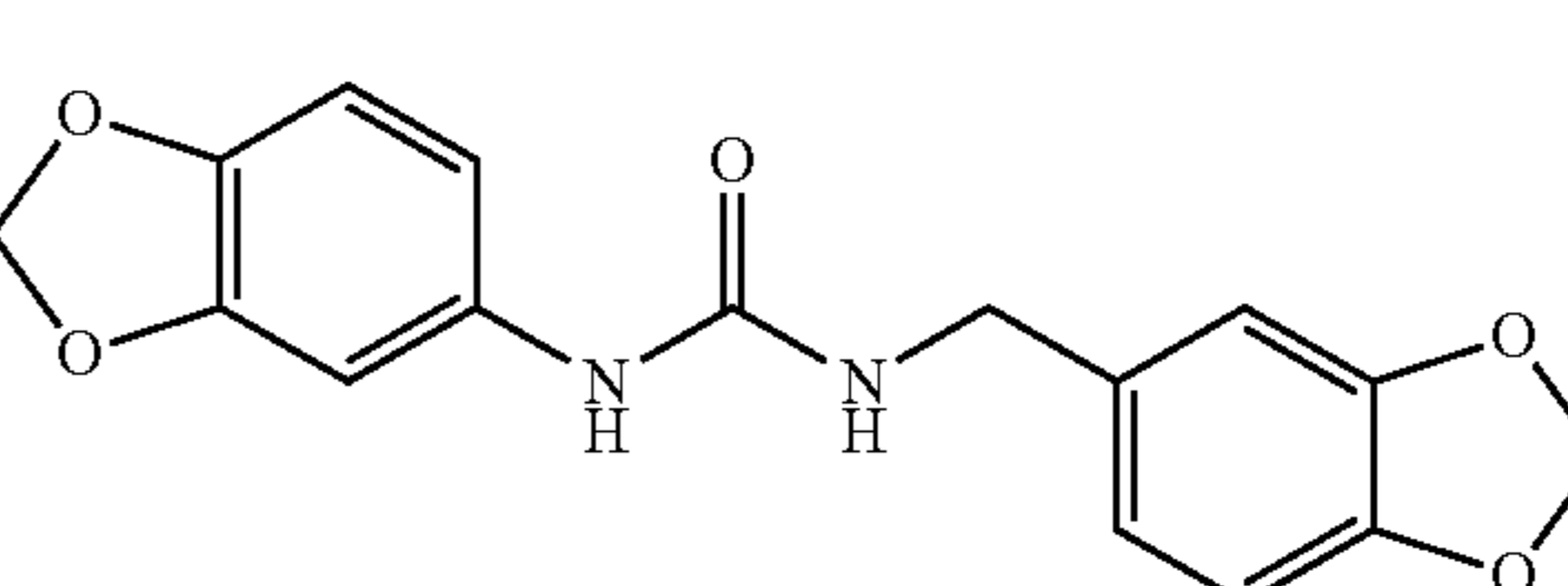
1-(3,4-methylenedioxyphenyl)-3-(3,4-methylenedioxybenzyl) urea
