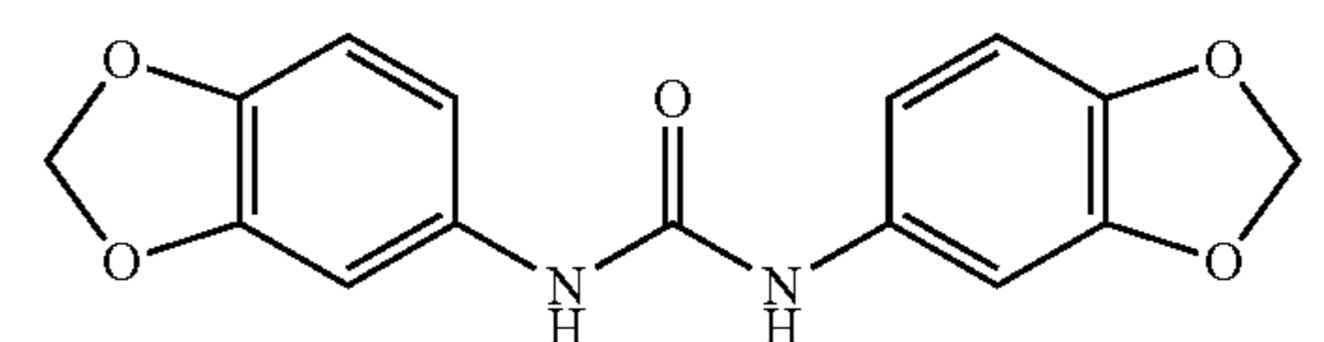
1,3-bis-(3,4-methylenedioxyphenyl)-urea
