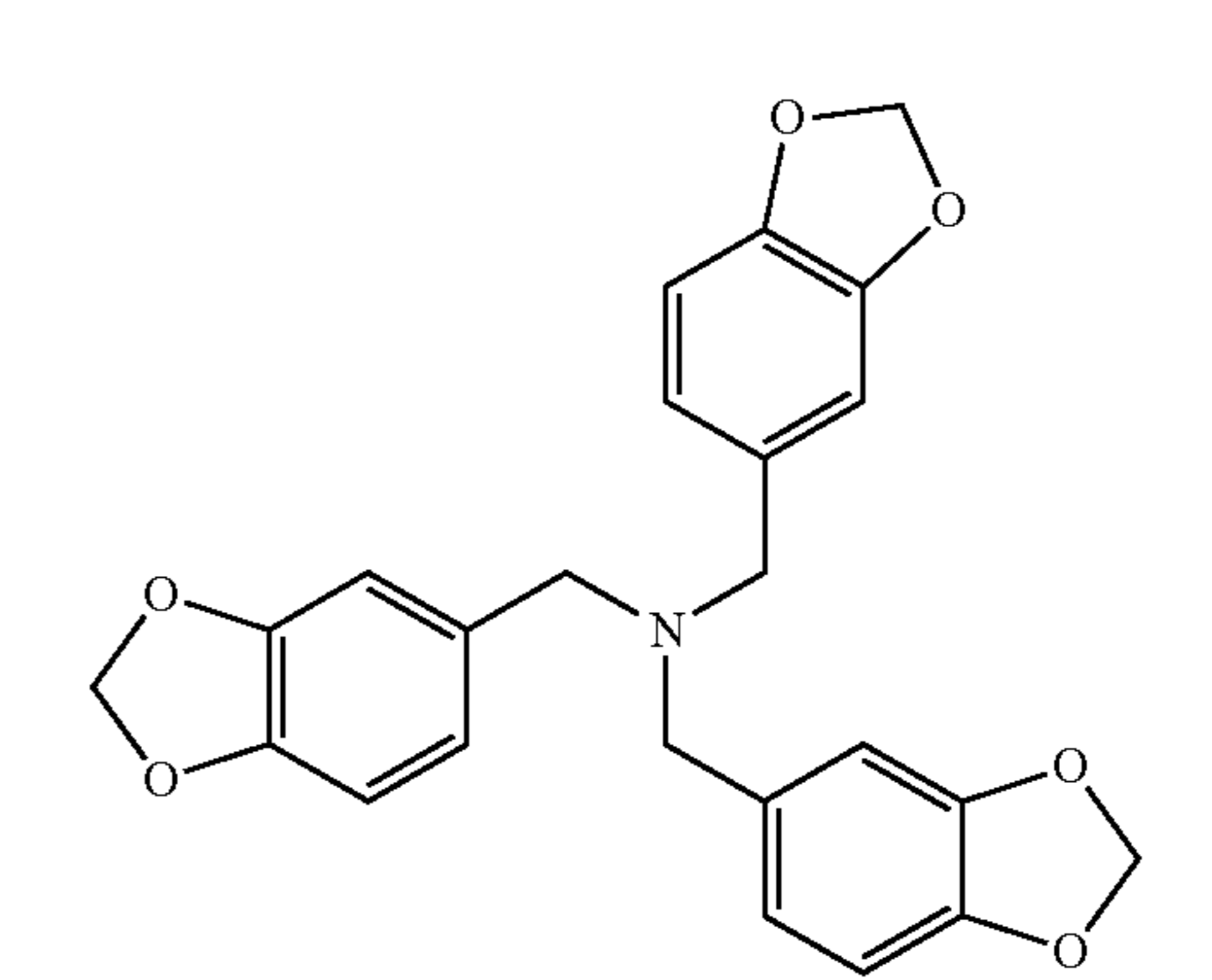
tris-(3,4-methylenedioxybenzyl)-amine
