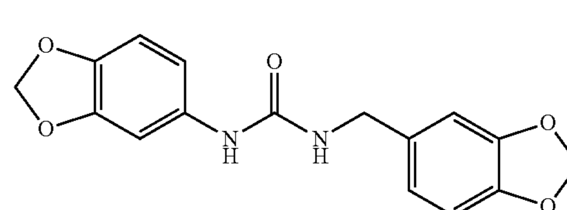
1-(3,4-methylenedioxyphenyl)-3-(3,4-methylenedioxybenzyl) urea
