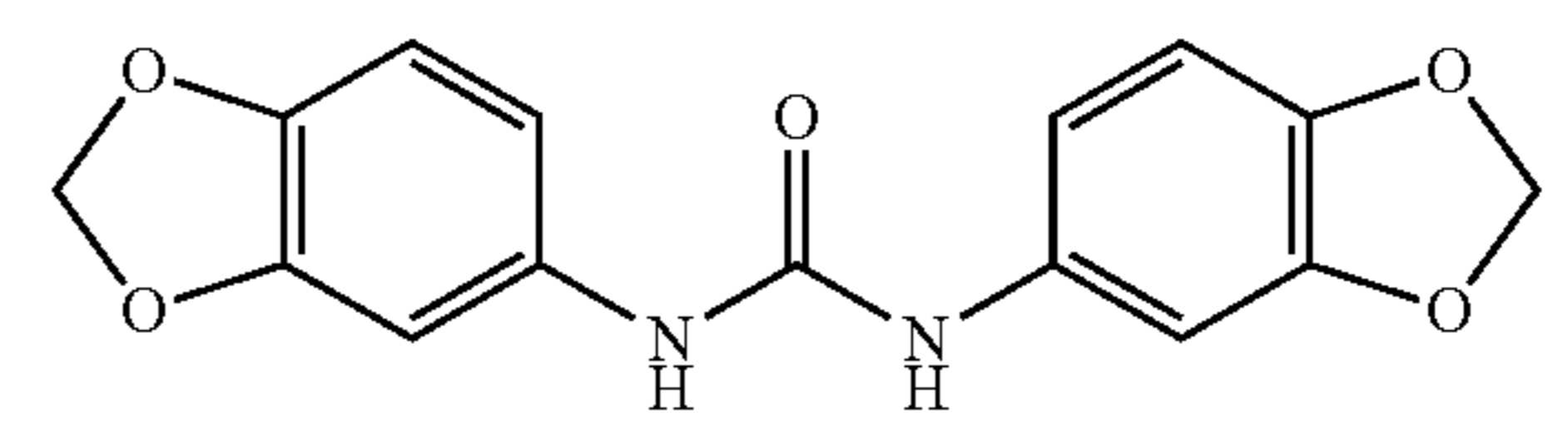
1,3-bis-(3,4-methylenedioxyphenyl)-urea
