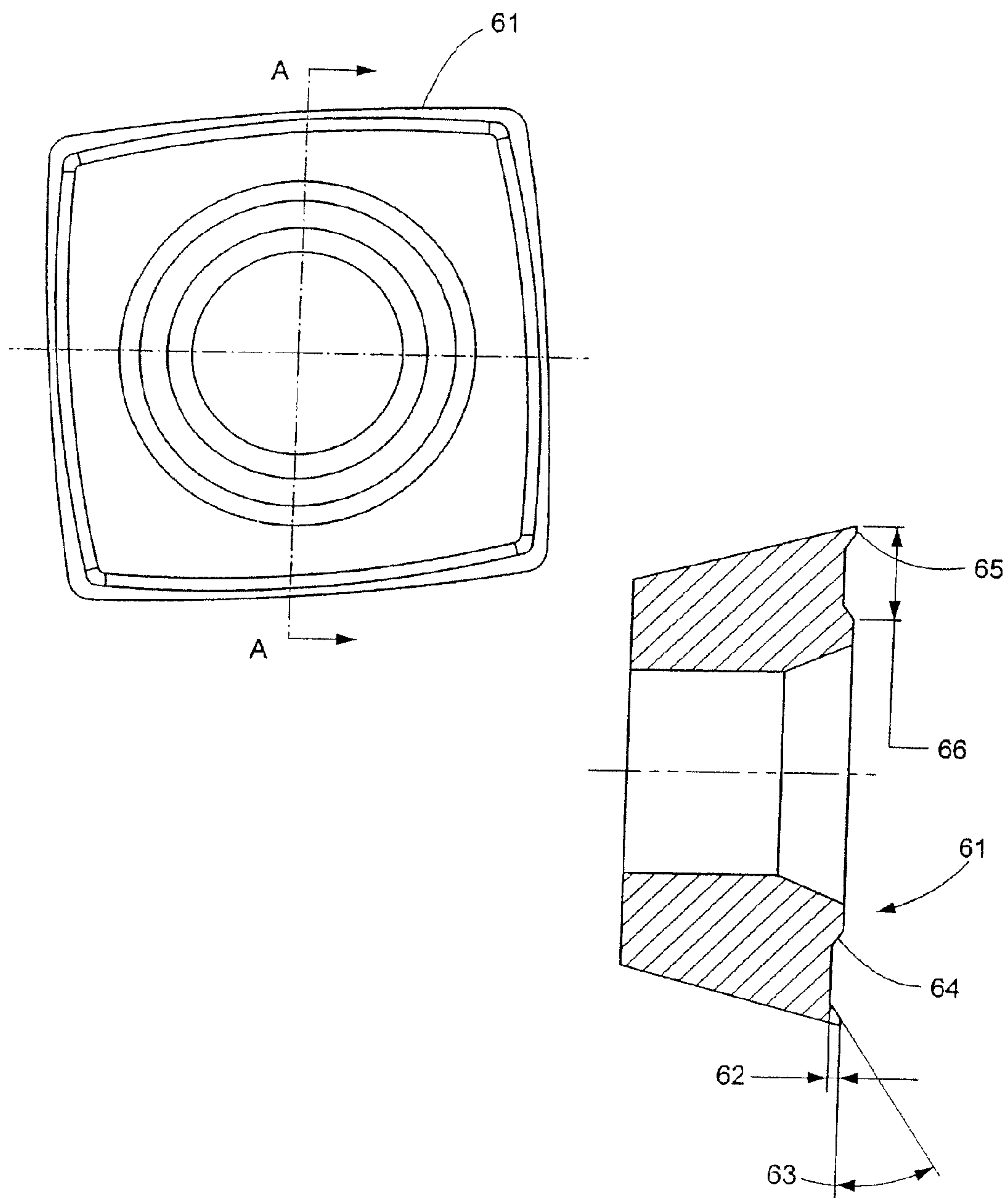
SECTION A-A
