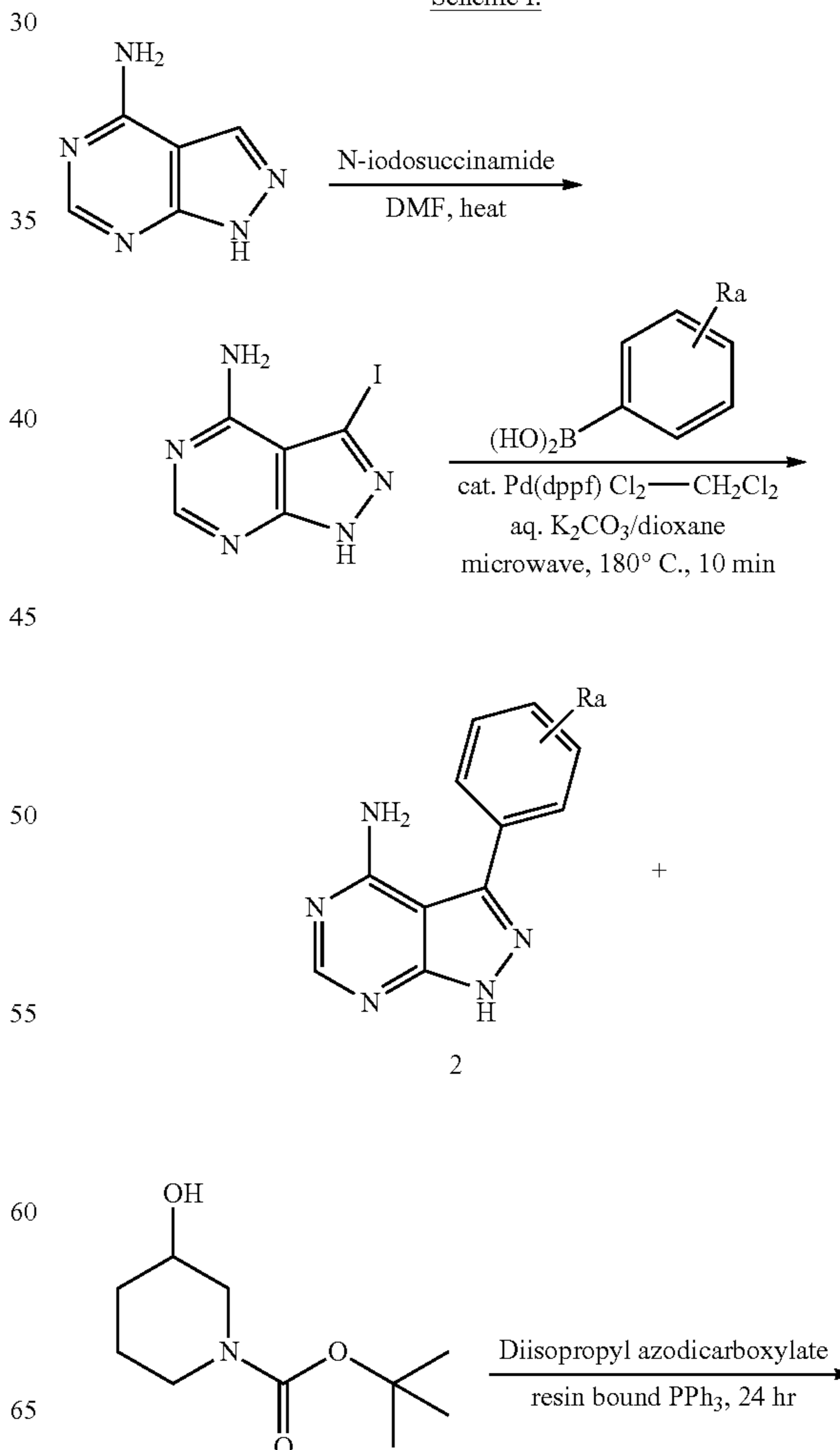
Scheme I.
