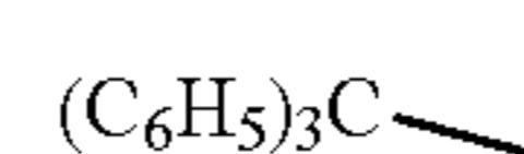
trityl
