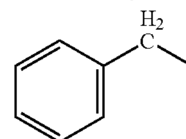
Bn
