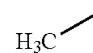
Me
