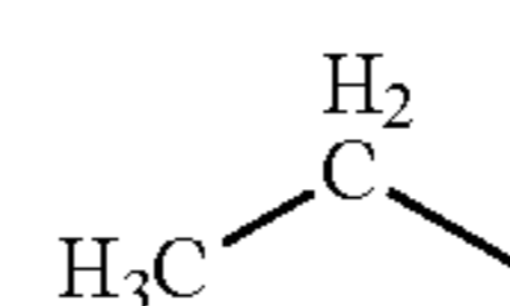
Et
