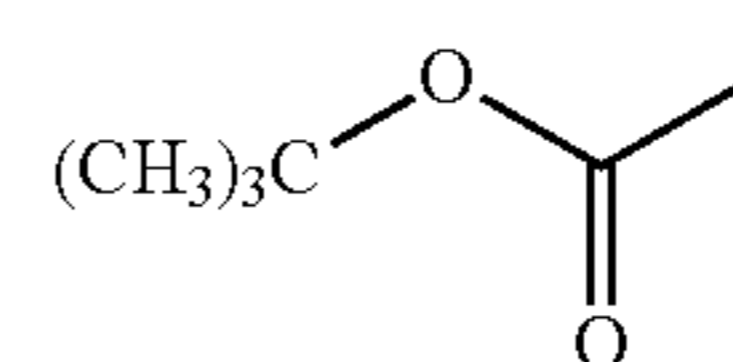
Boc
