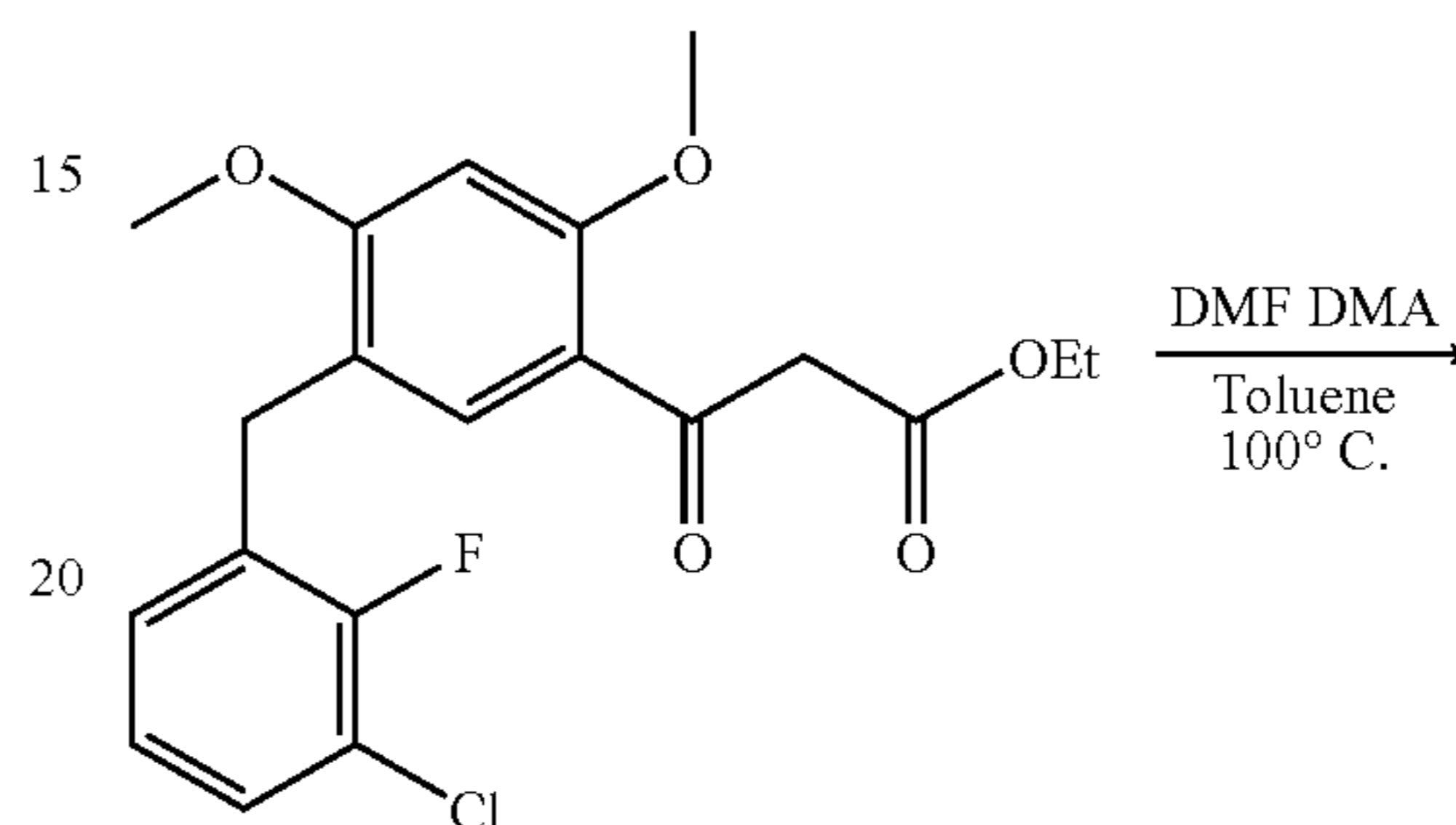
Compound 6a C 20 H 20 ClFO 5 Mol. Wt.: 394.82
