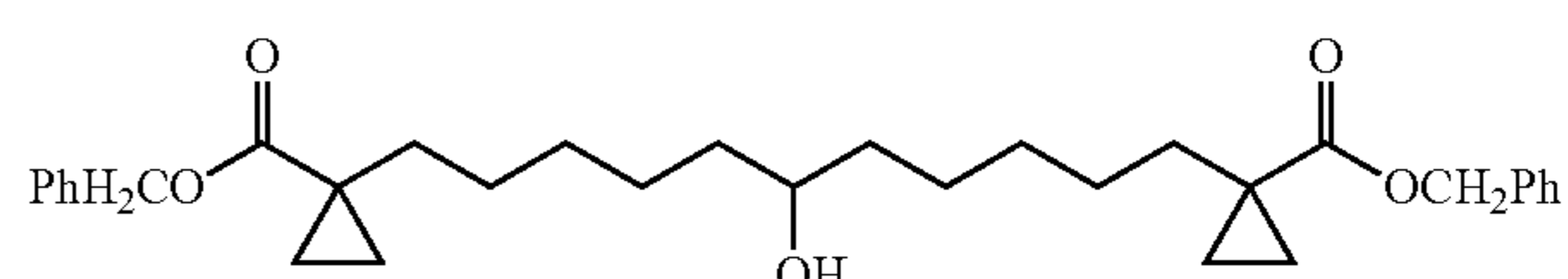
1,11-Bis-(1-benzyloxycarbonyl-cyclopropyl)-undecan-6-ol
