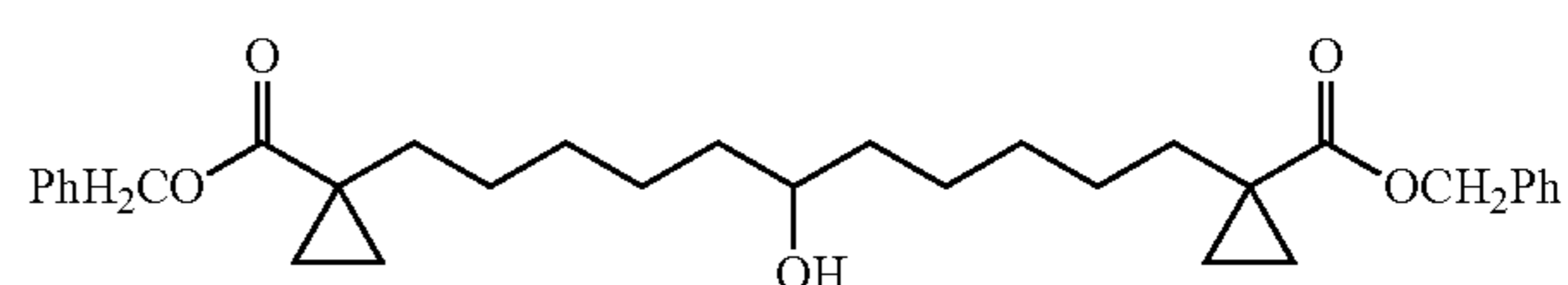
1,11-Bis-(1-benzyloxycarbonyl-cyclopropyl)-undecan-6-ol
