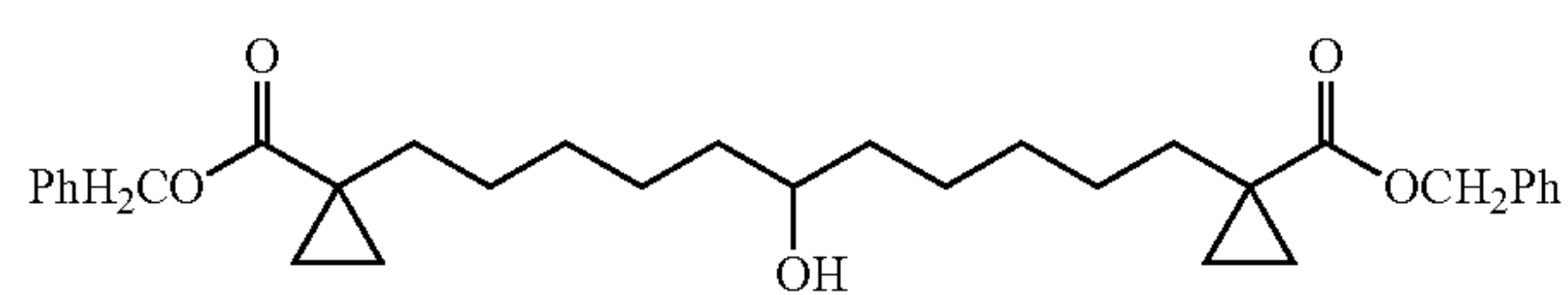
1,11-Bis-(1-benzyloxycarbonyl-cyclopropyl)-undecan-6-ol
