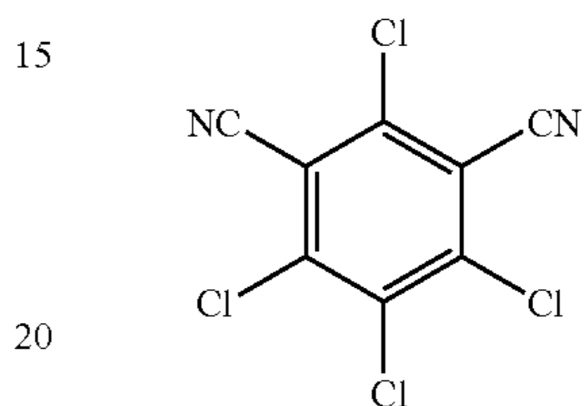
(CHLOROTHALONIL)
