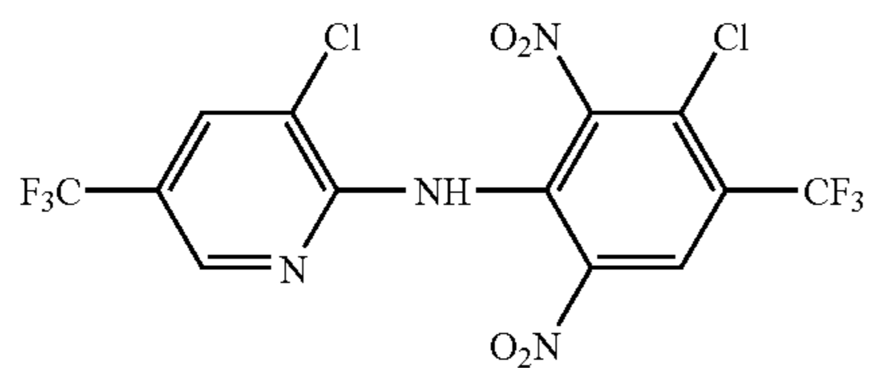
(FLUAZINAM)
