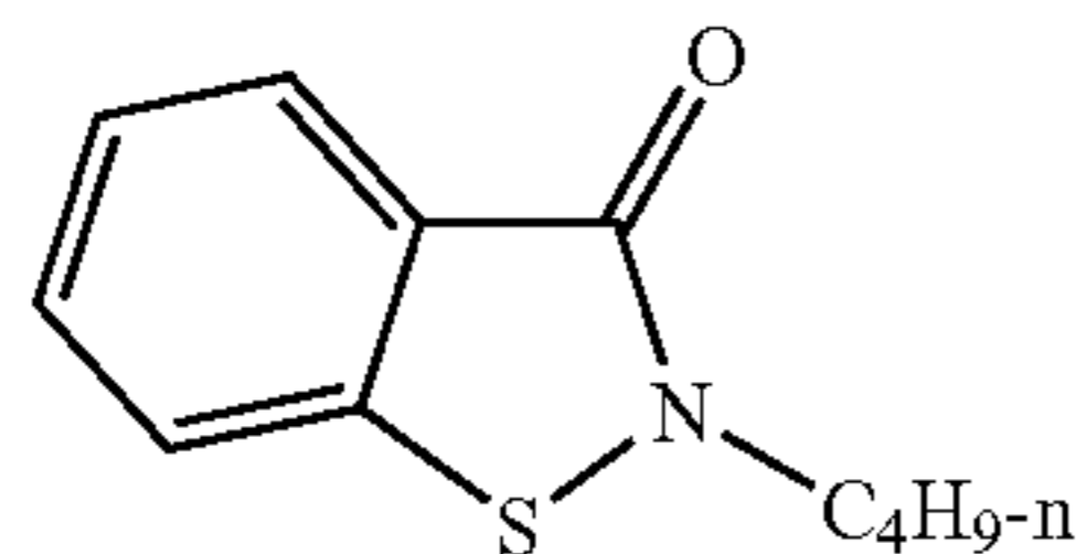
butylbenzothiazolinone
