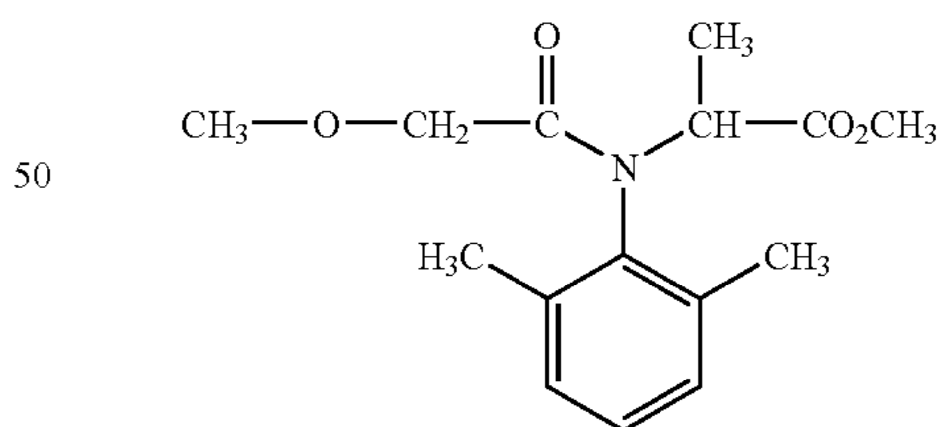
(METALAXYL)
