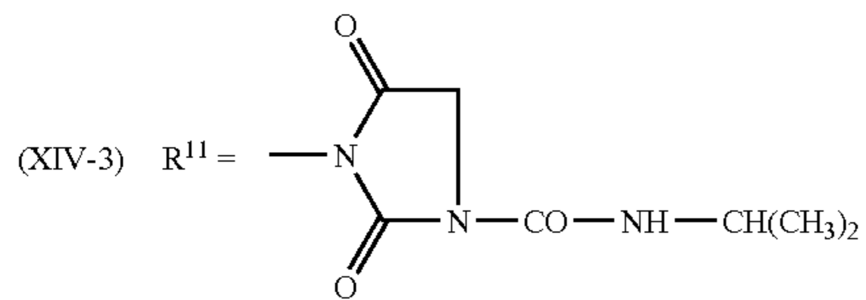
(IPRODIONE)
