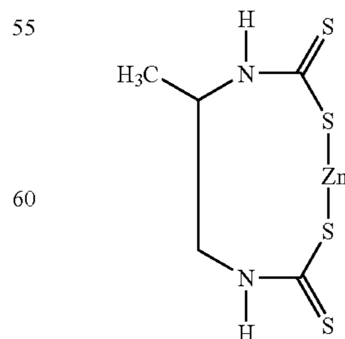
(ANTRACOL)
