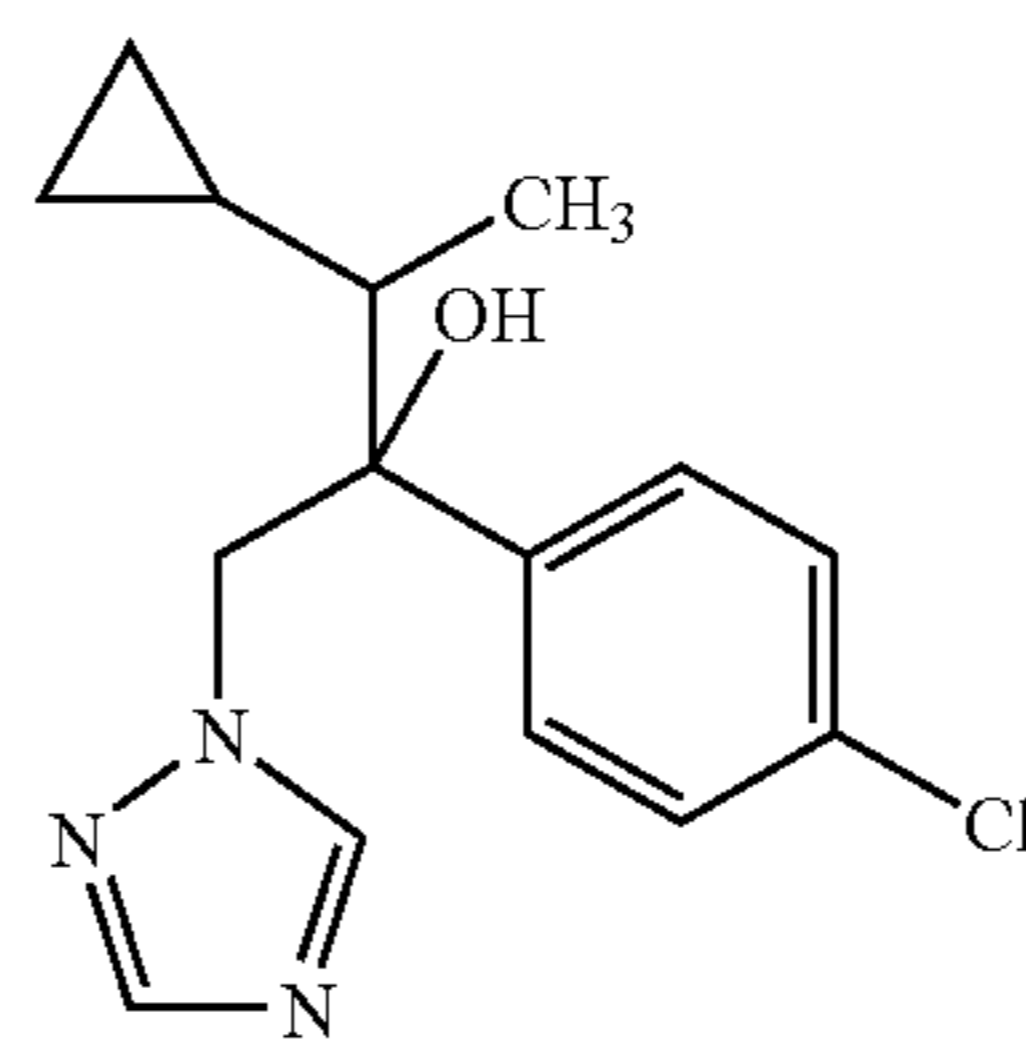
cyproconazole
