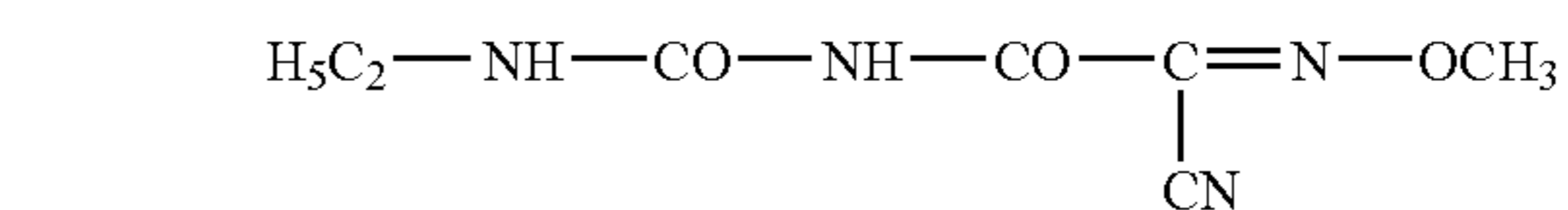
(CYMOXANIL)
