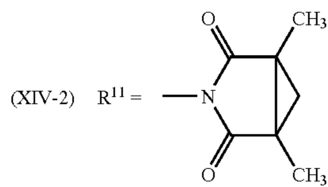
(PROCYMIDONE)
