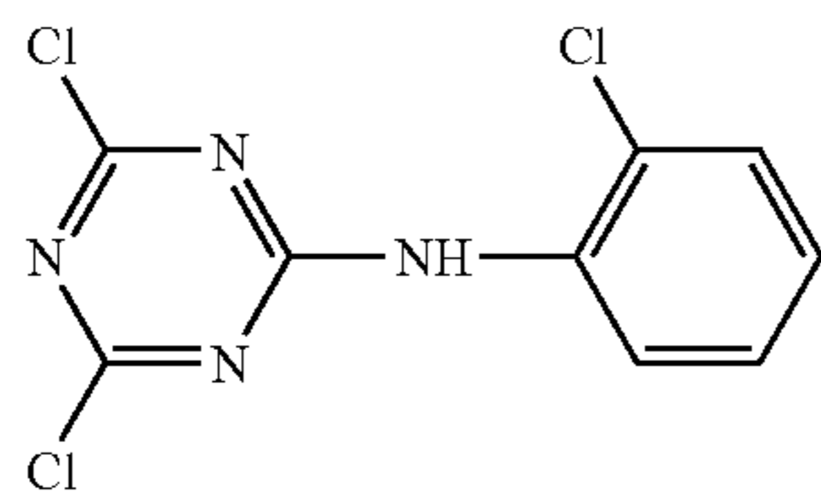
(ANILAZIN)
