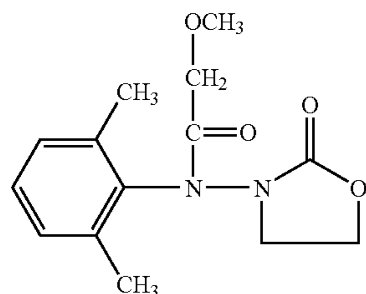
(OXADIXYL)
