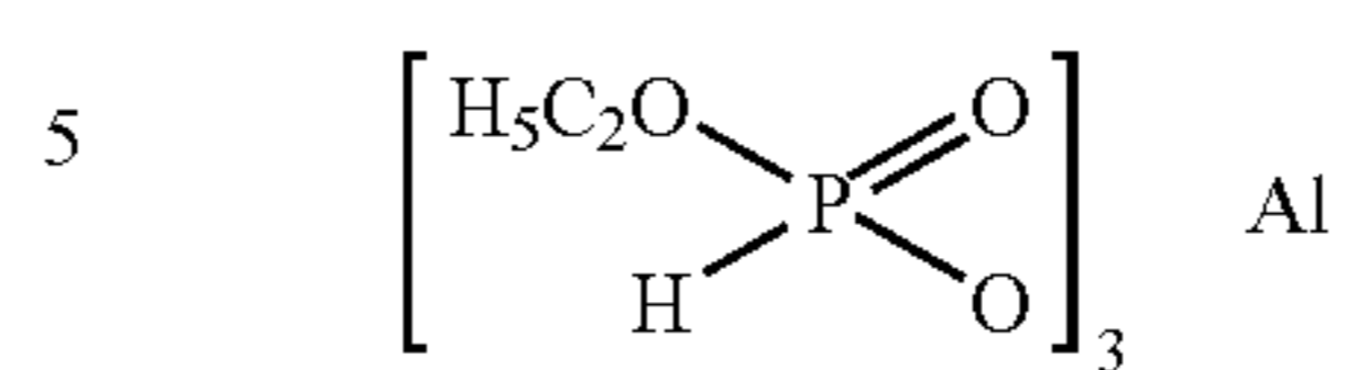
(FOSETYL AL)
