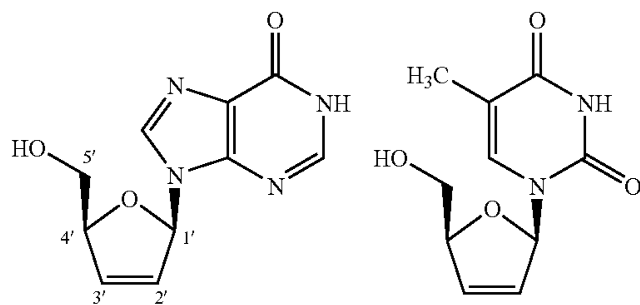
Stavudine
