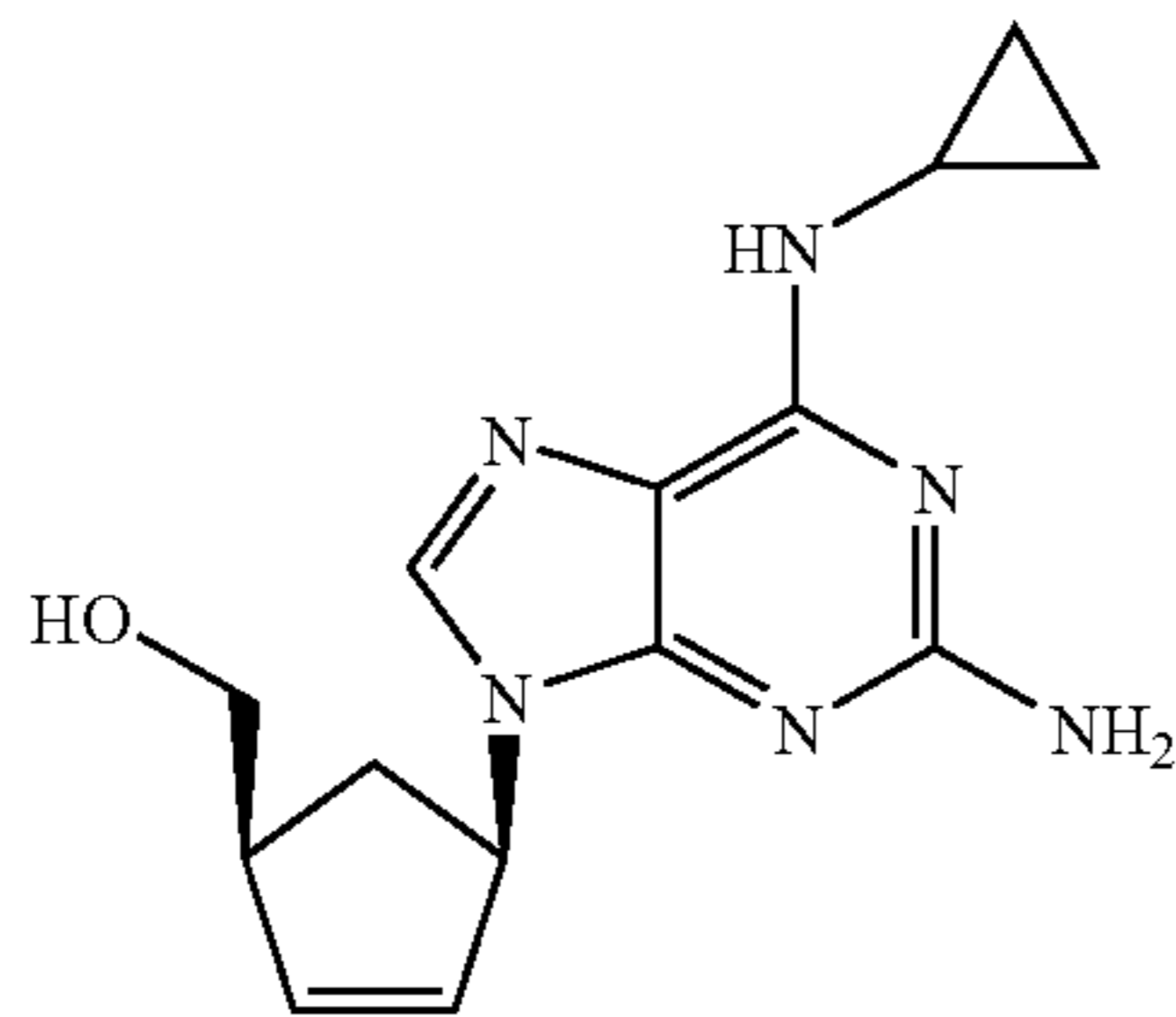
Abacavir
