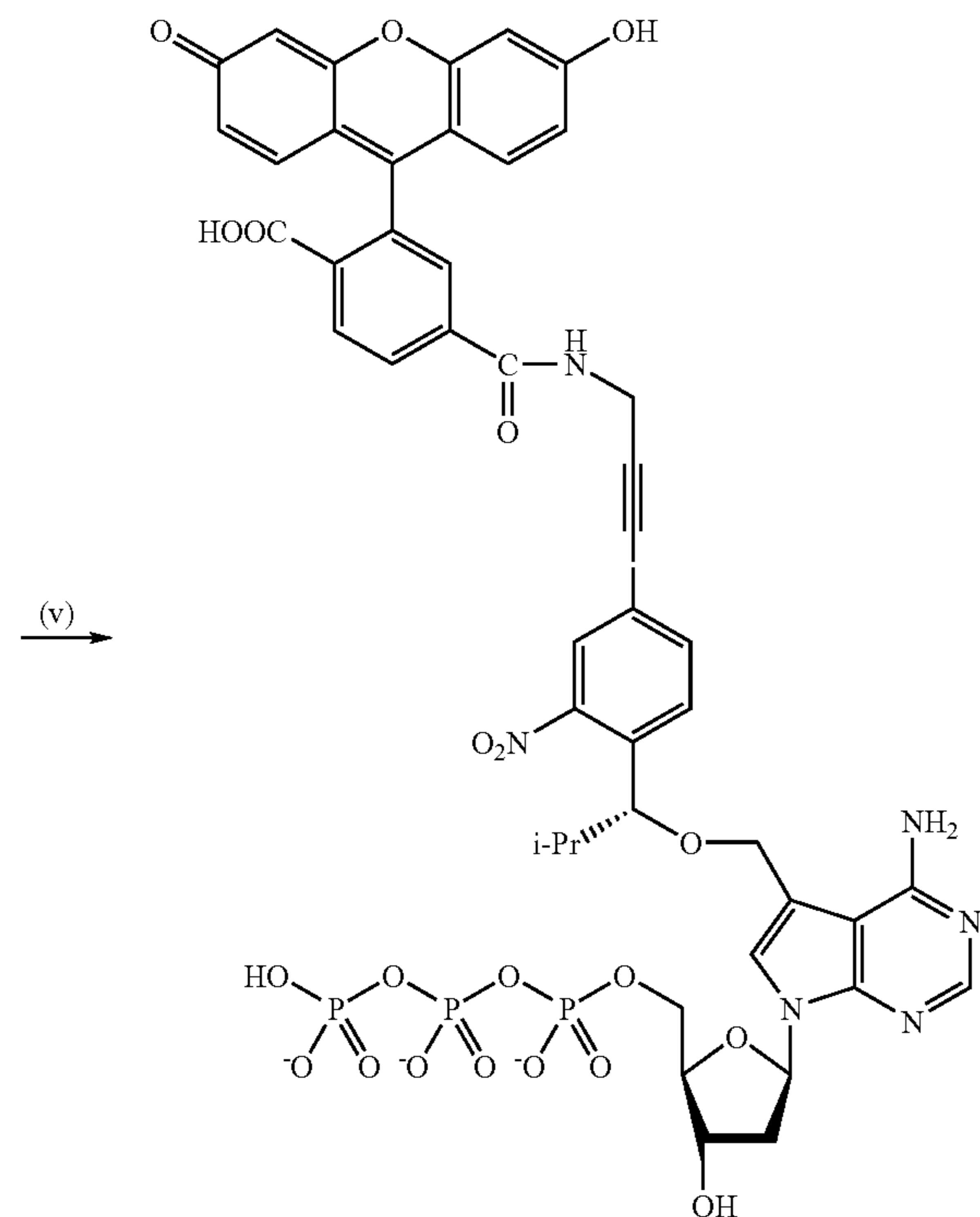
Scheme 27.
