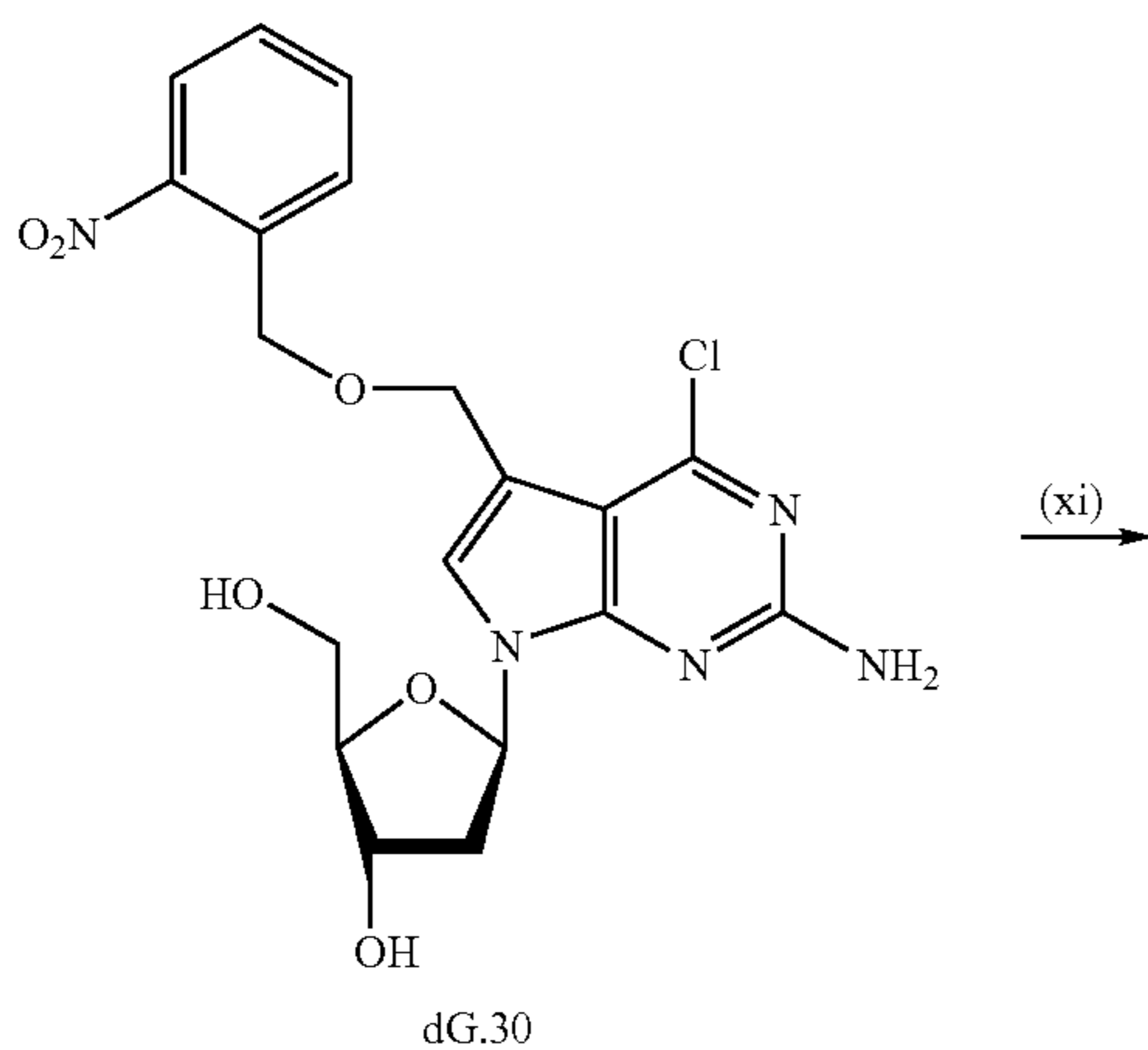
Scheme 20.
