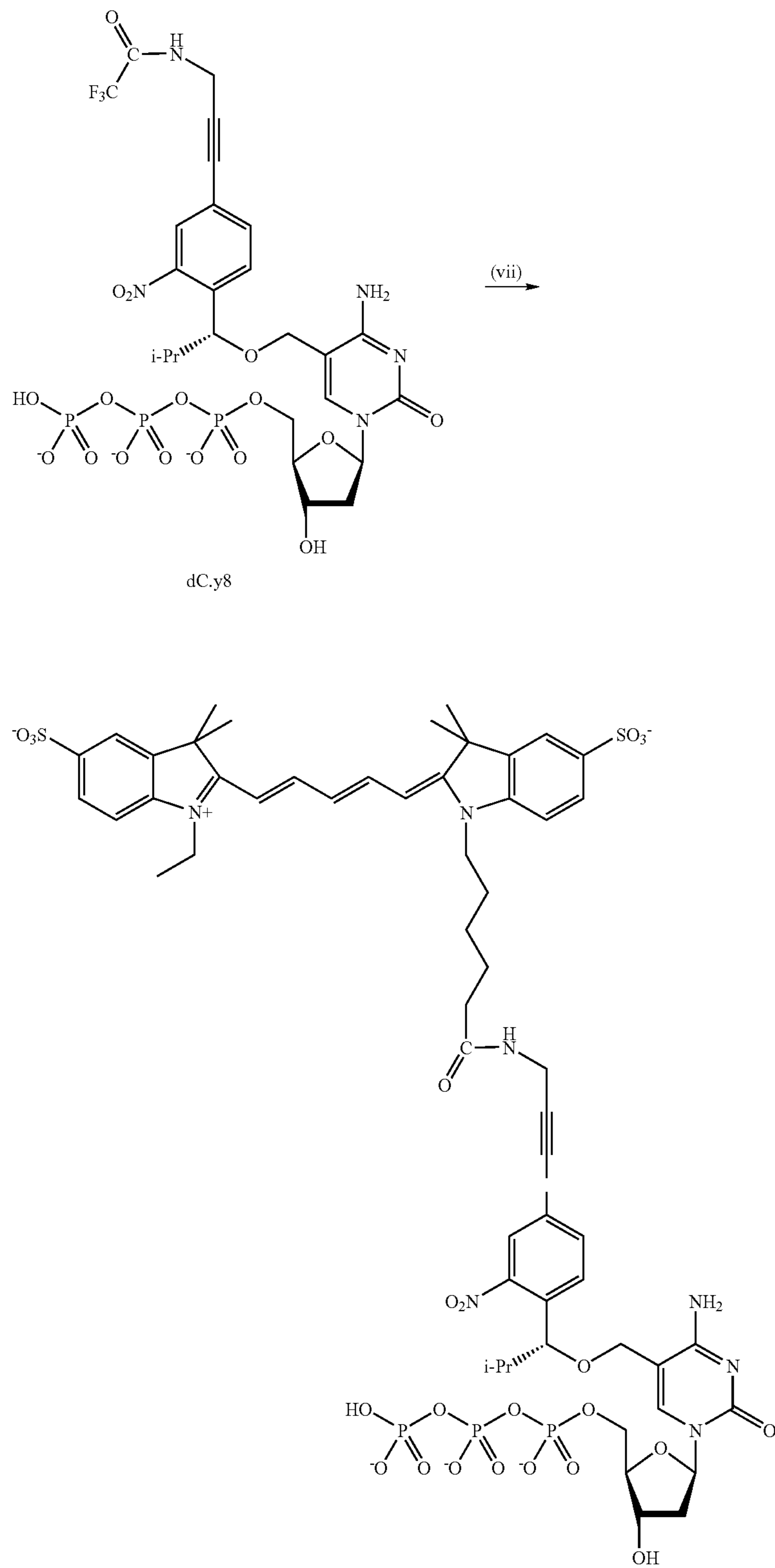
Scheme 16.
