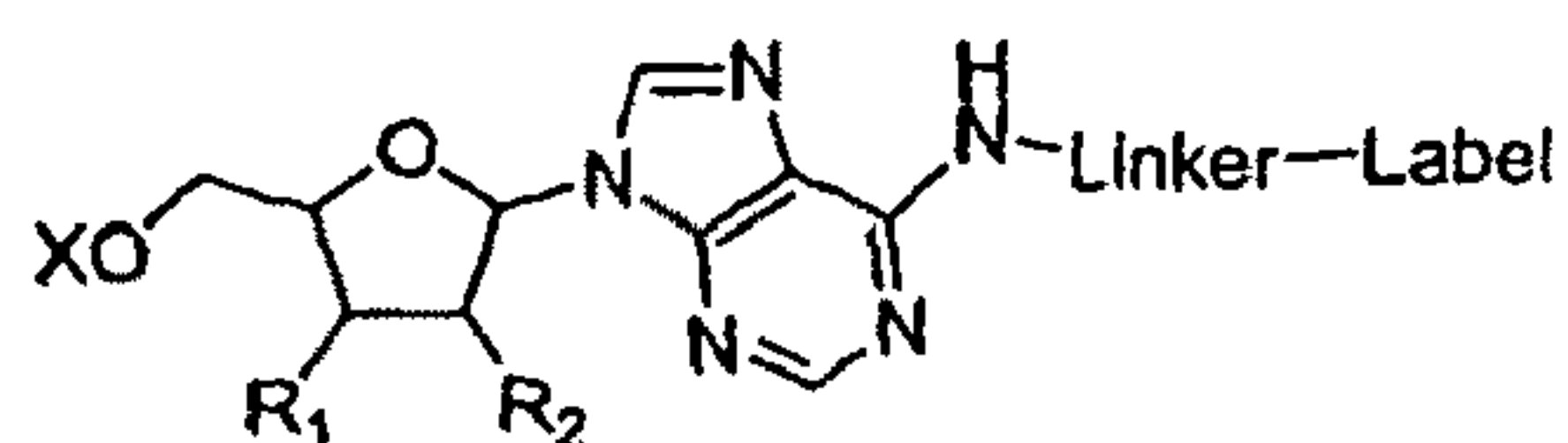
Adenosine N6-linker
