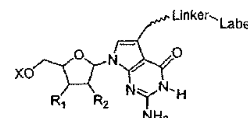
N7 Deazaguanosine C7-linker
