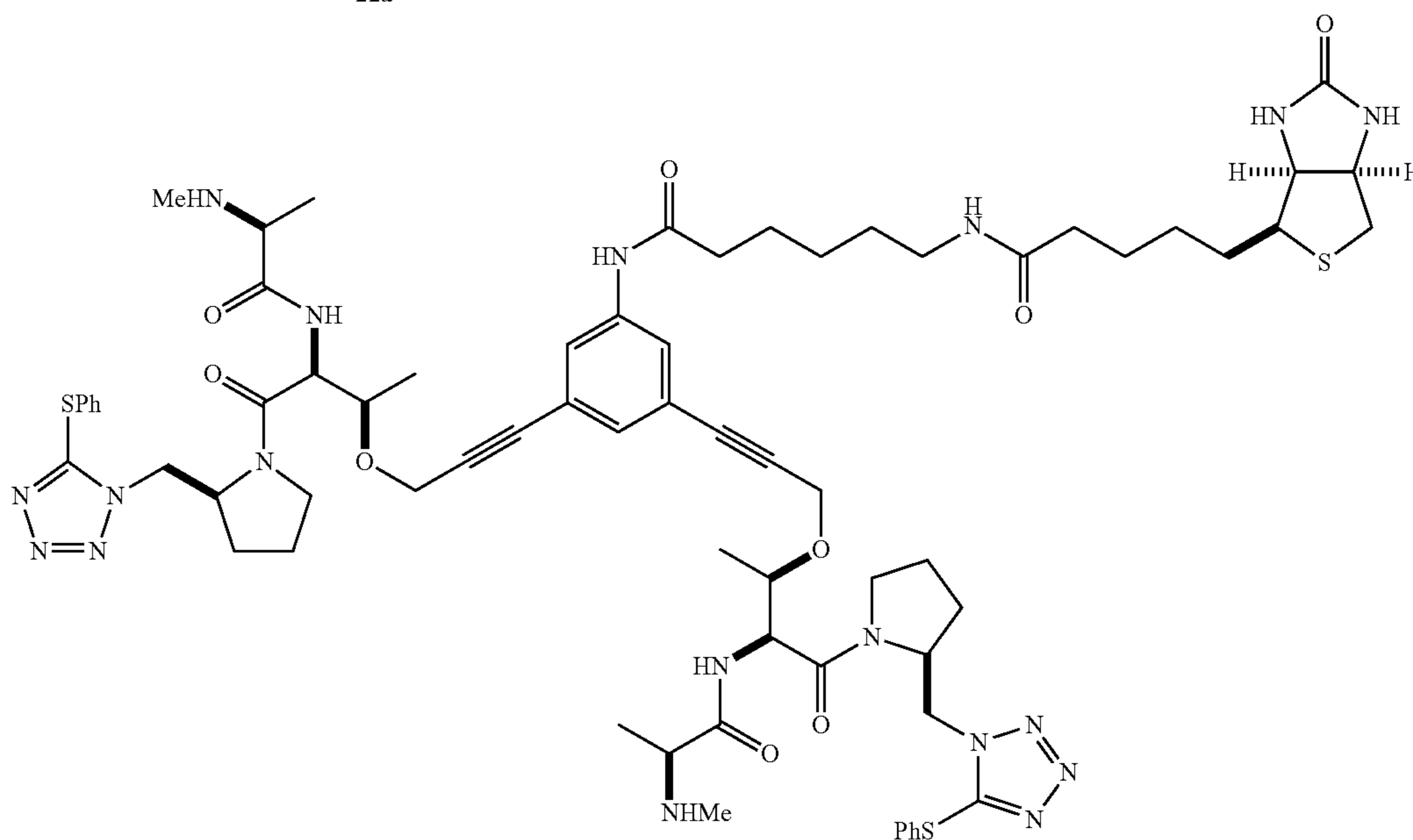
24a
