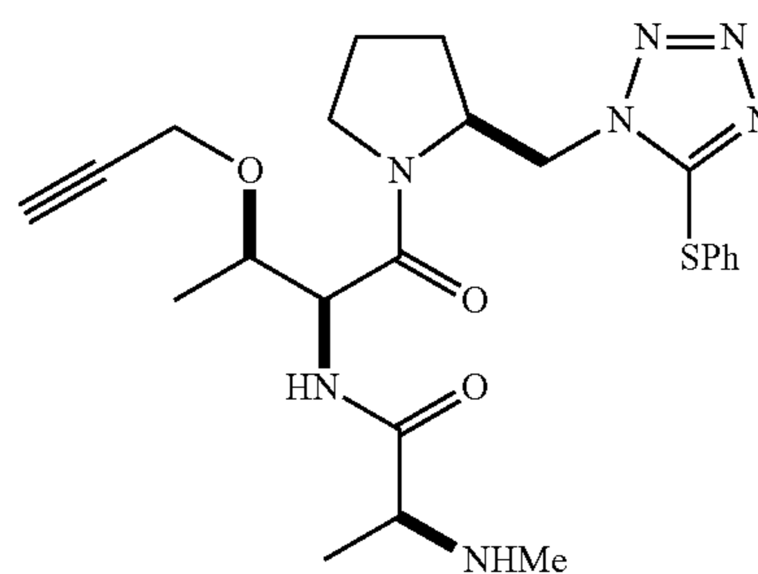
23a
