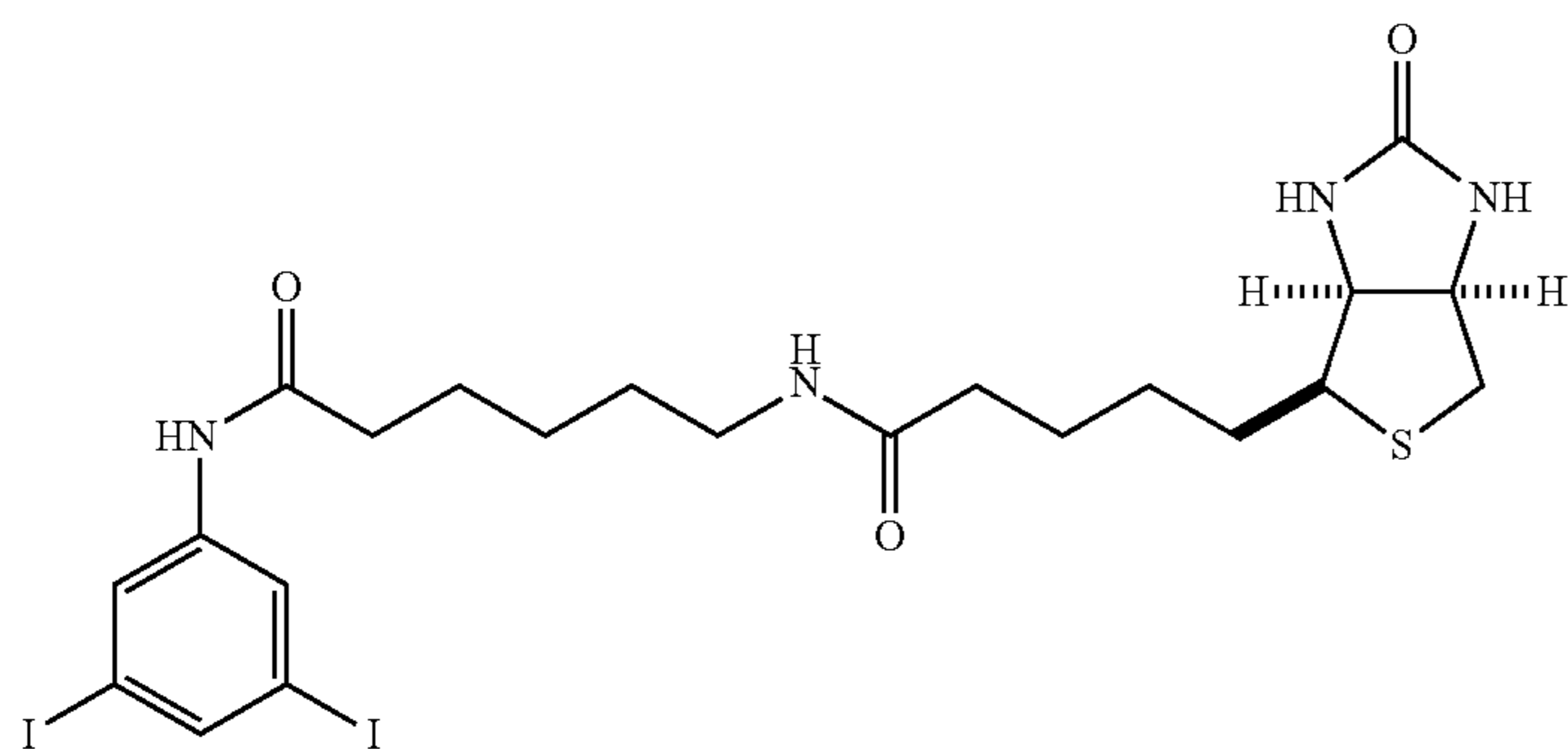
22a
