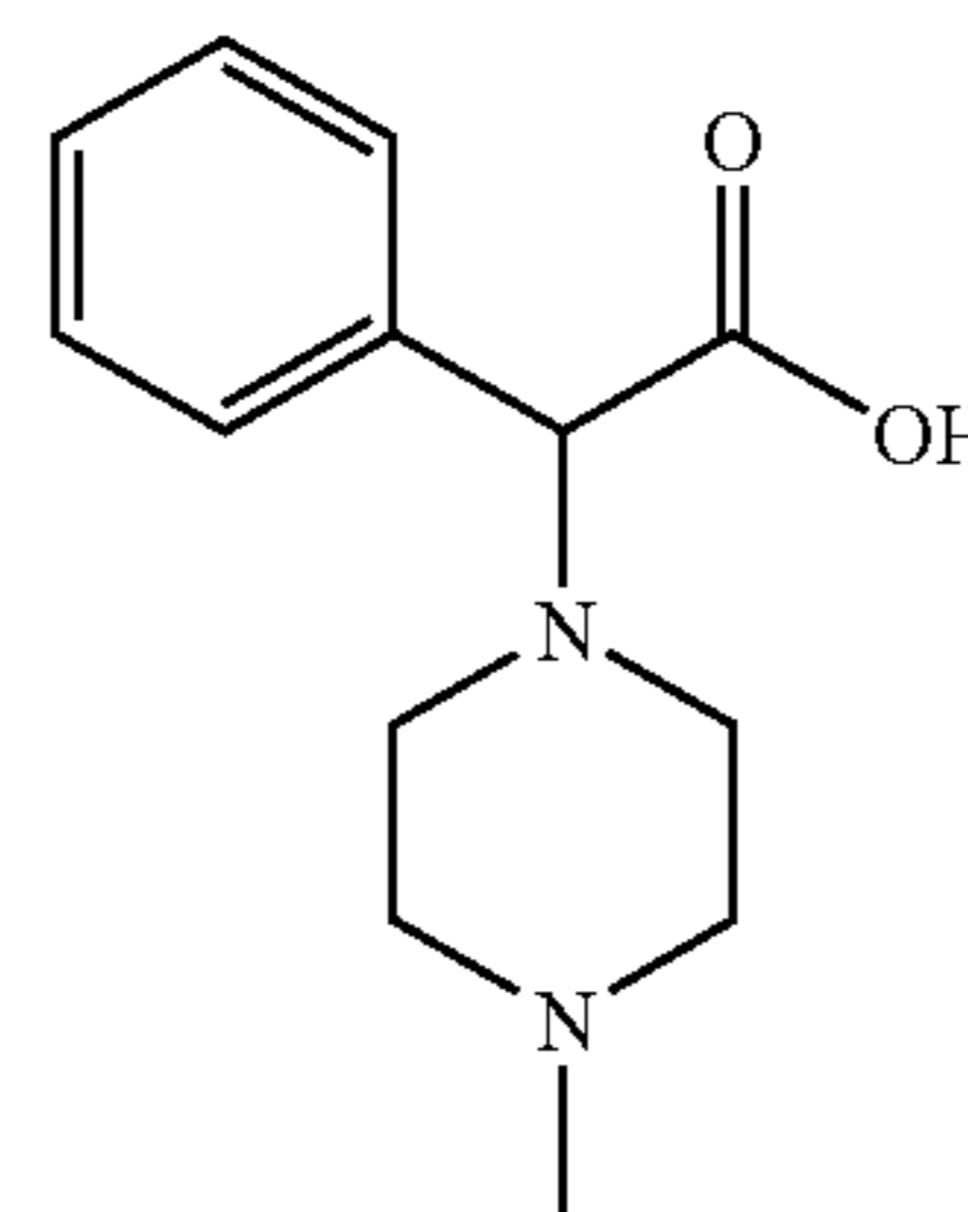
Cap-7a: enantiomer-2 Cap-7b: enantiomer-2
