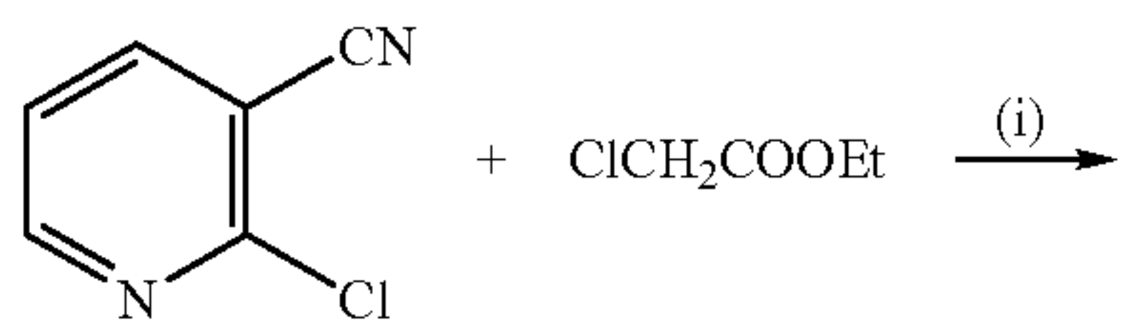
Scheme-E
