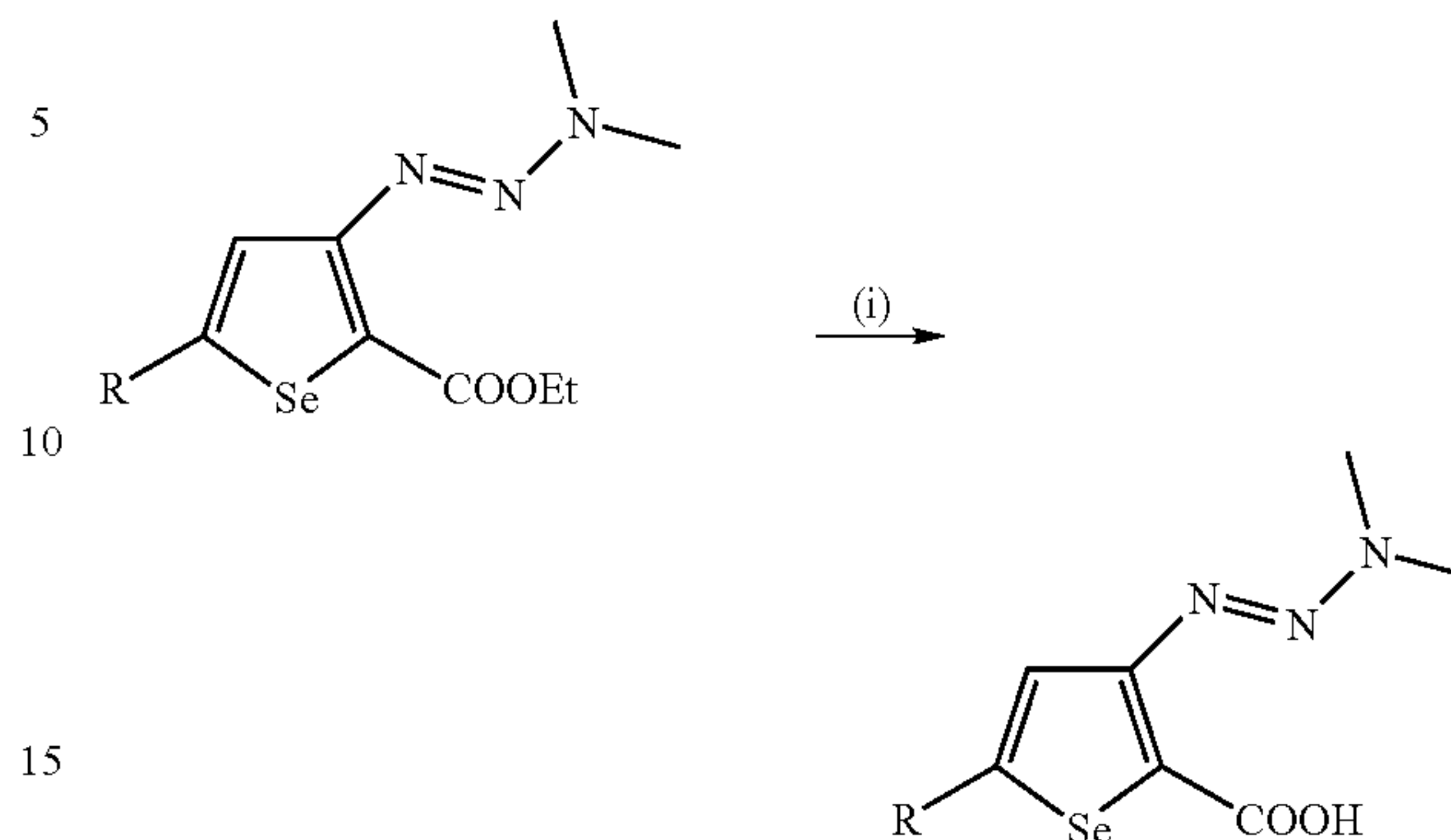
Scheme-F
