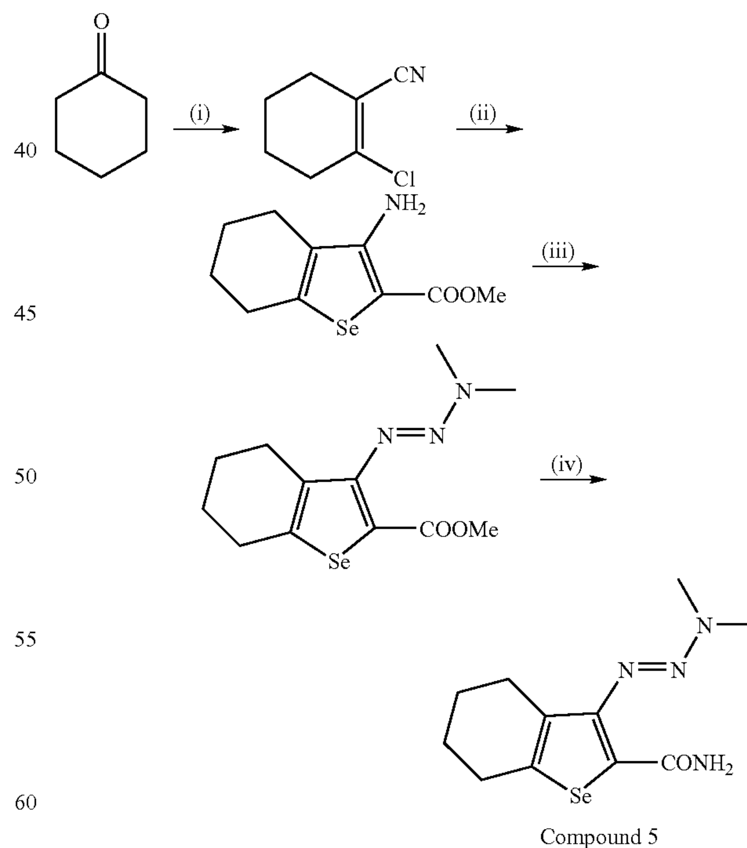
Scheme-D
