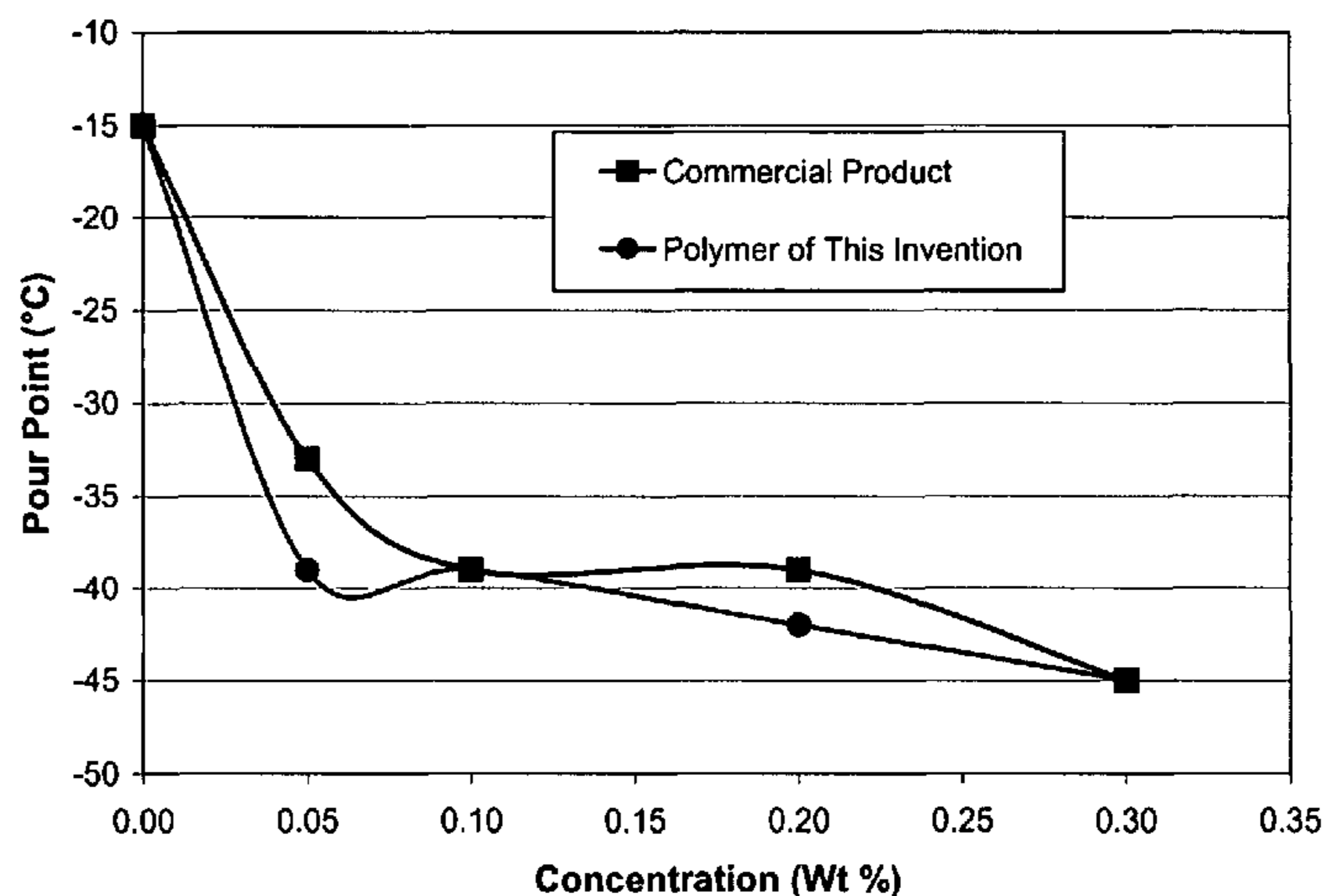
Pour Point in N100DW Oil
