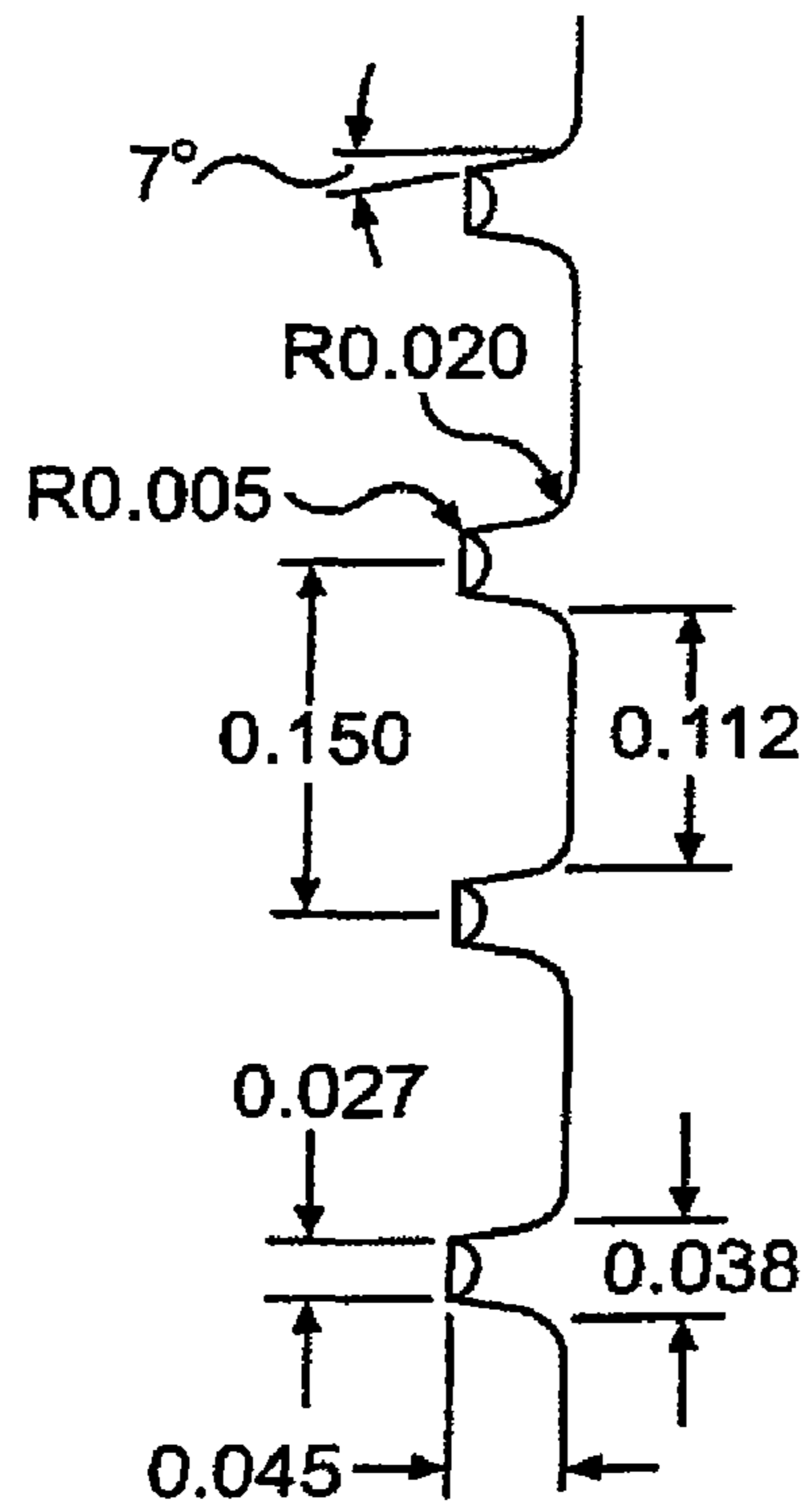
SECTION A-A
