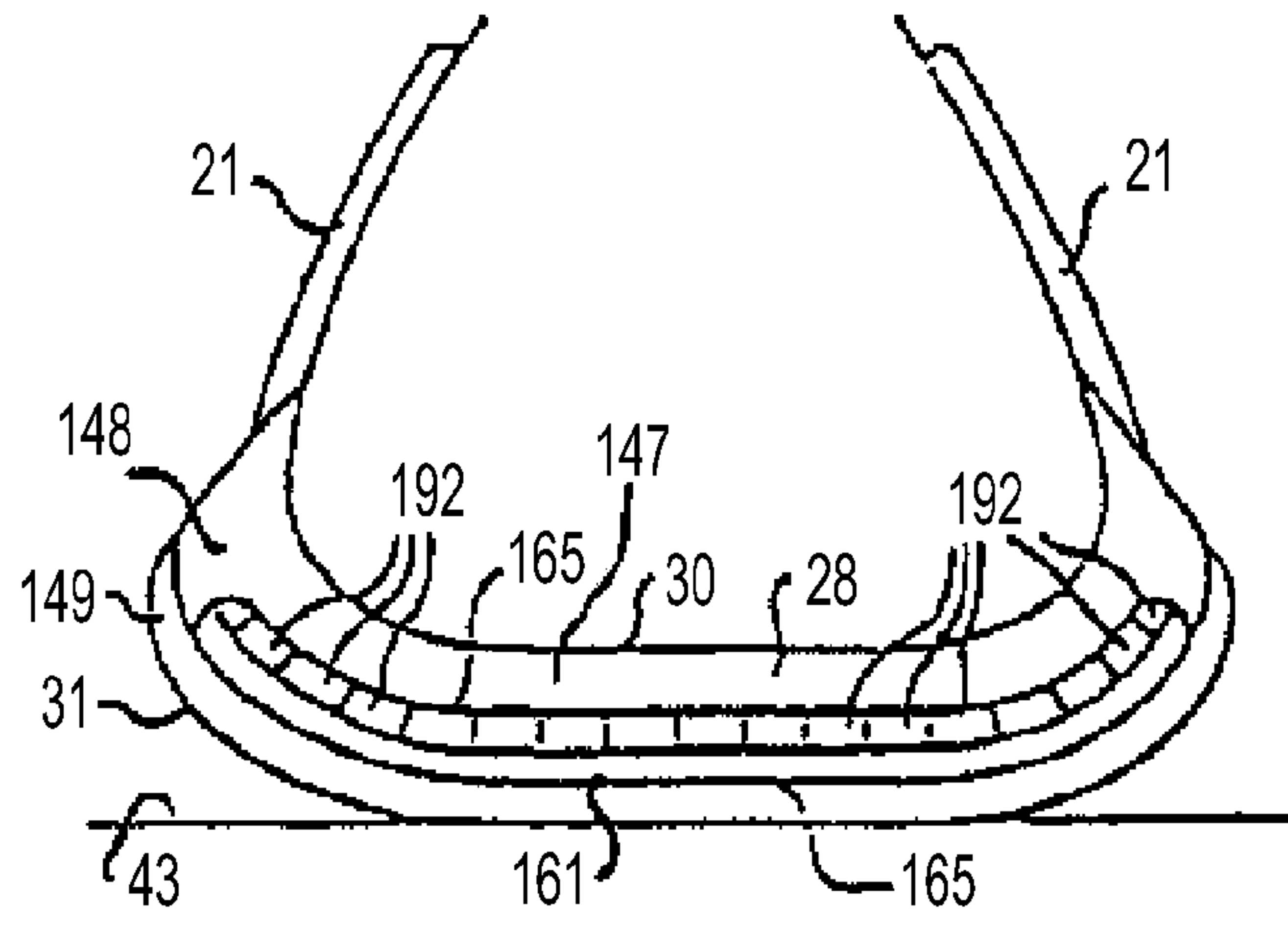
FIG. 59F PRIOR ART
