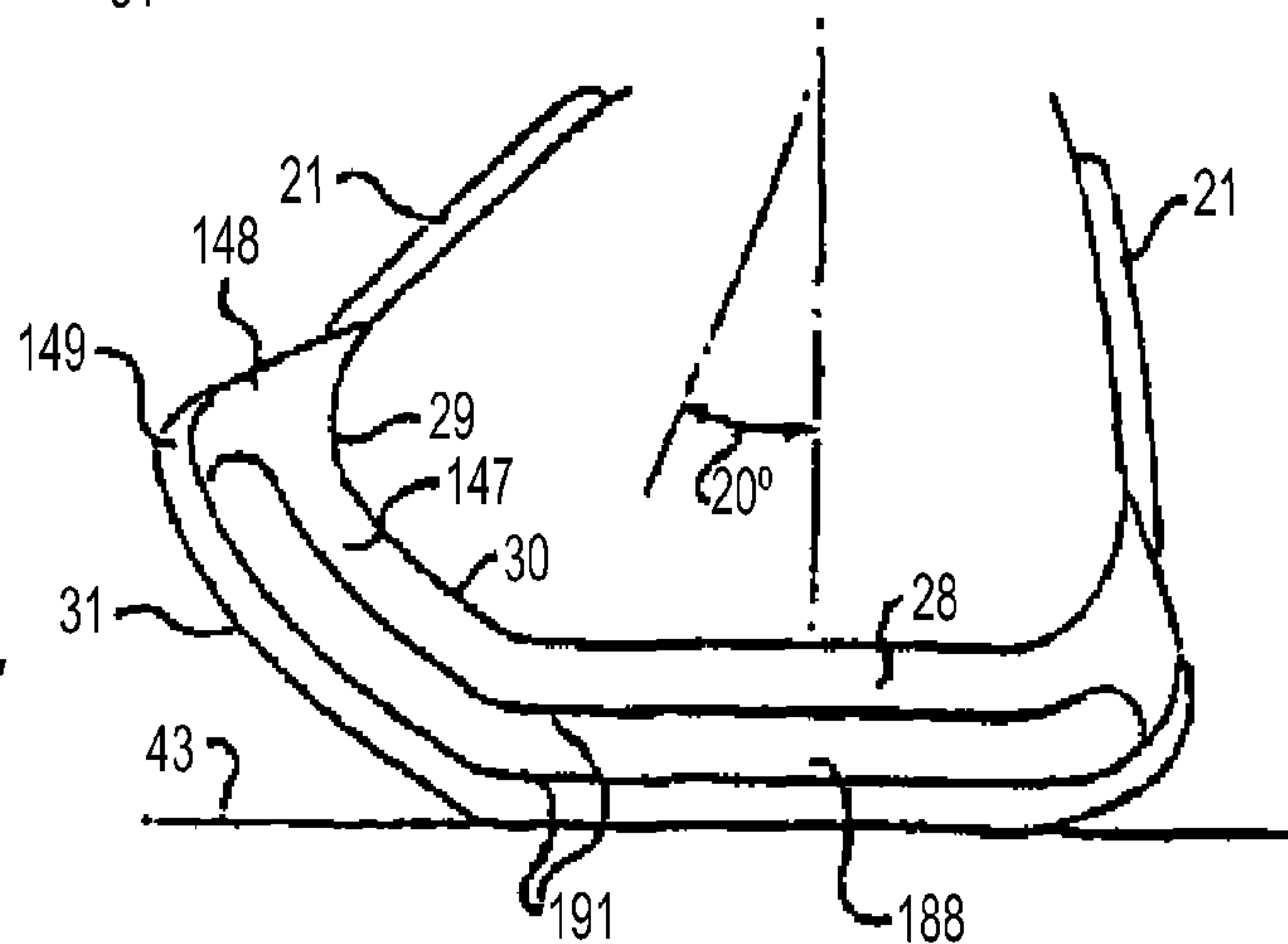
FIG. 60E PRIOR ART
