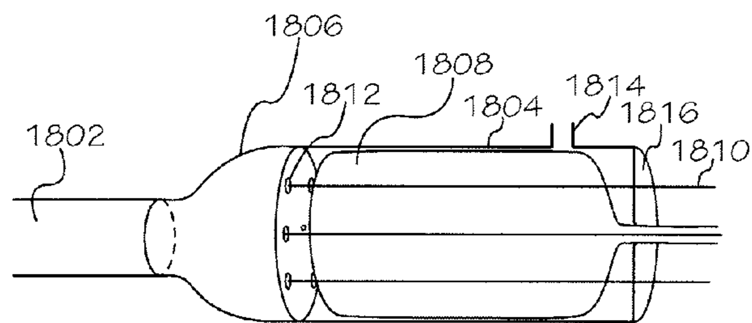
FIG 18A
