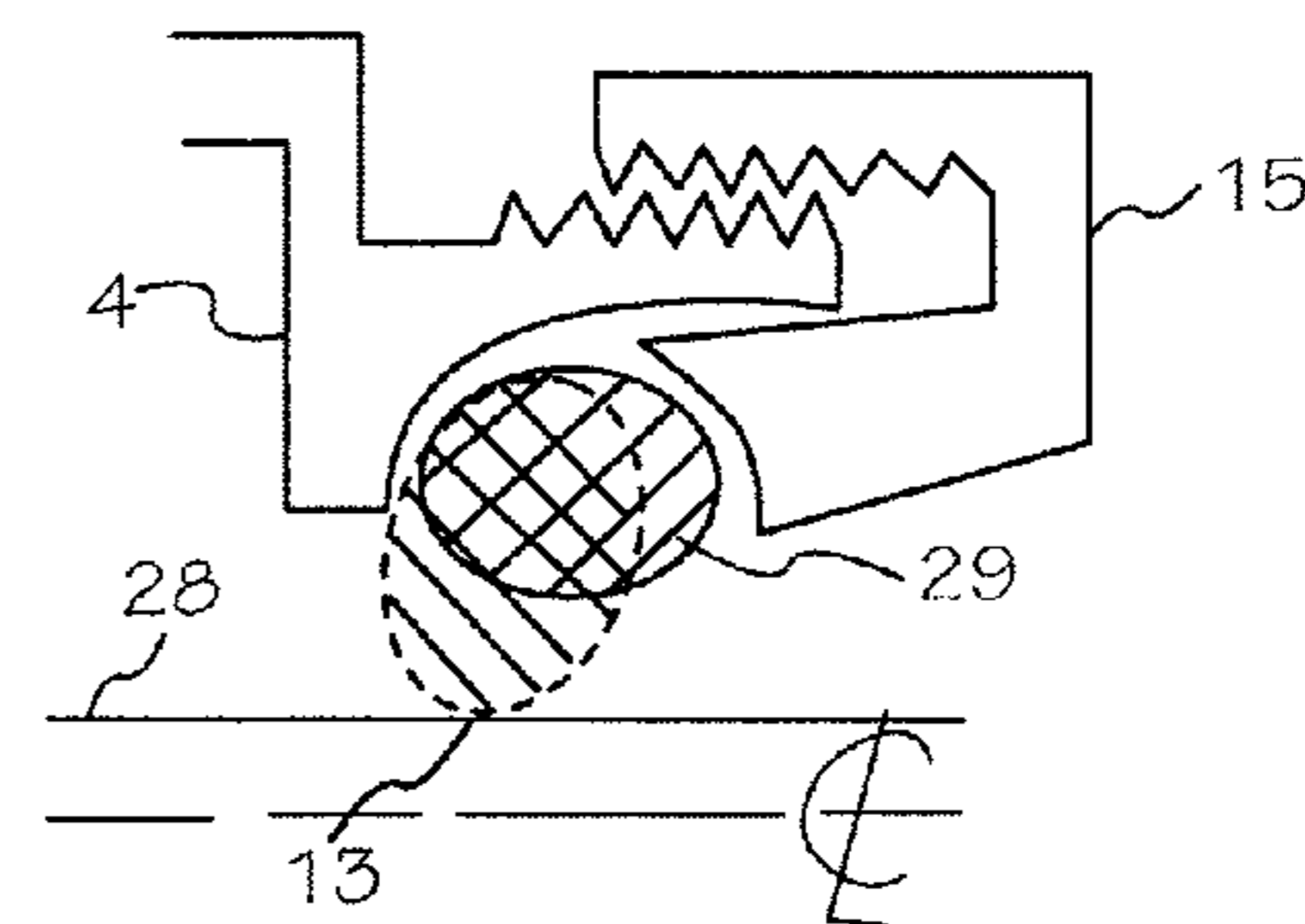
FIG 5F
