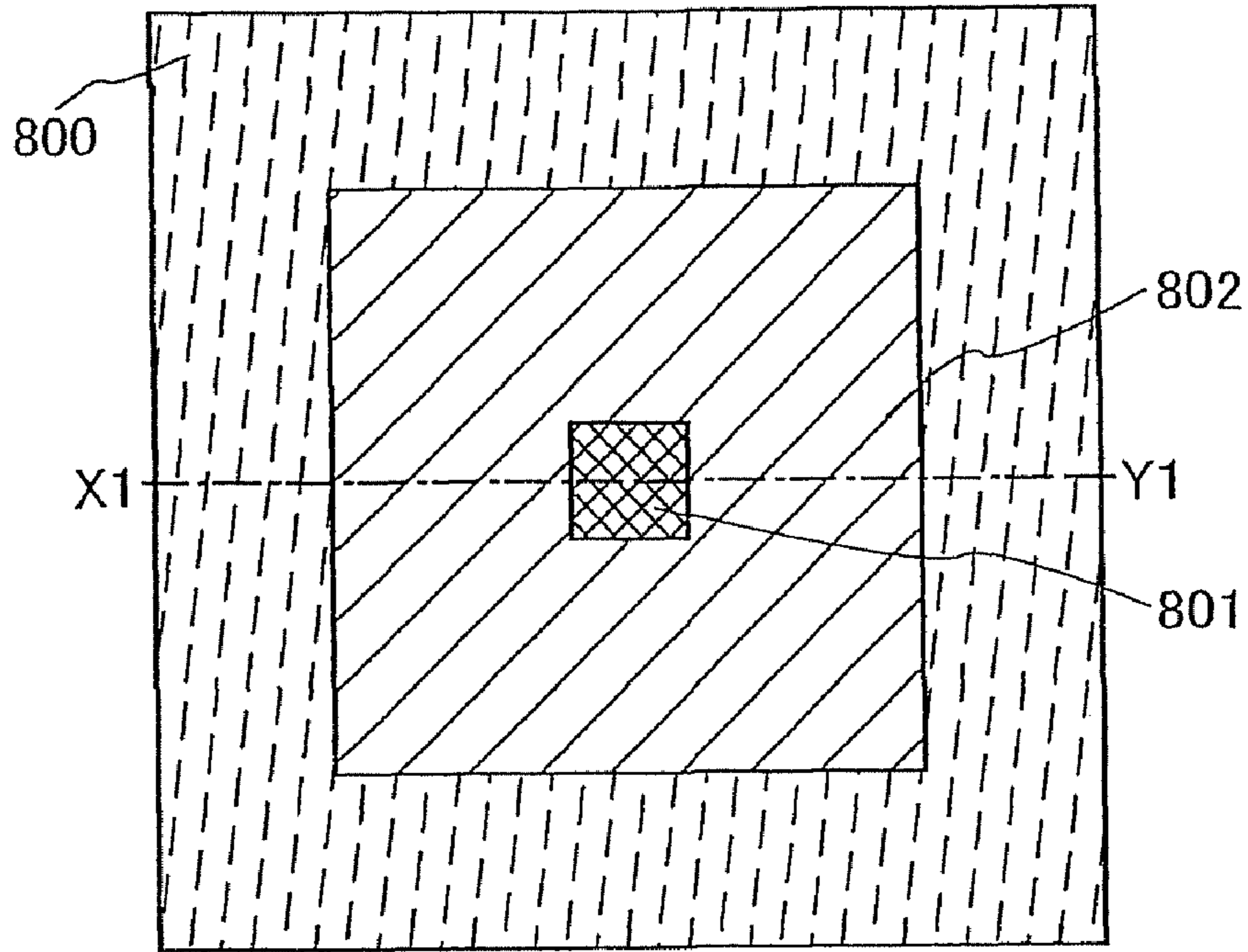
FIG. 27A
