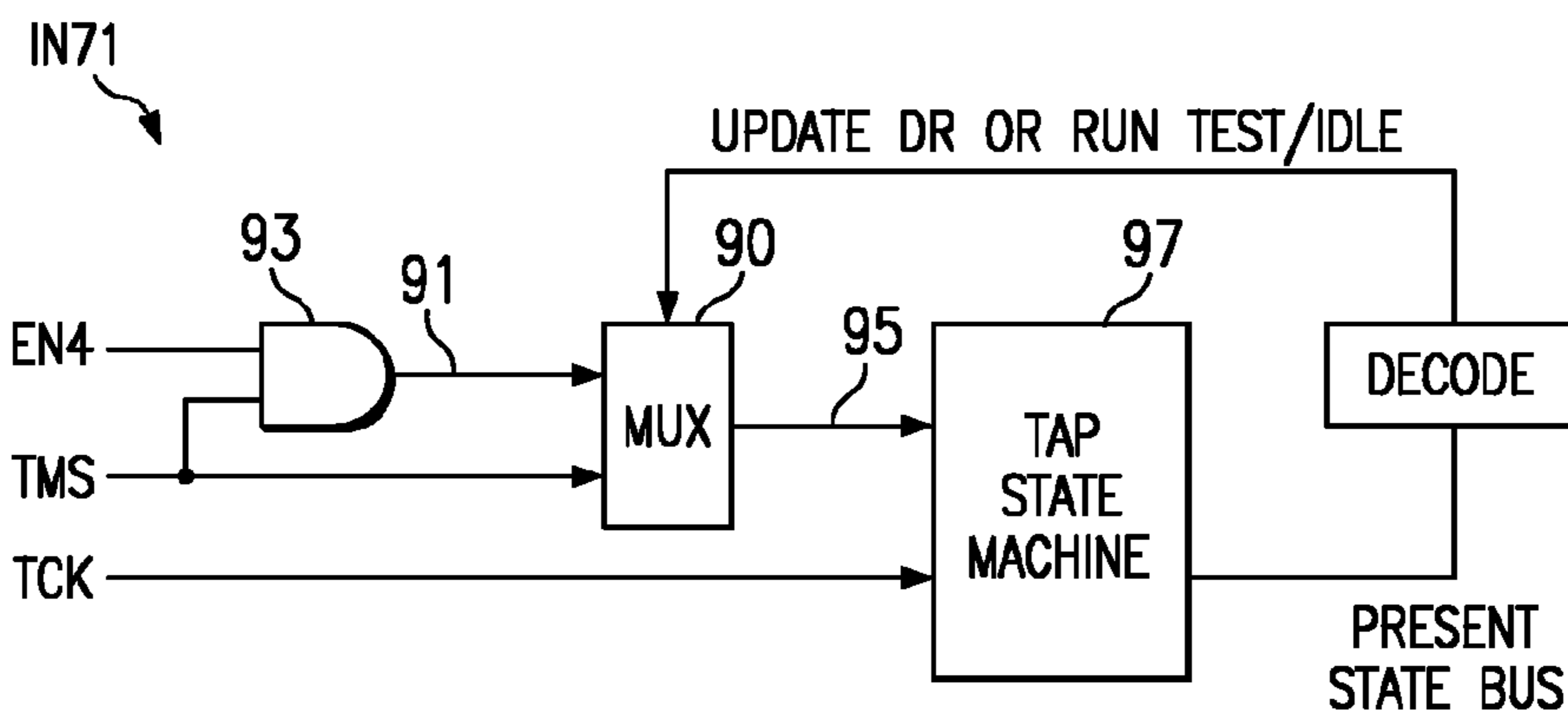
FIG. 9A
