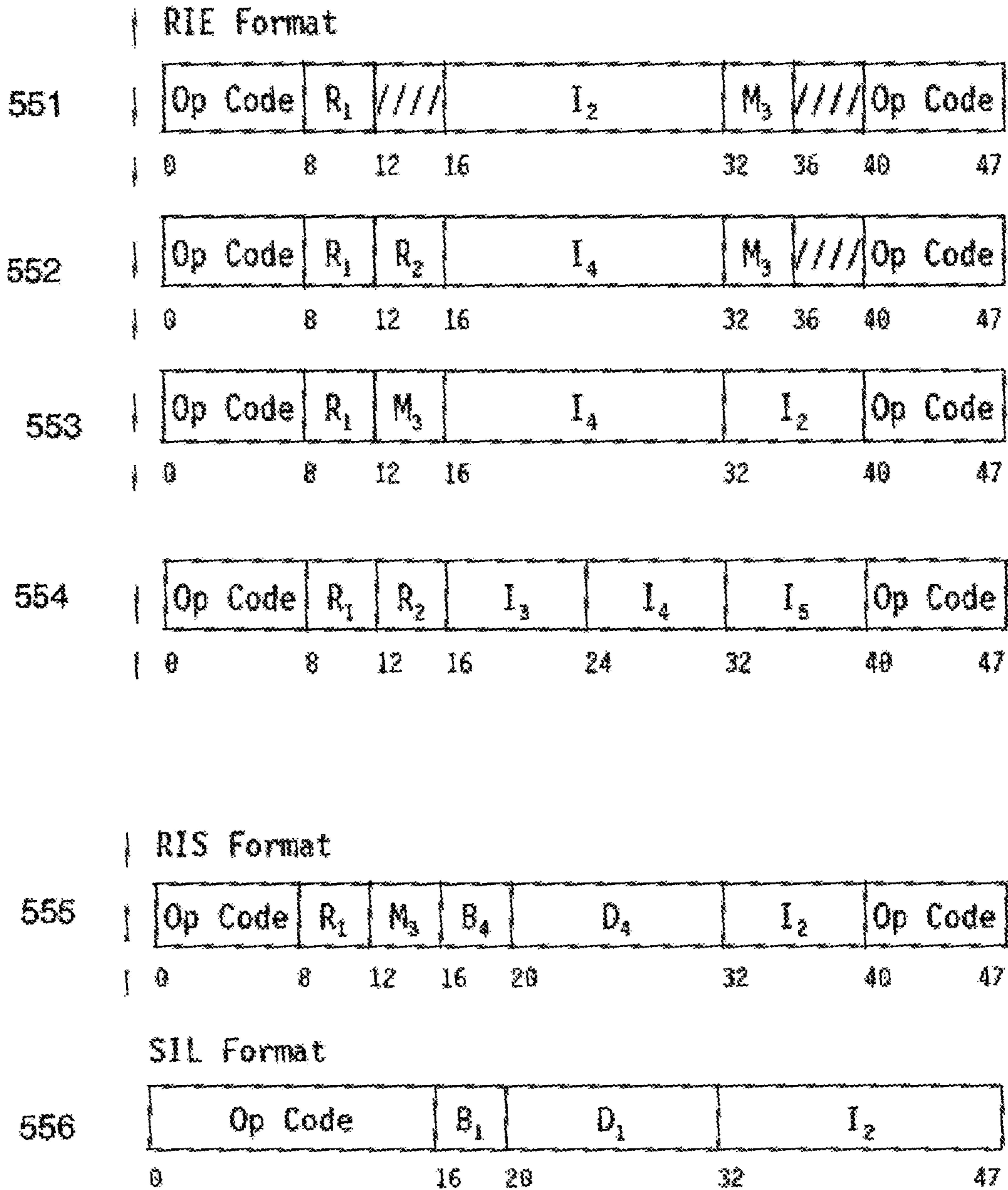
FIG. 5F
