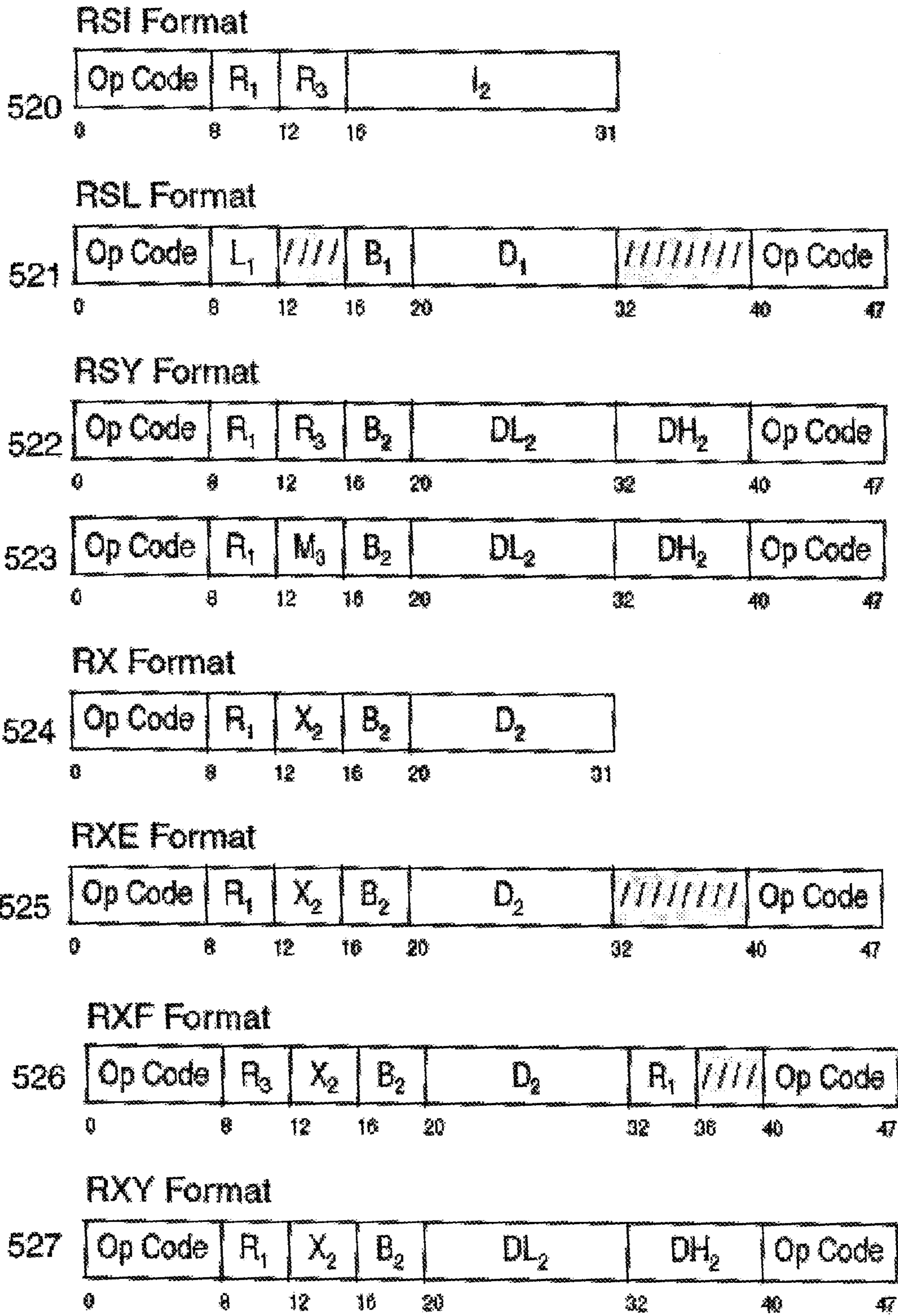
FIG. 5C
