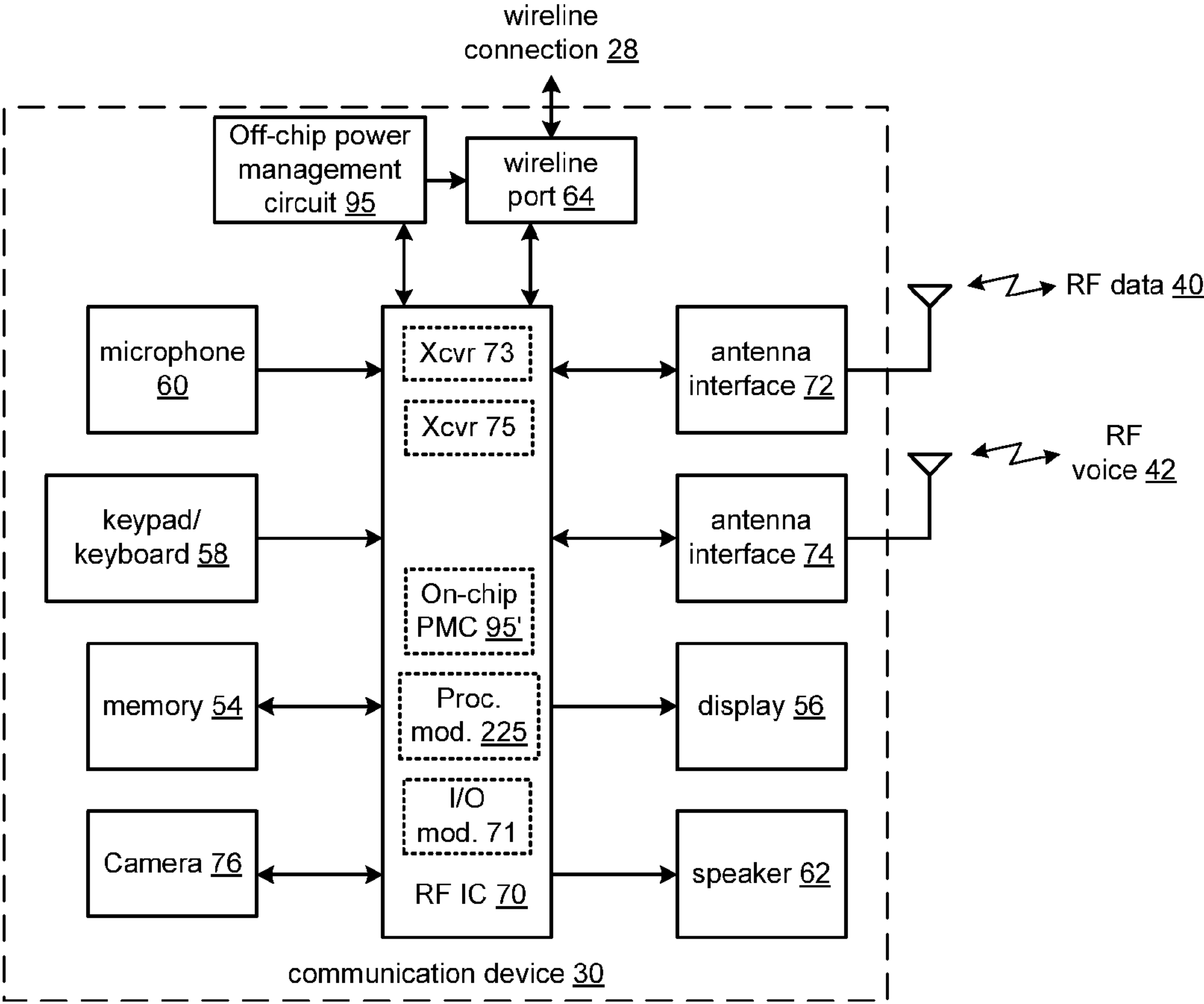
FIG. 4
