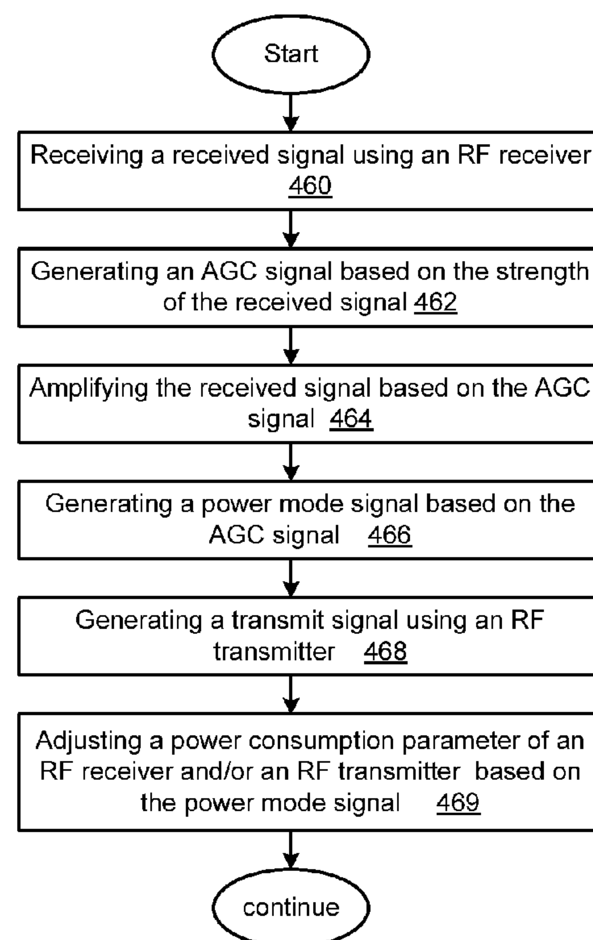
FIG. 27
