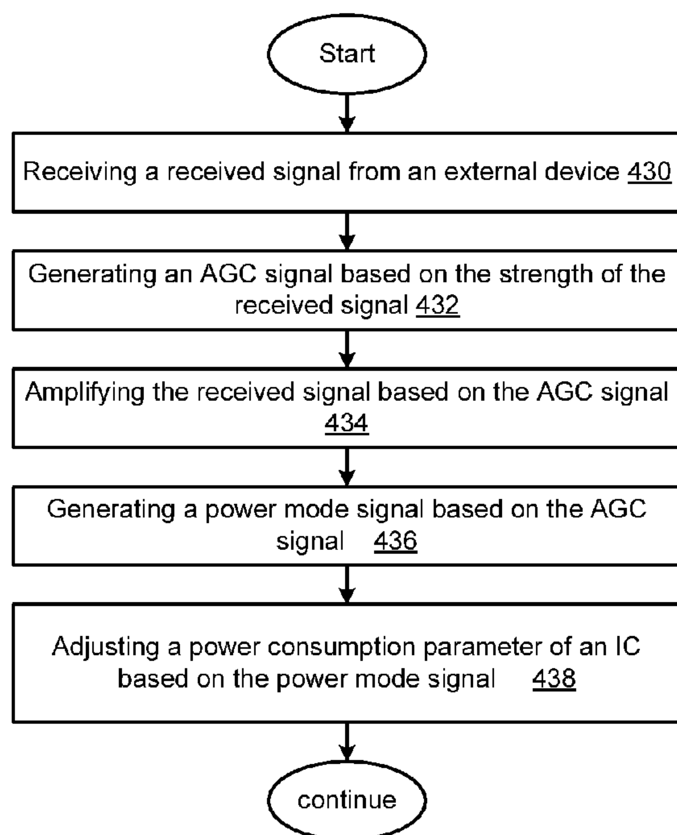
FIG. 24
