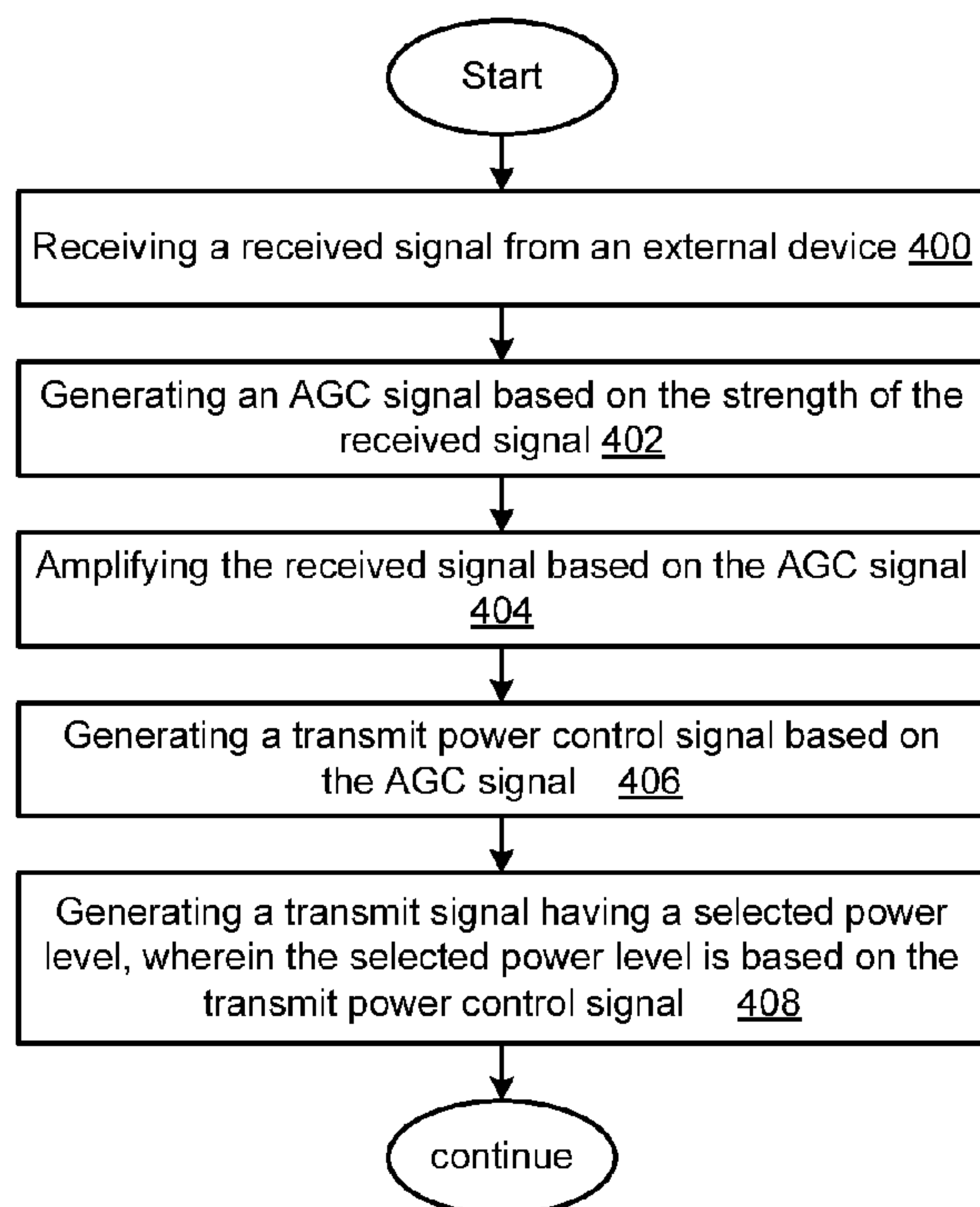
FIG. 21
