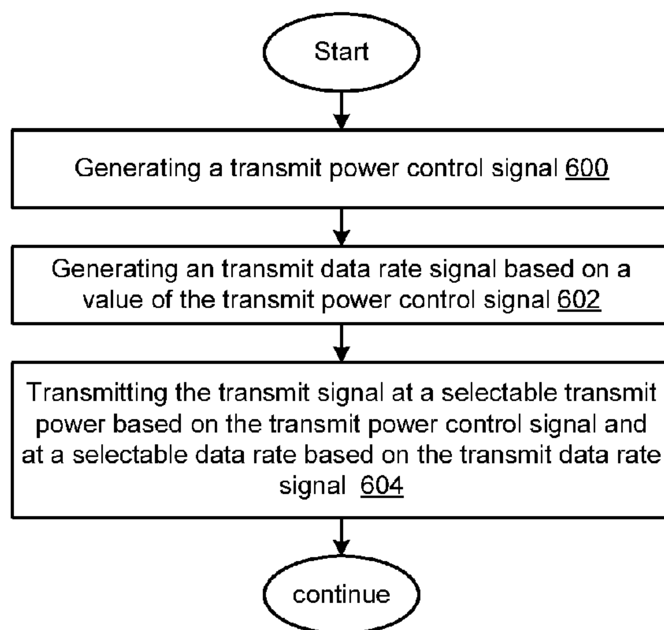
FIG. 32
