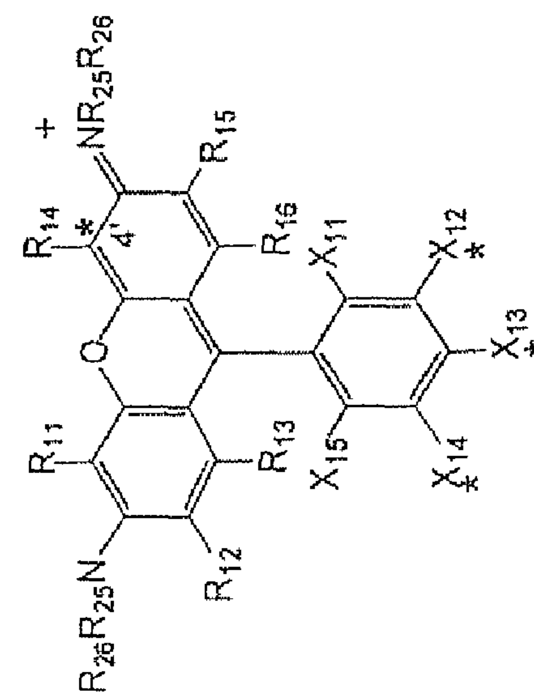
RHODAMINE
