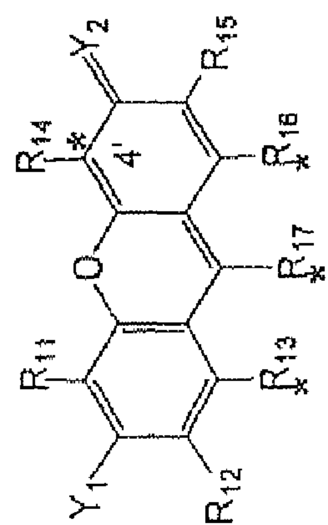
XANTHENE
