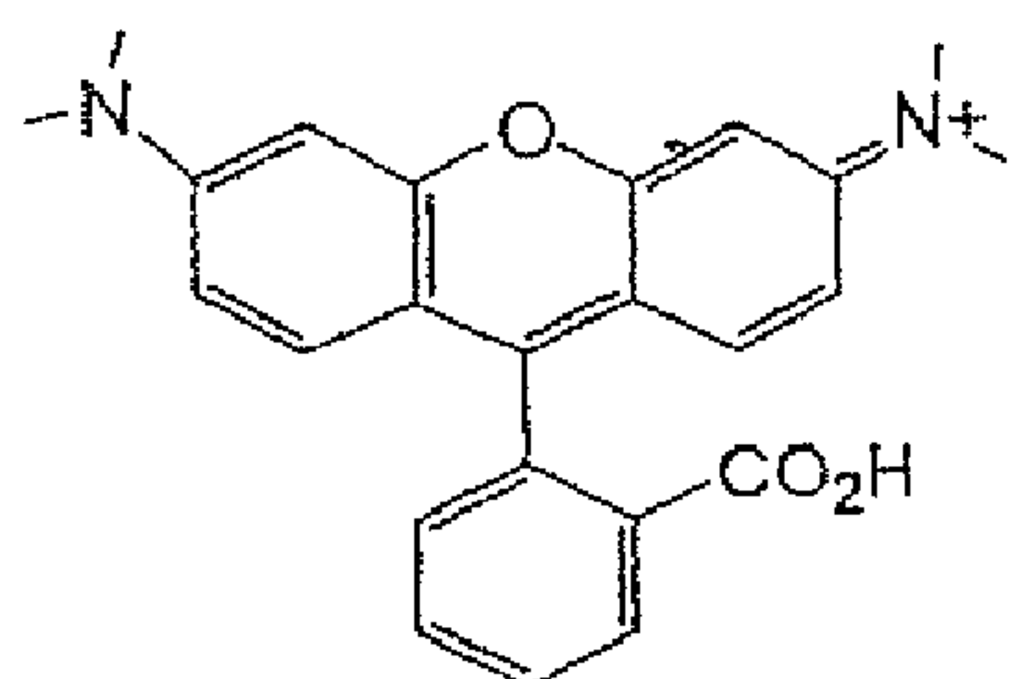
Rhodamine
