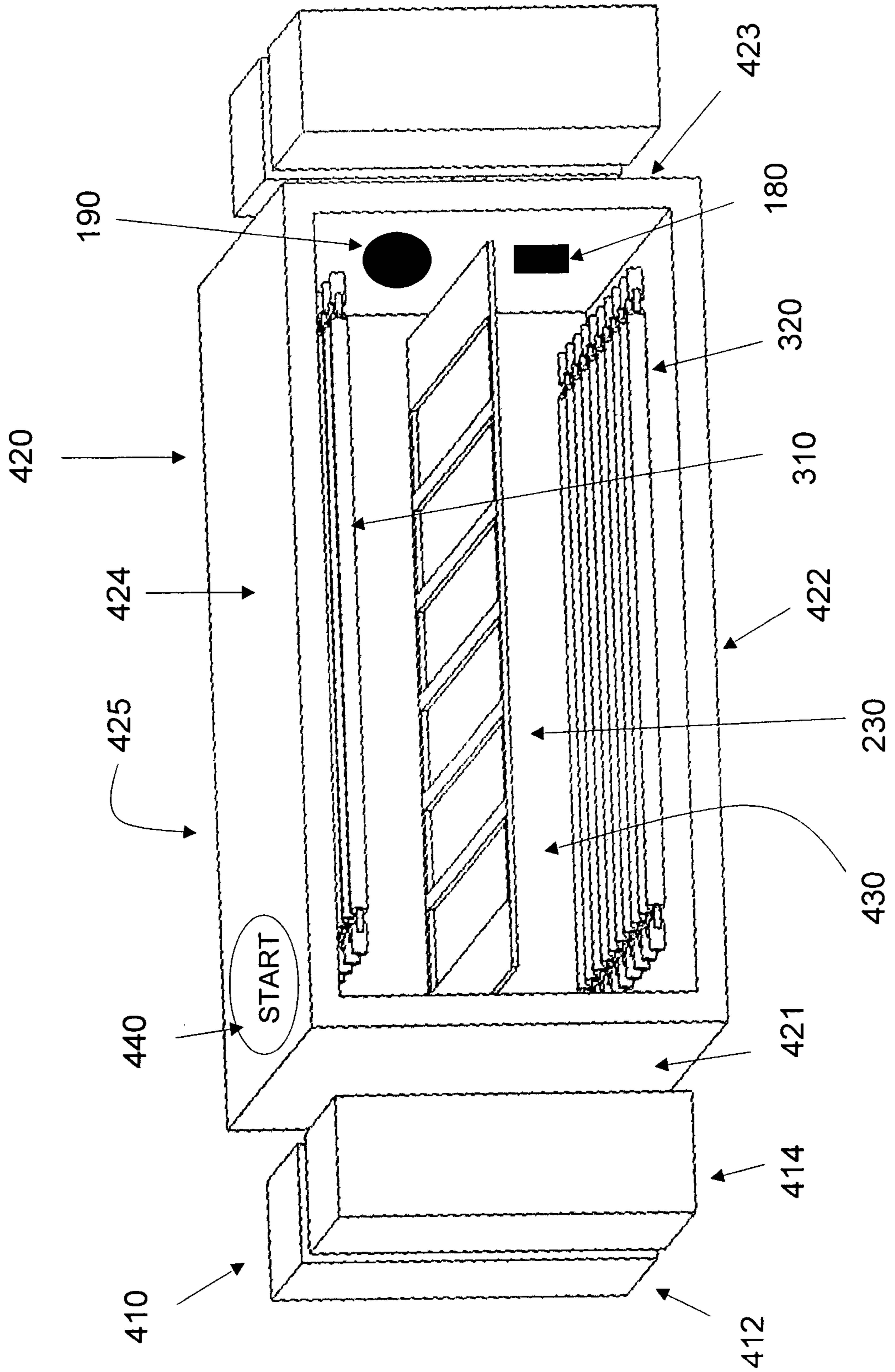
FIG. 4 RADIANT OVEN
