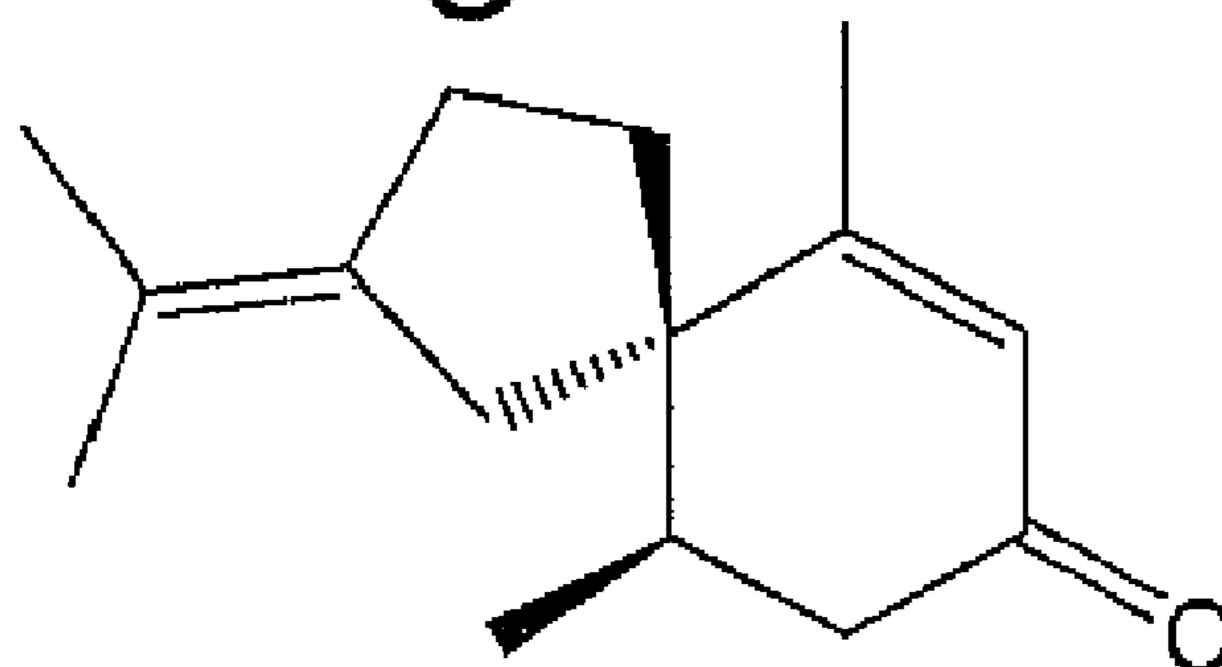
5-epi-β-vetivone (1)
