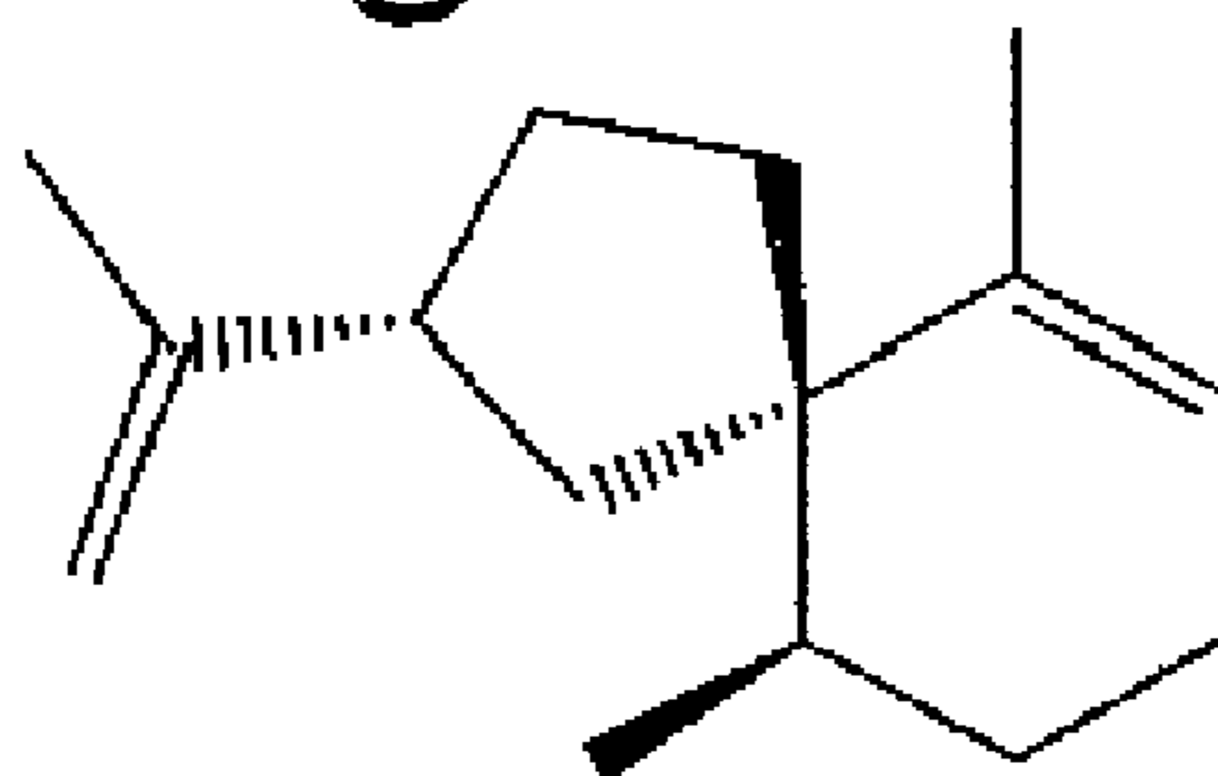
(-)-Premnaspirdiene (2)
