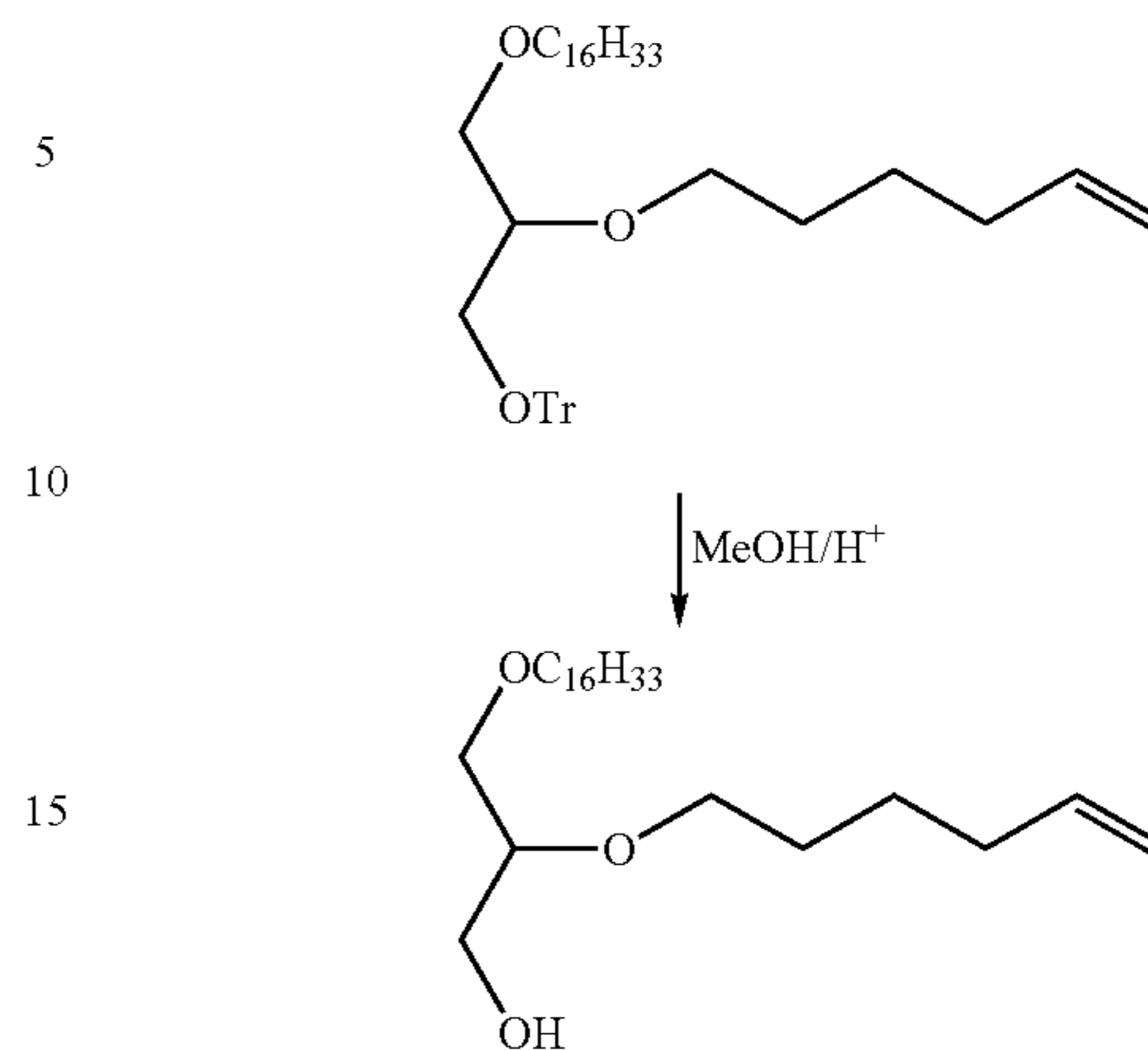
Scheme VI
