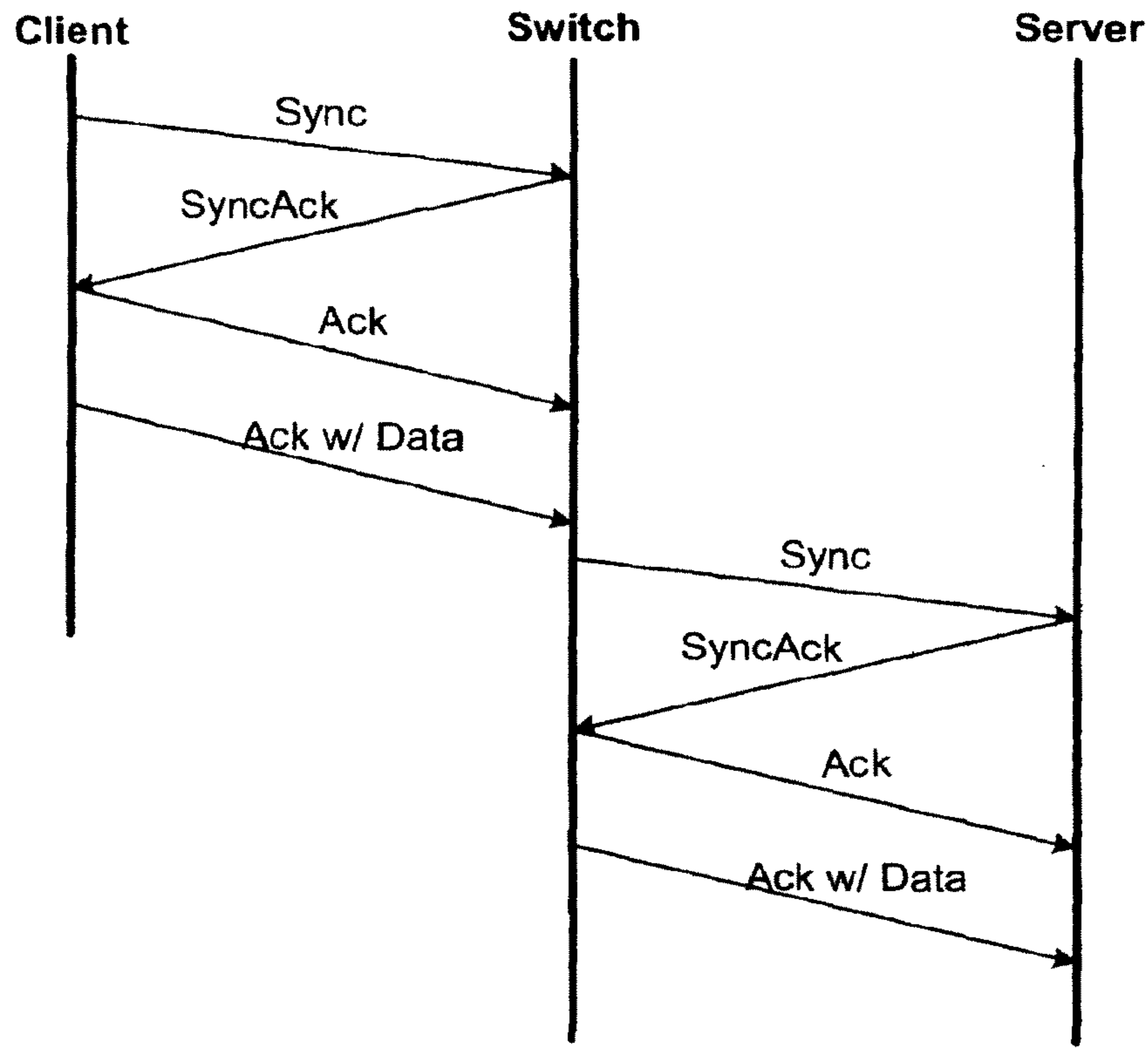
FIG. 17 TCP Slicing
