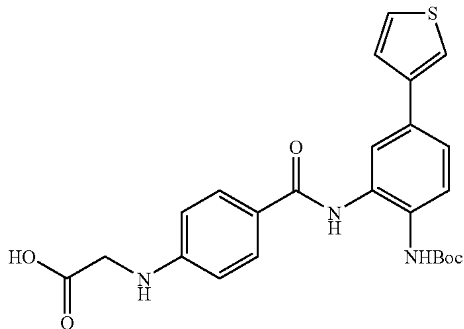
{[4-([2-[(tert-butoxycarbonyl)amino]-5-(3-thienyl)phenyl]amino}carbonyl)phenyl]amino}acetic acid
