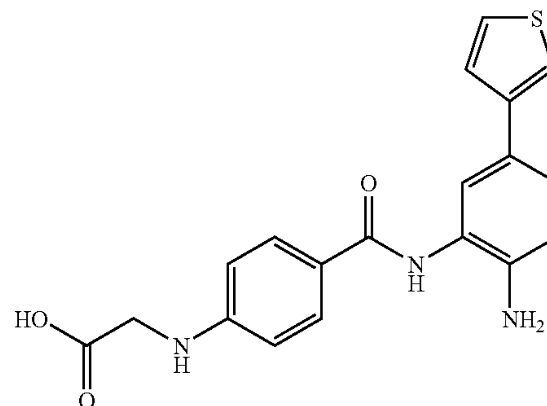
{[4-([2-[(tert-butoxycarbonyl)amino]-5-(3-thienyl)phenyl]amino}carbonyl)phenyl]amino}acetic acid
