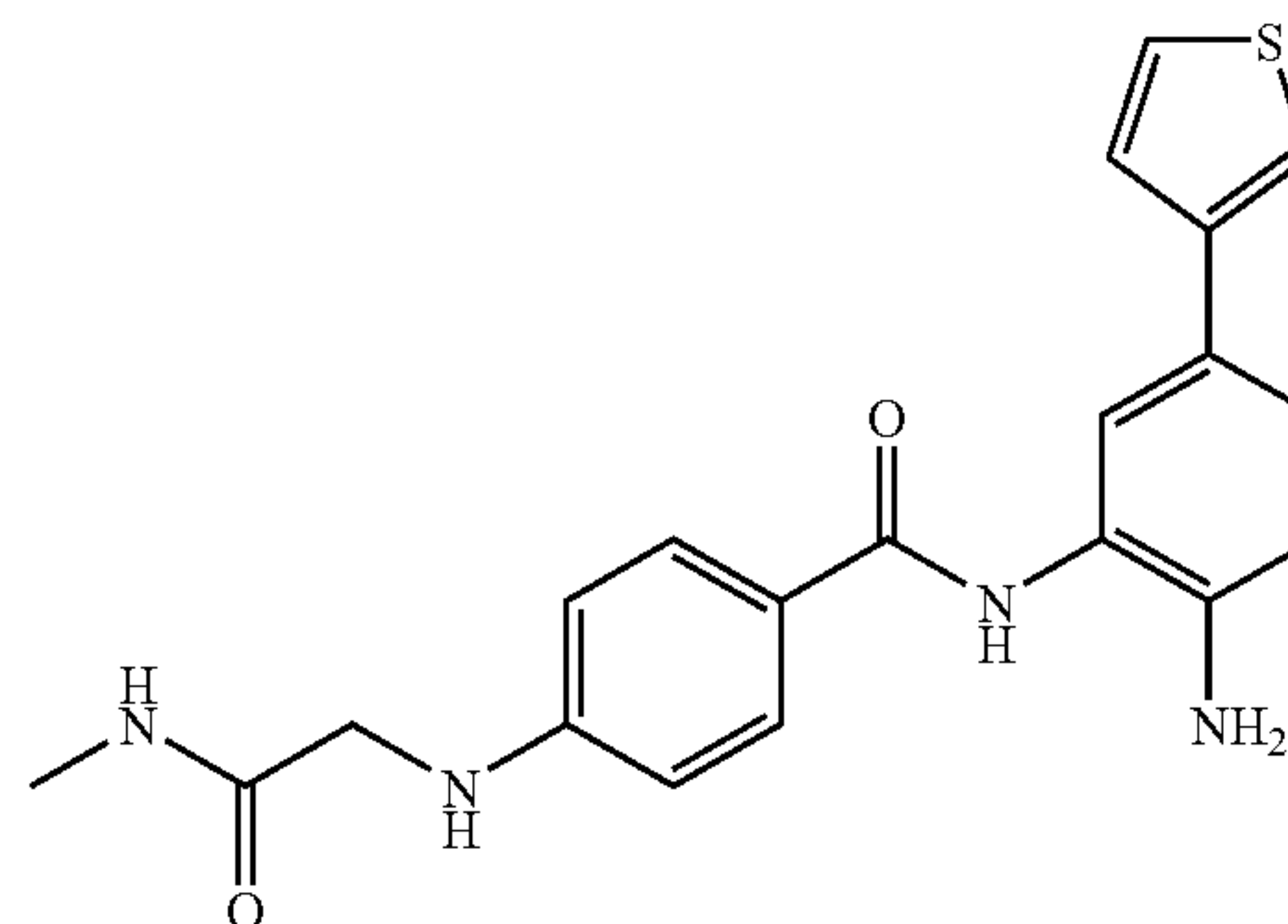
N-[2-amino-5-(3-thienyl)phenyl]-4-[(2-(methylamino)-2-oxoethyl)amino]benzamide
