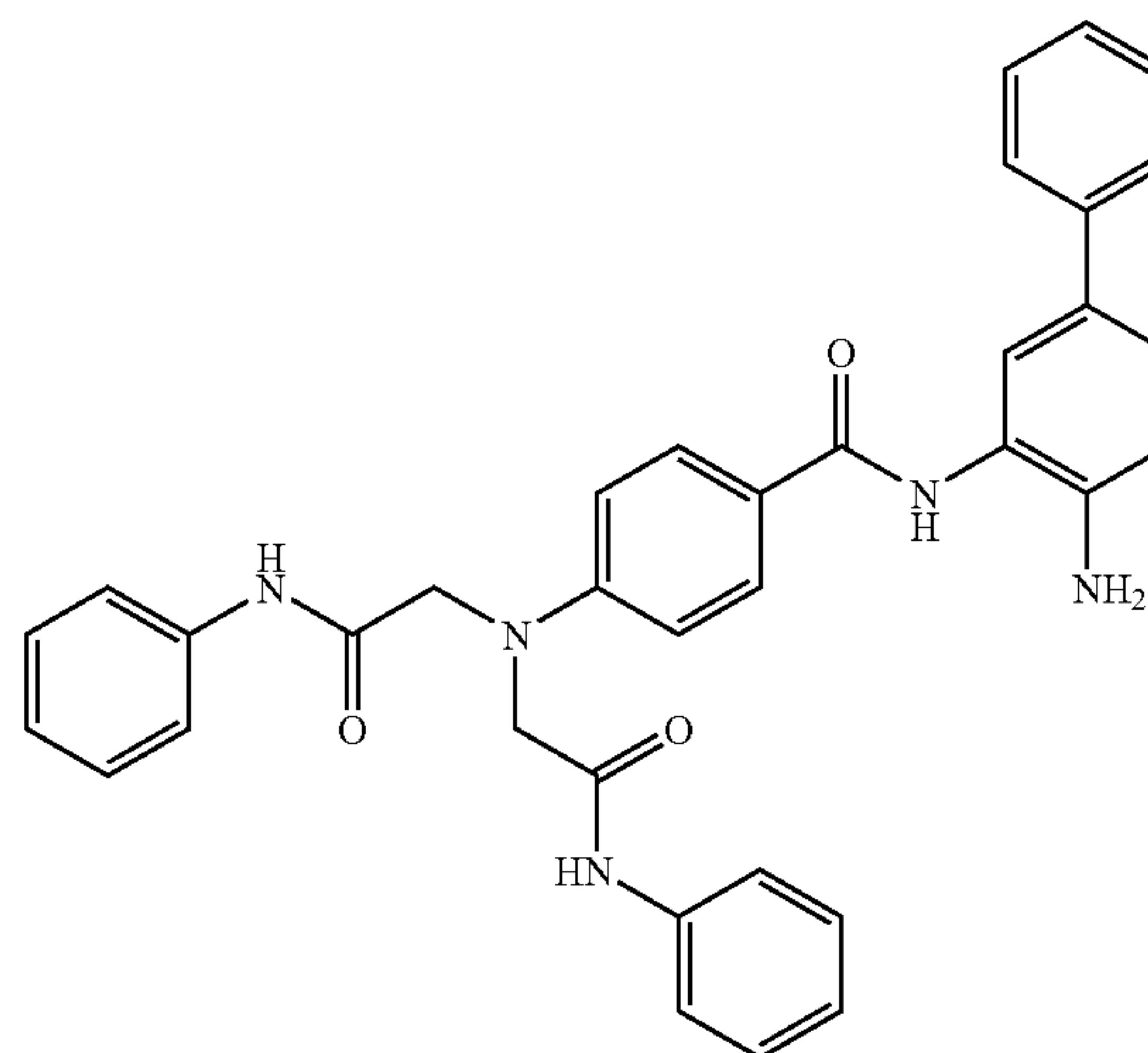
N-(4-aminobiphenyl-3-yl)-4-[bis(2-anilino-2-oxoethyl)amino]benzamide
