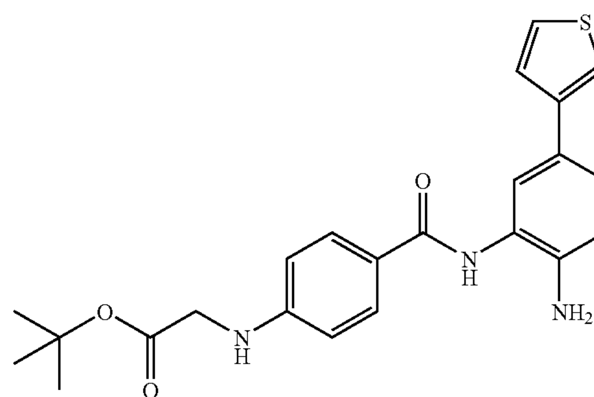
tert-Butyl[4-([2-amino-5-(3-thienyl)phenyl]amino)carbonyl]phenyl]amino]acetate
