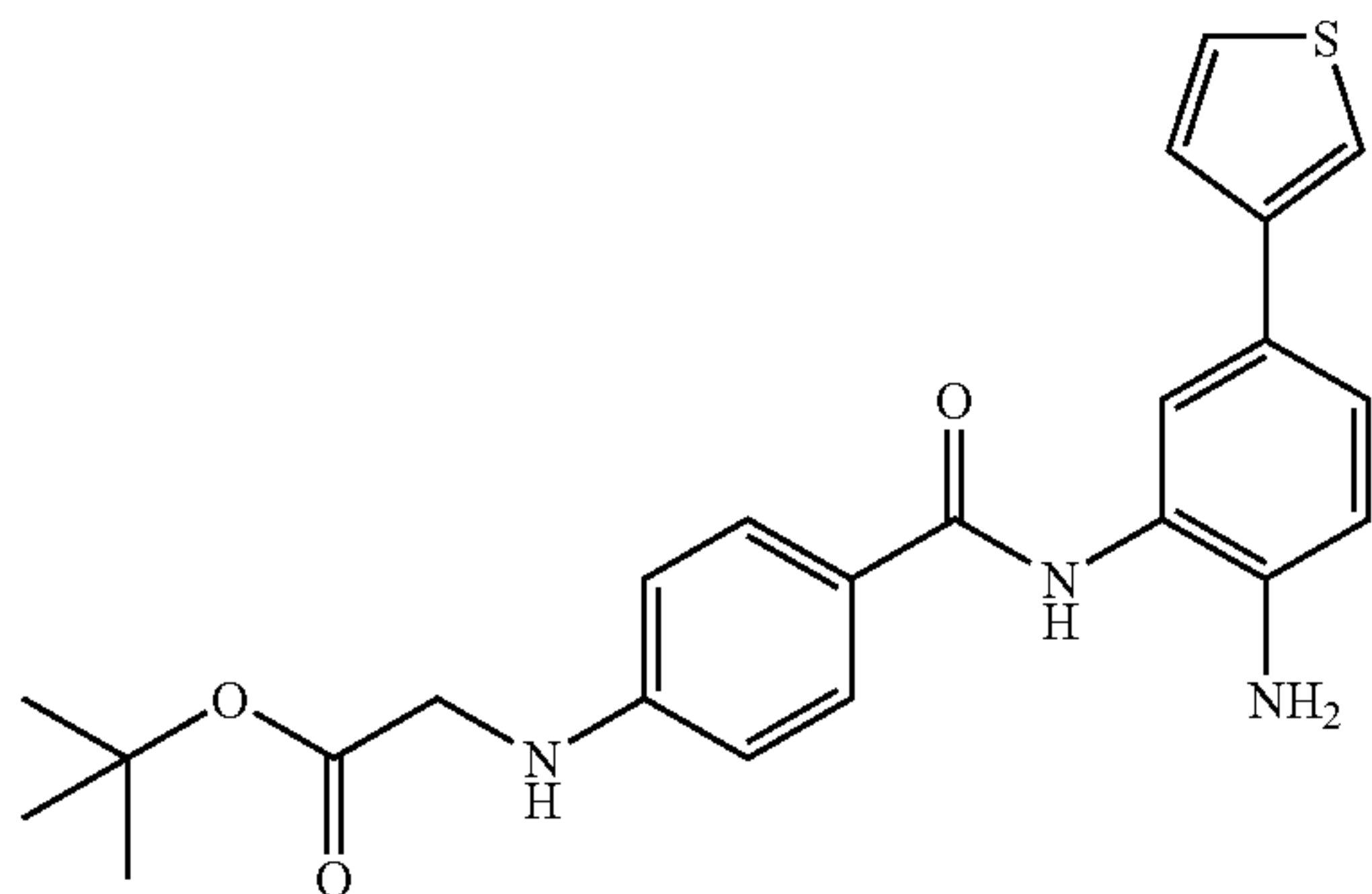
tert-Butyl [(4-{[2-amino-5-(3-thienyl)phenyl]amino}carbonyl)phenyl]amino]acetate
