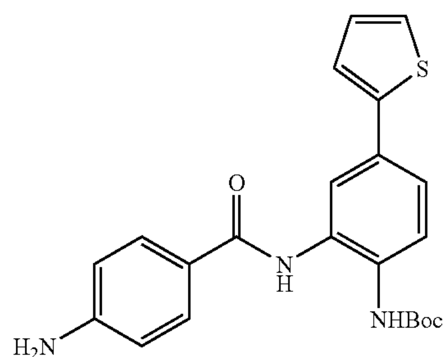
tert-Butyl [2-[(4-aminobenzoyl)amino]-4-(2-thienyl)phenyl]carbamate
