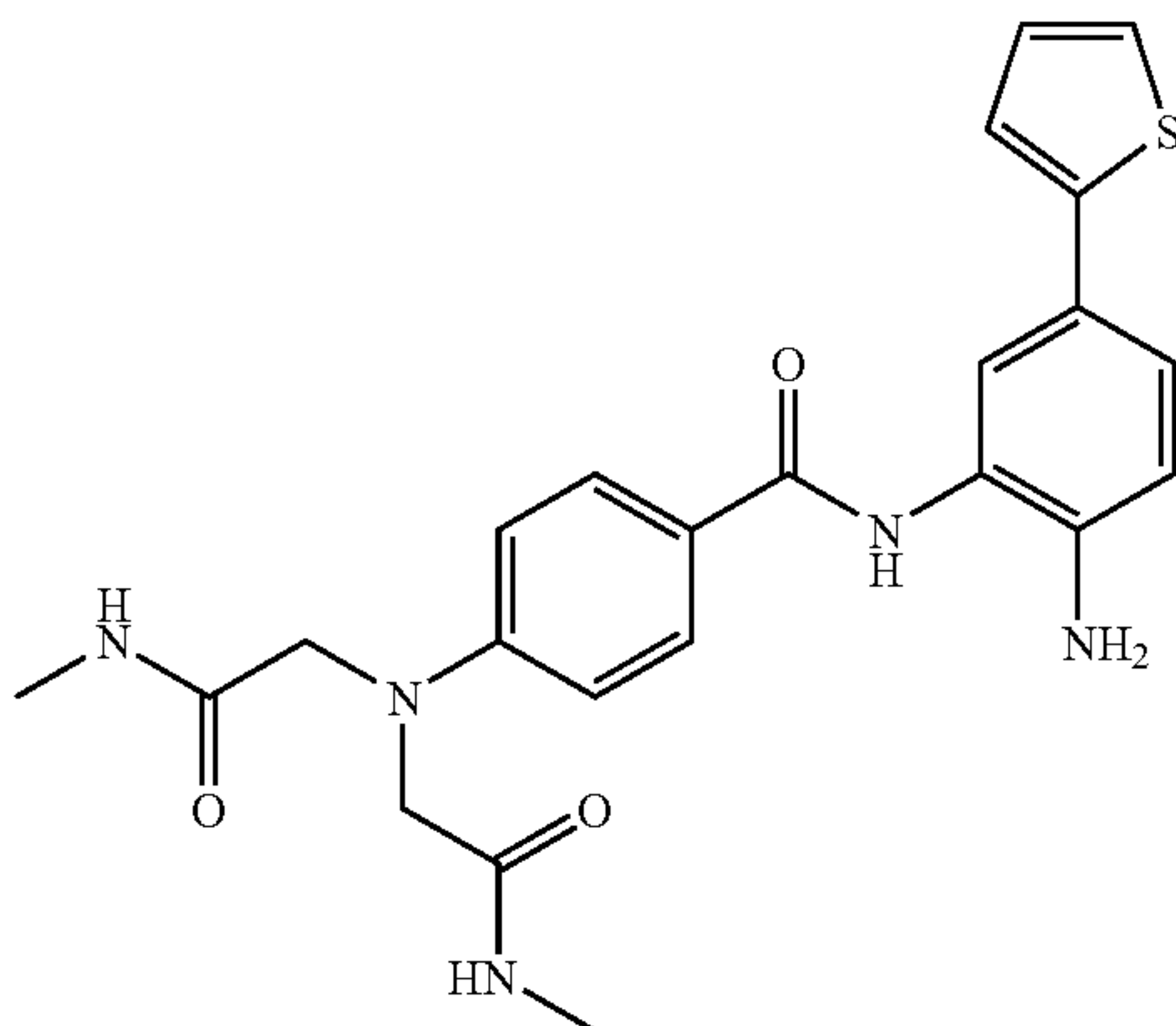
N-[2-amino-5-(2-thienyl)phenyl]-4-{bis[2-(methylamino)-2-oxoethyl]amino}benzamide
