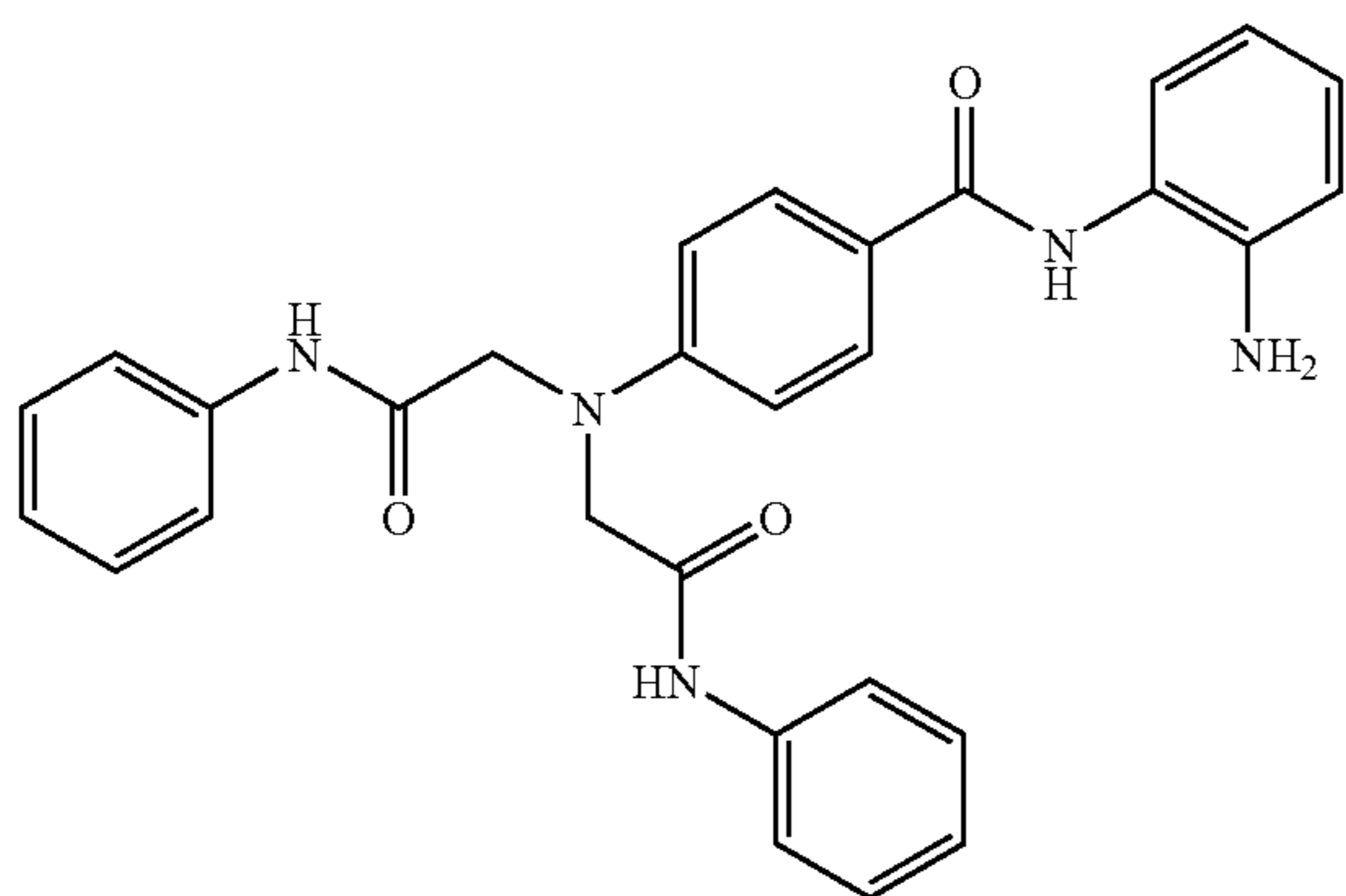
N-(2-aminophenyl)-4-[bis(2-anilino-2-oxoethyl) amino]benzamide
