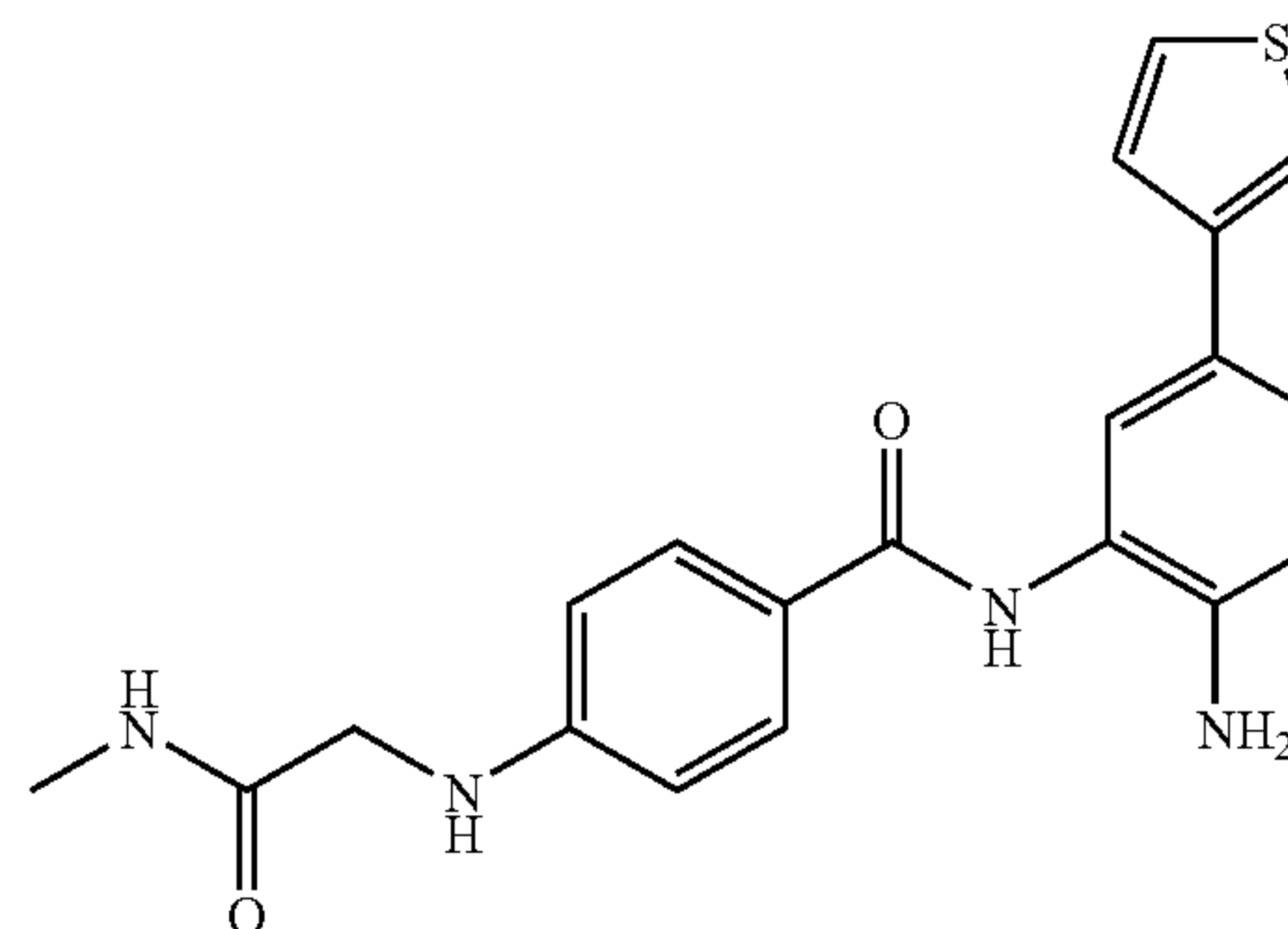
N-[2-amino-5-(3-thienyl)phenyl]-4-{[2-(methylamino)-2-oxoethyl]amino}benzamide
