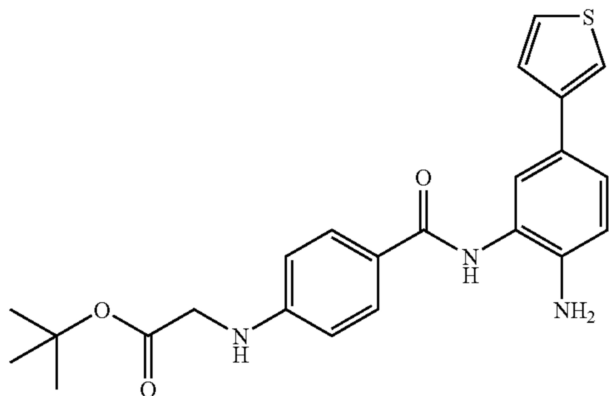
tert-Butyl[(4-{[2-amino-5-(3-thienyl)phenyl]amino}carbonyl)phenyl]amino]acetate
