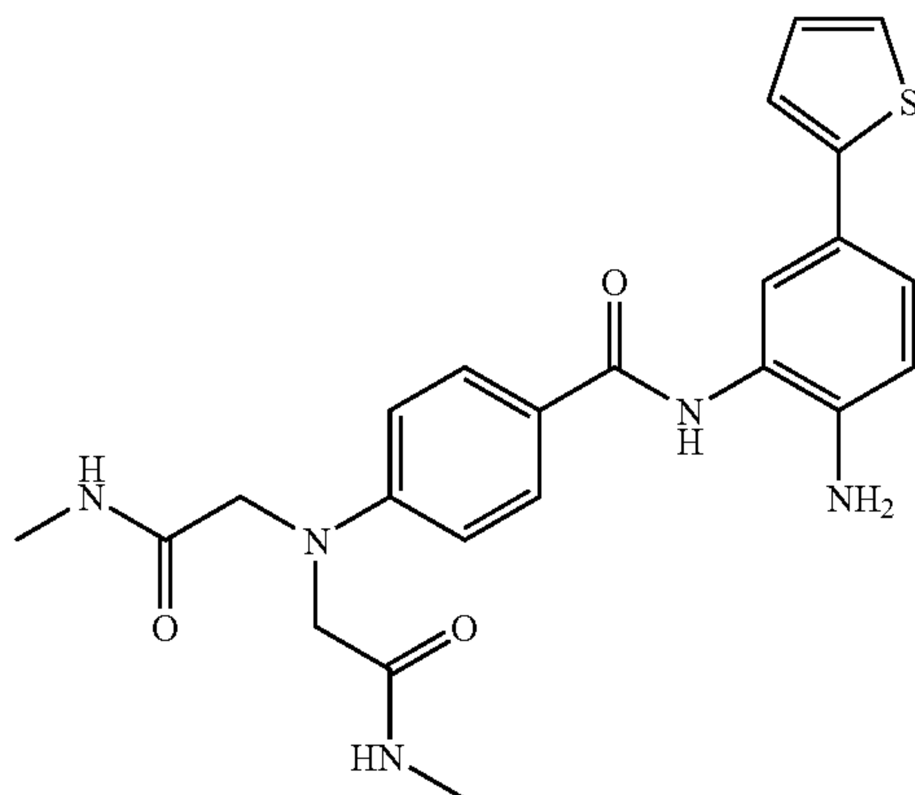
N-[2-amino-5-(2-thienyl)phenyl]-4-{bis[2-(methylamino)-2-oxoethyl]amino}benzamide
