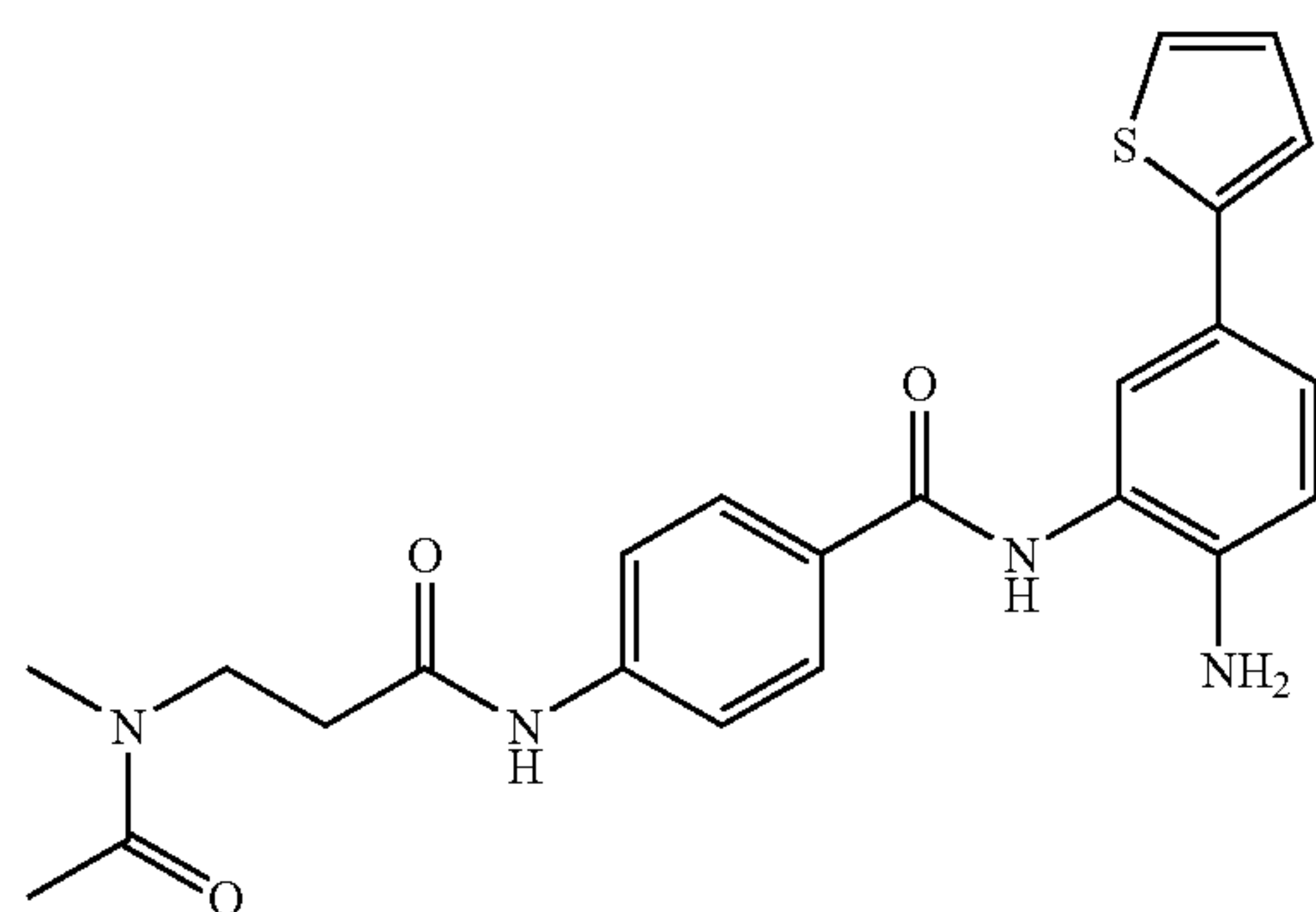
4-({3-[acetyl(methyl)aminol]propanoyl}amino)-N-[2-amino-5-(2-thienyl)phenyl]benzamide
