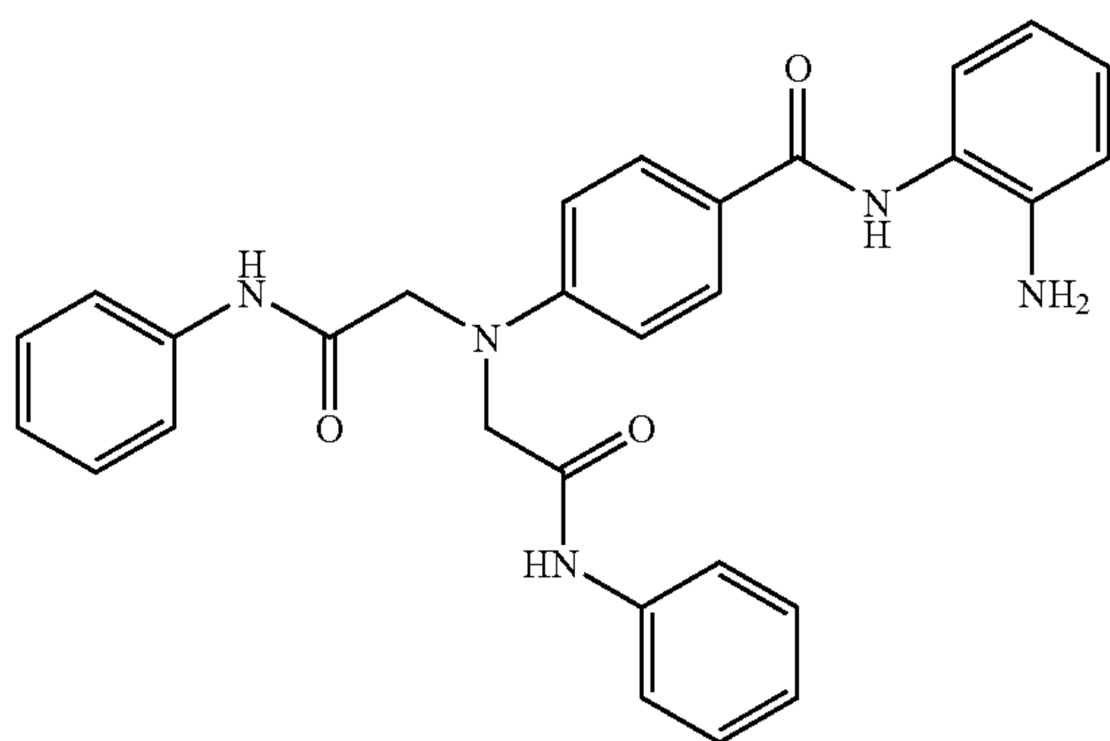
N-(2-aminophenyl)-4-[bis(2-anilino-2-oxoethyl) amino]benzamide
