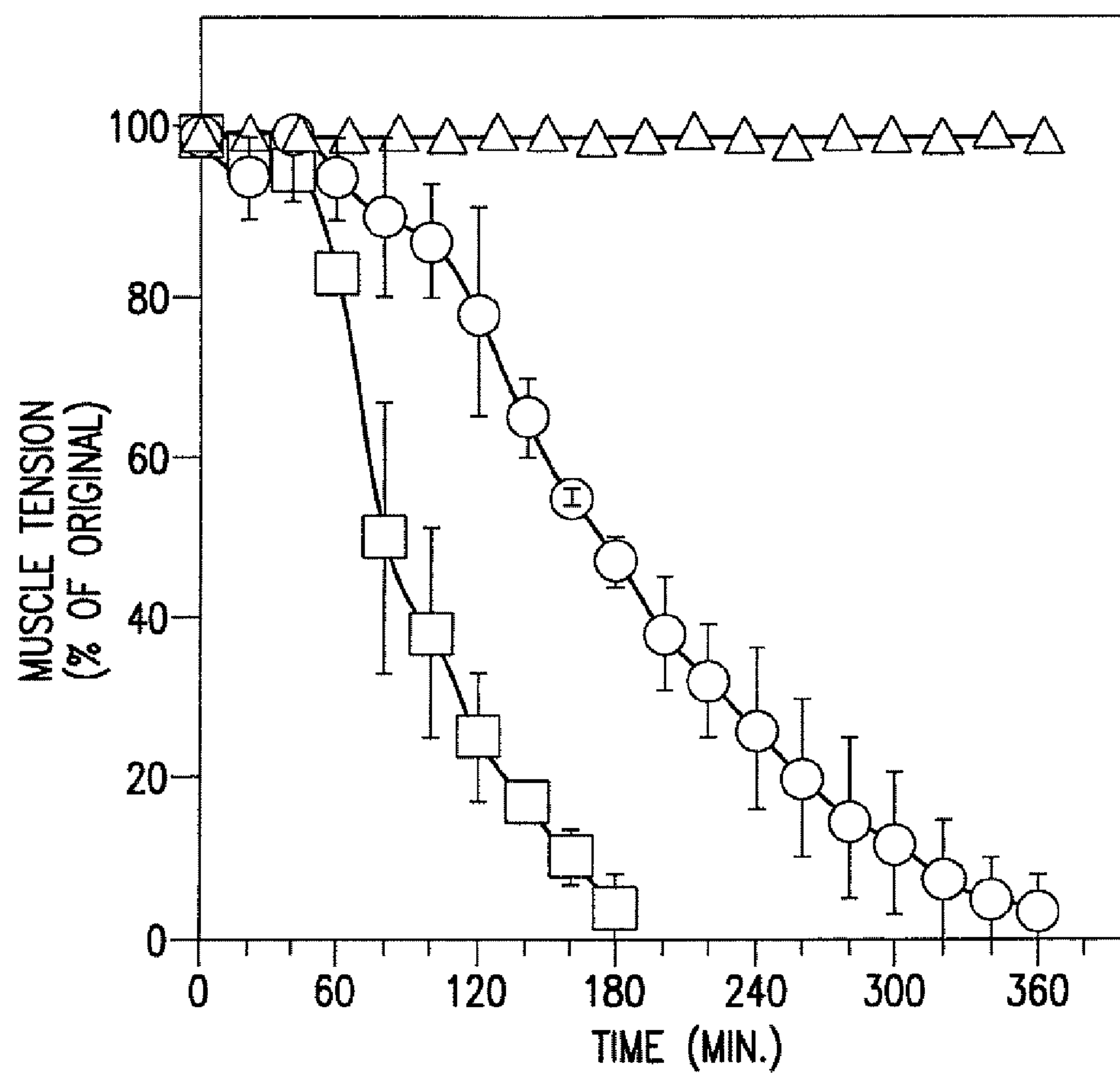
FIG.9
