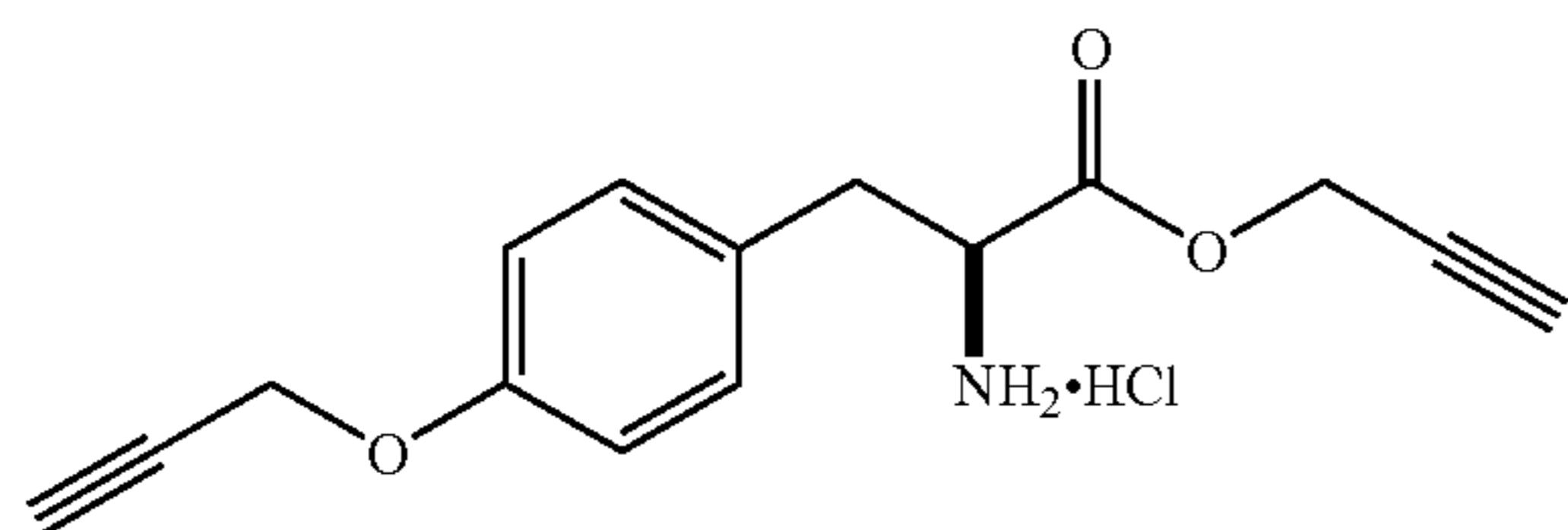
2-Amino-3-[4-(prop-2-ynoxy)phenyl]-propionic acid propargyl ester
