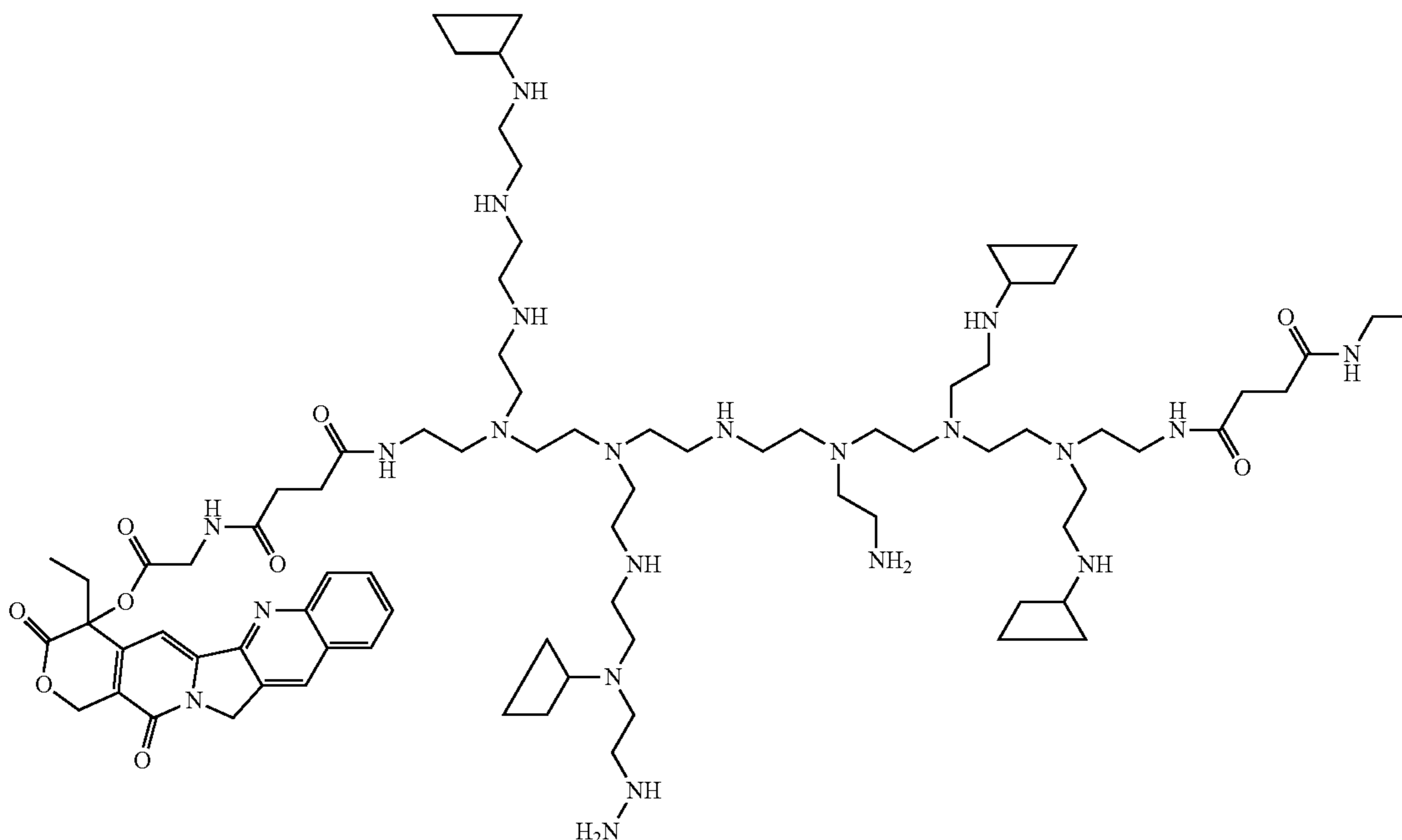
Scheme LI
