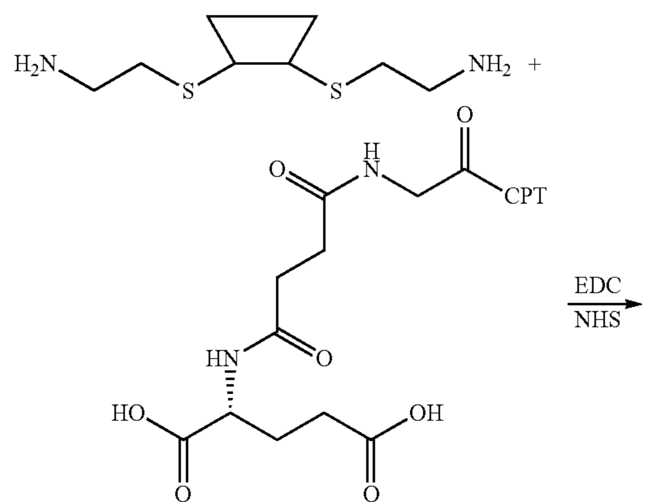
Scheme VI
