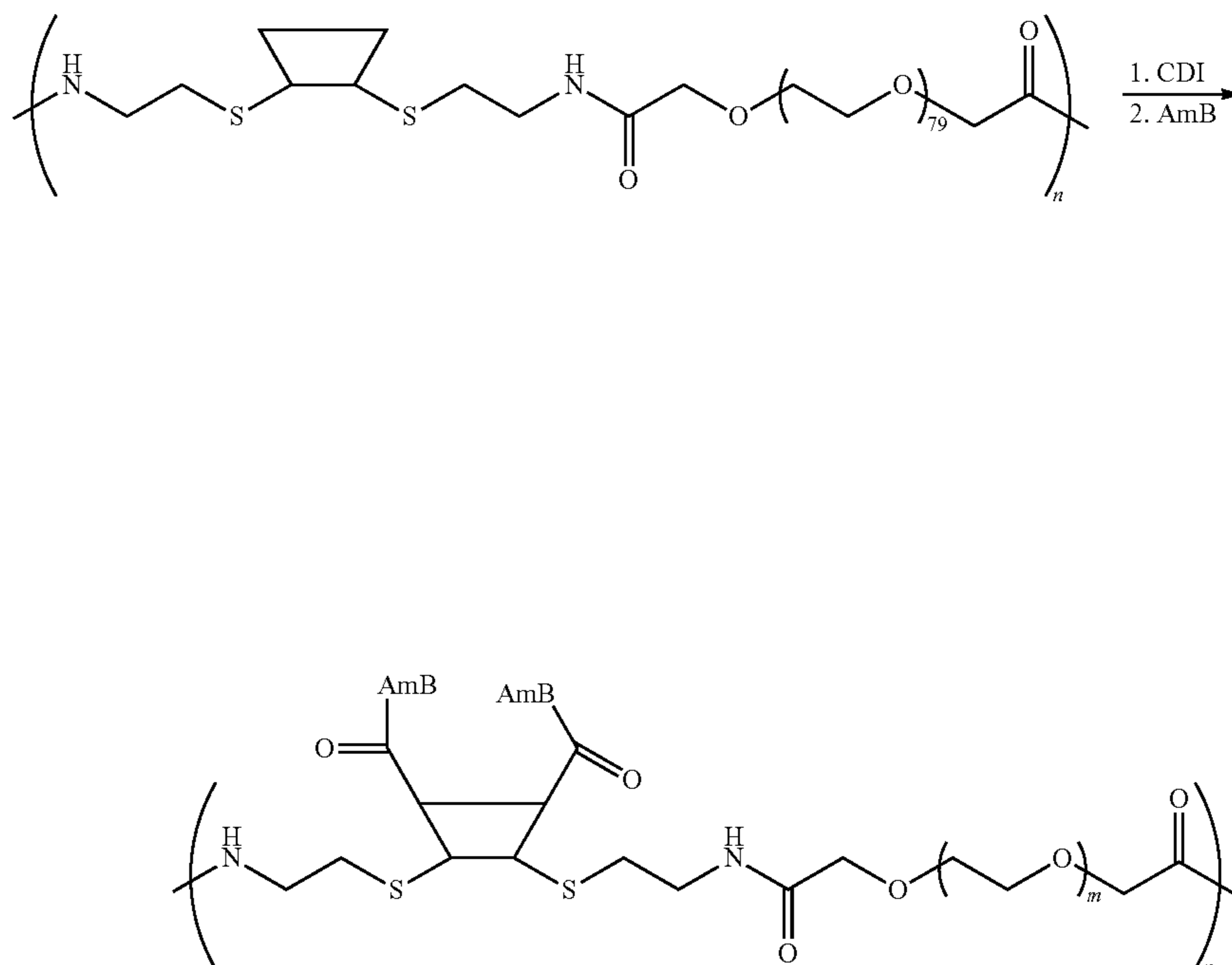
Scheme LII
