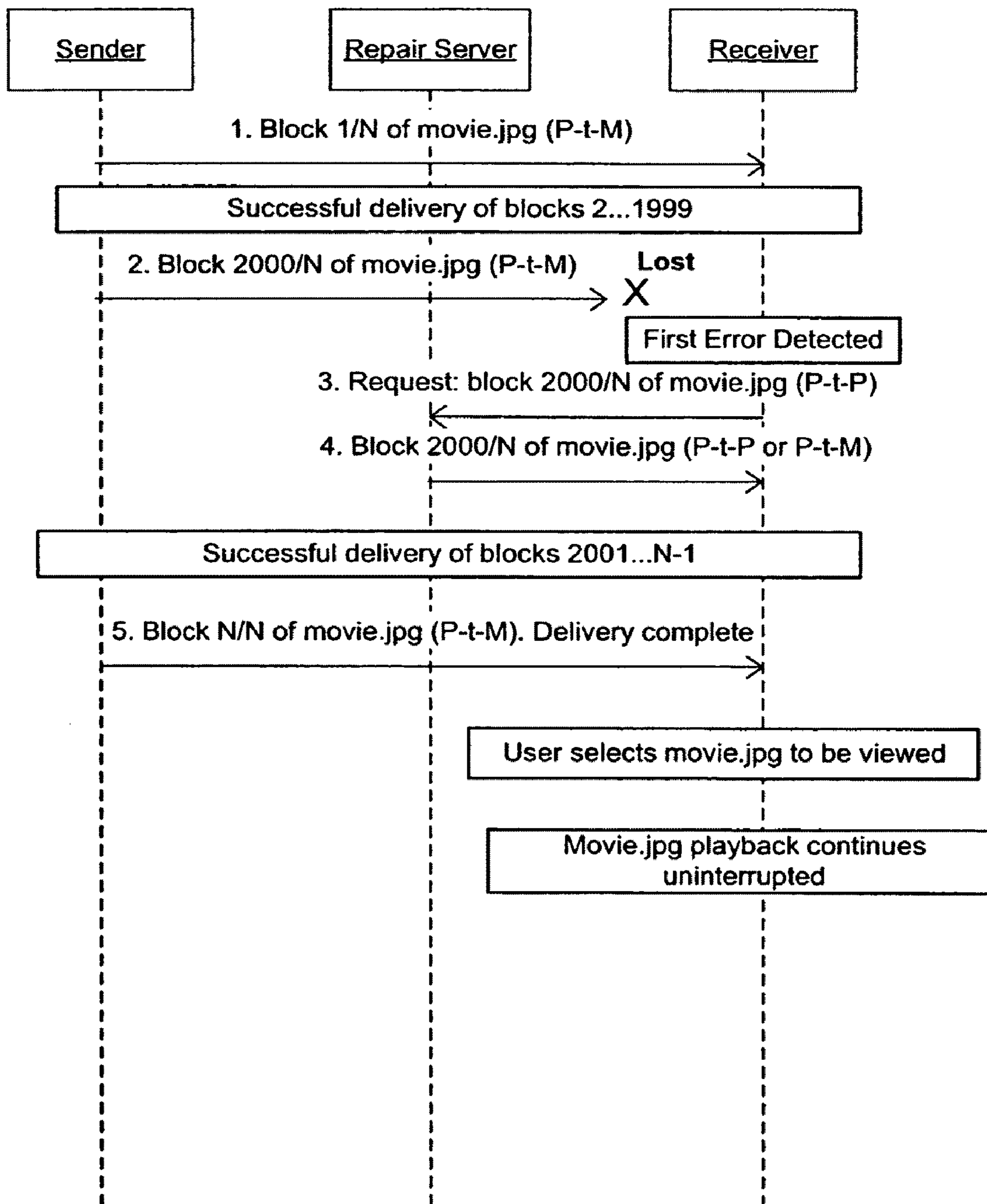
FIG. 12
