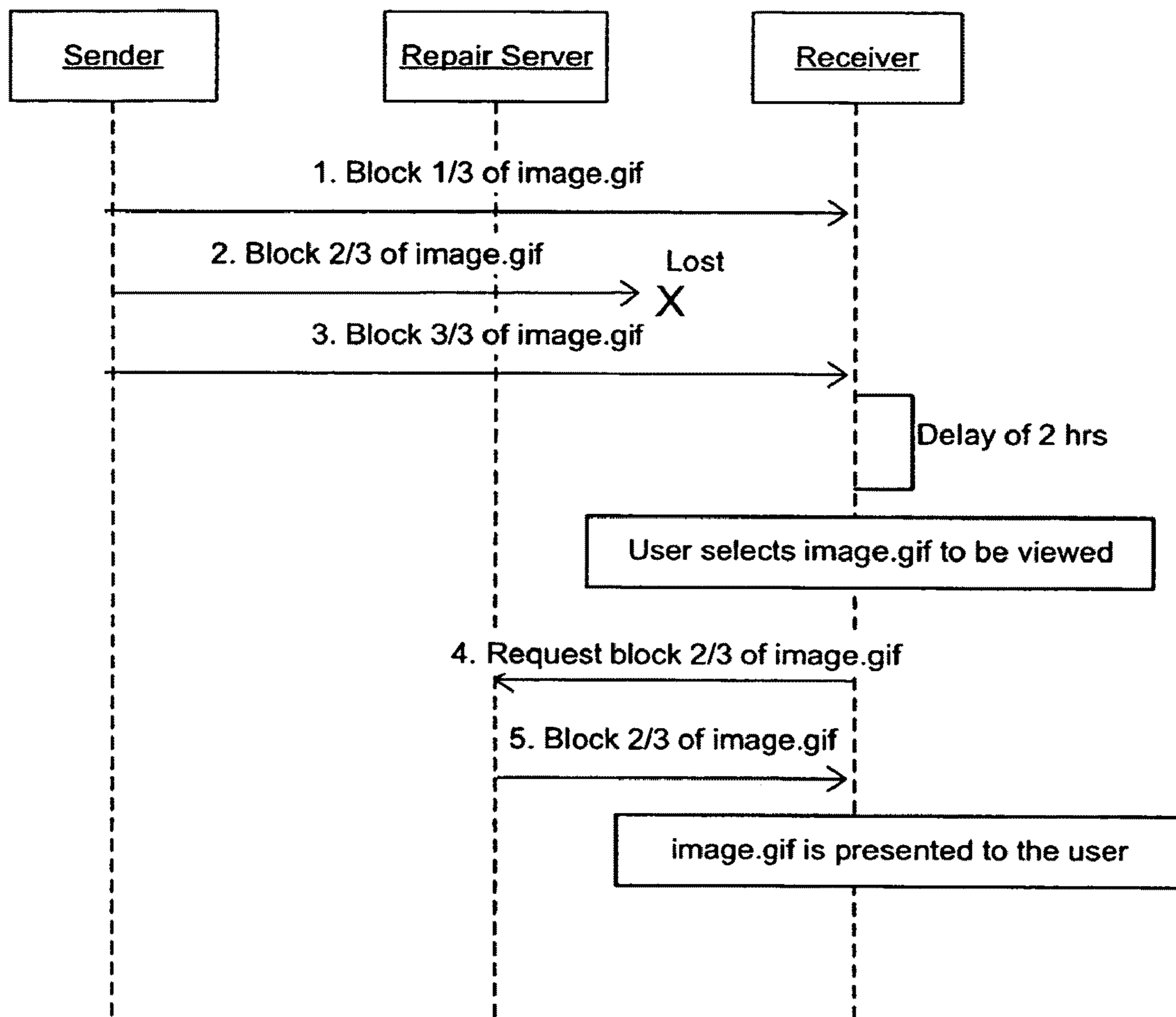
FIG. 10
