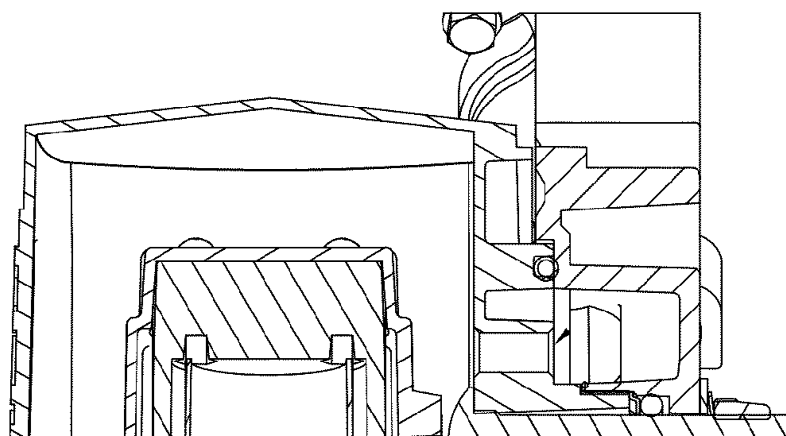
SECTION D-D
