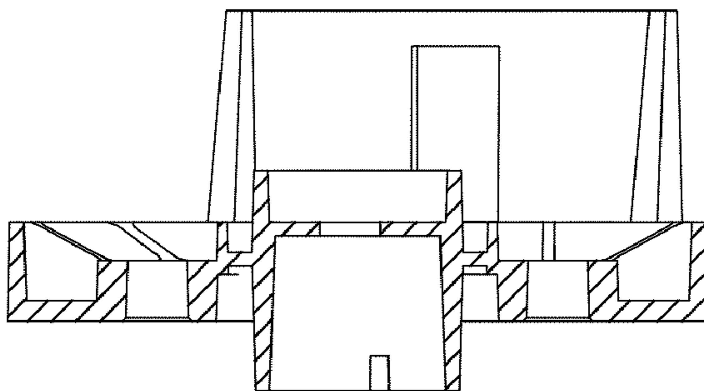
SECTION C-C Fig. 6H
