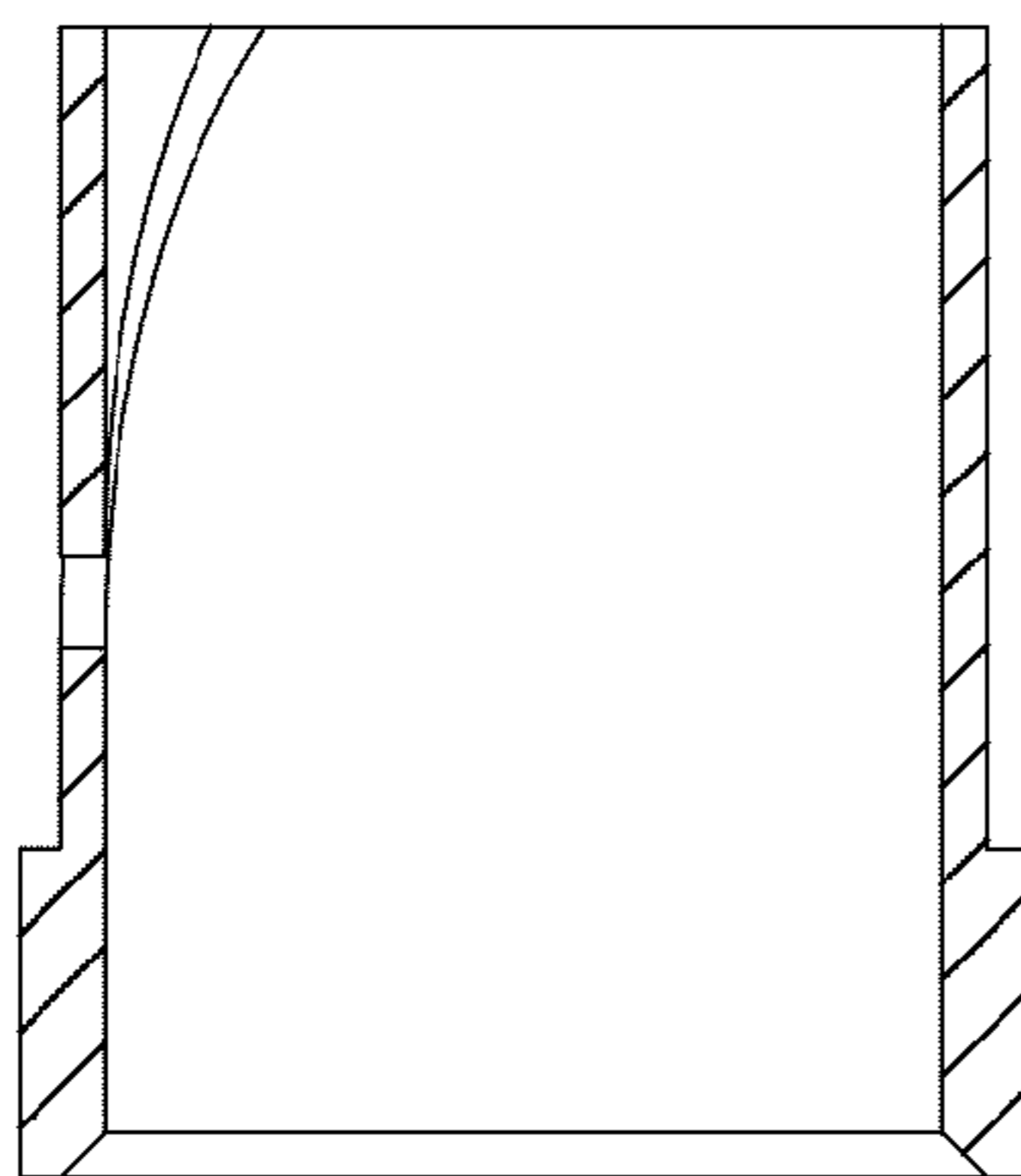
SECTION A-A Fig. 9D
