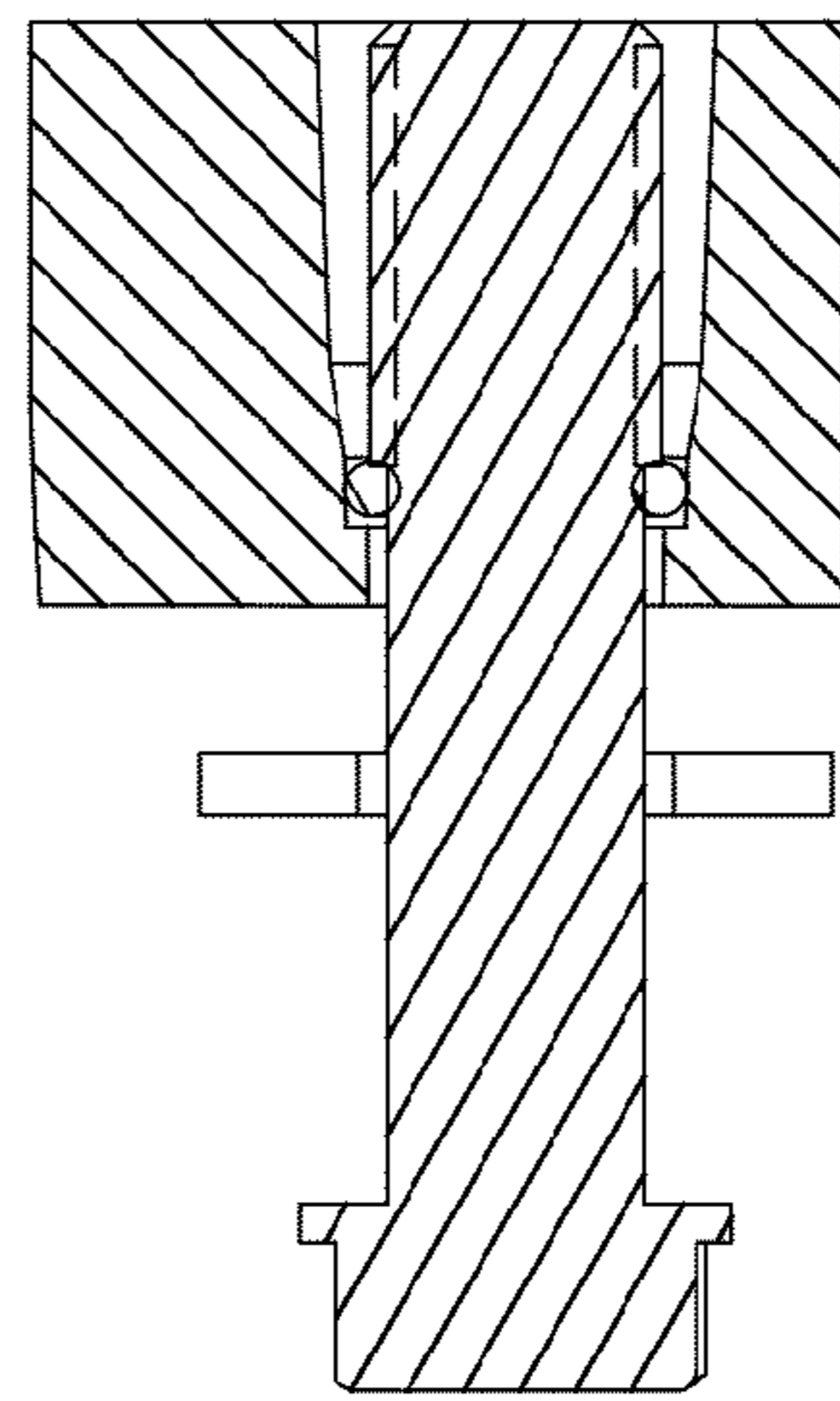
SECTION A-A
