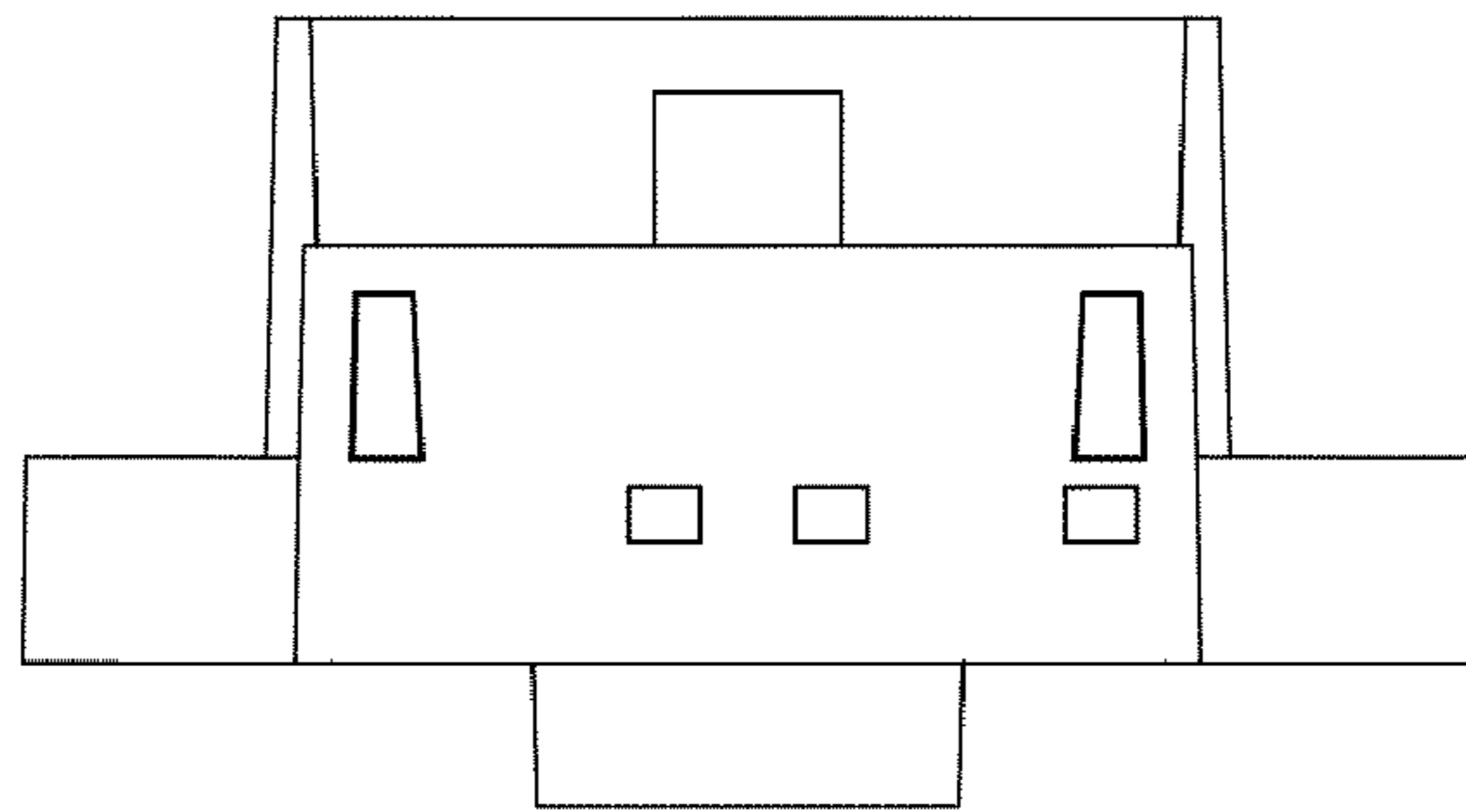
VIEW E-E Fig. 6F
