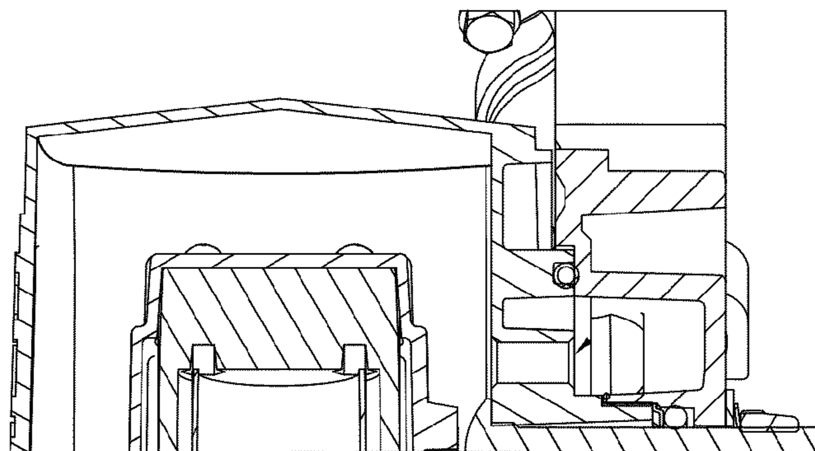
SECTION D-D
