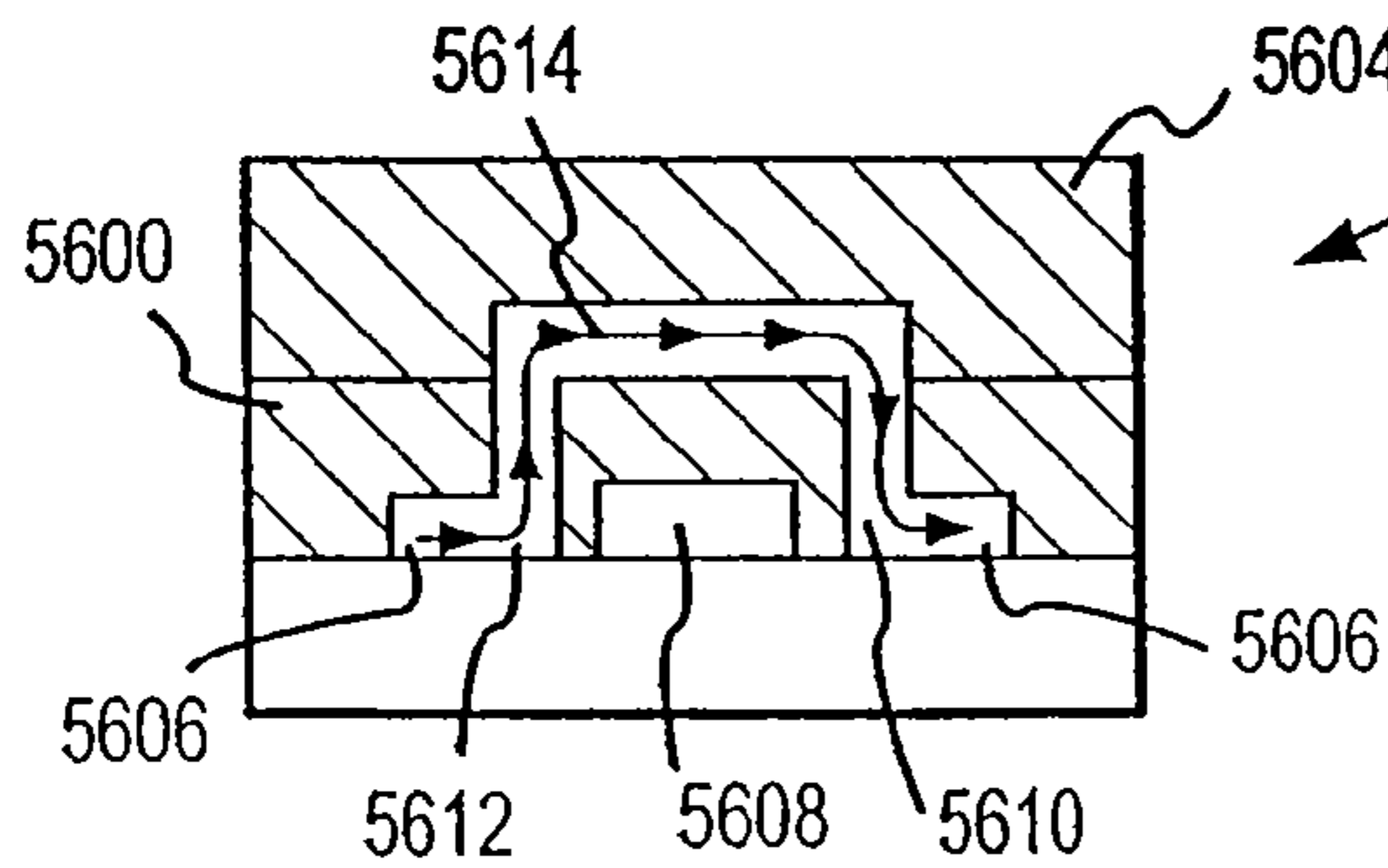
FIG. 52C
