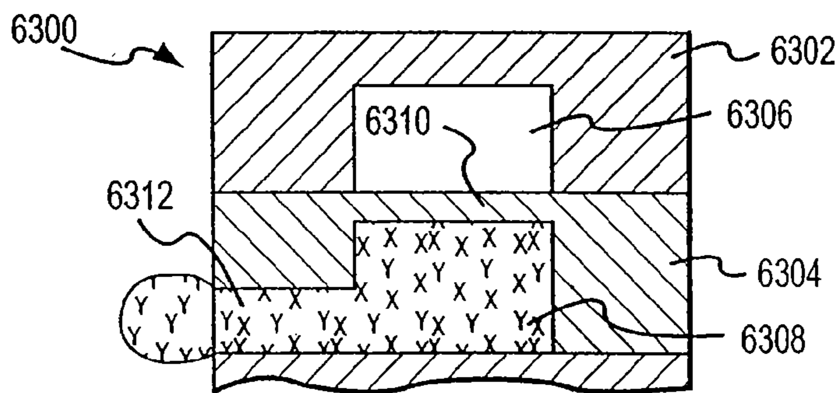
FIG. 58C
