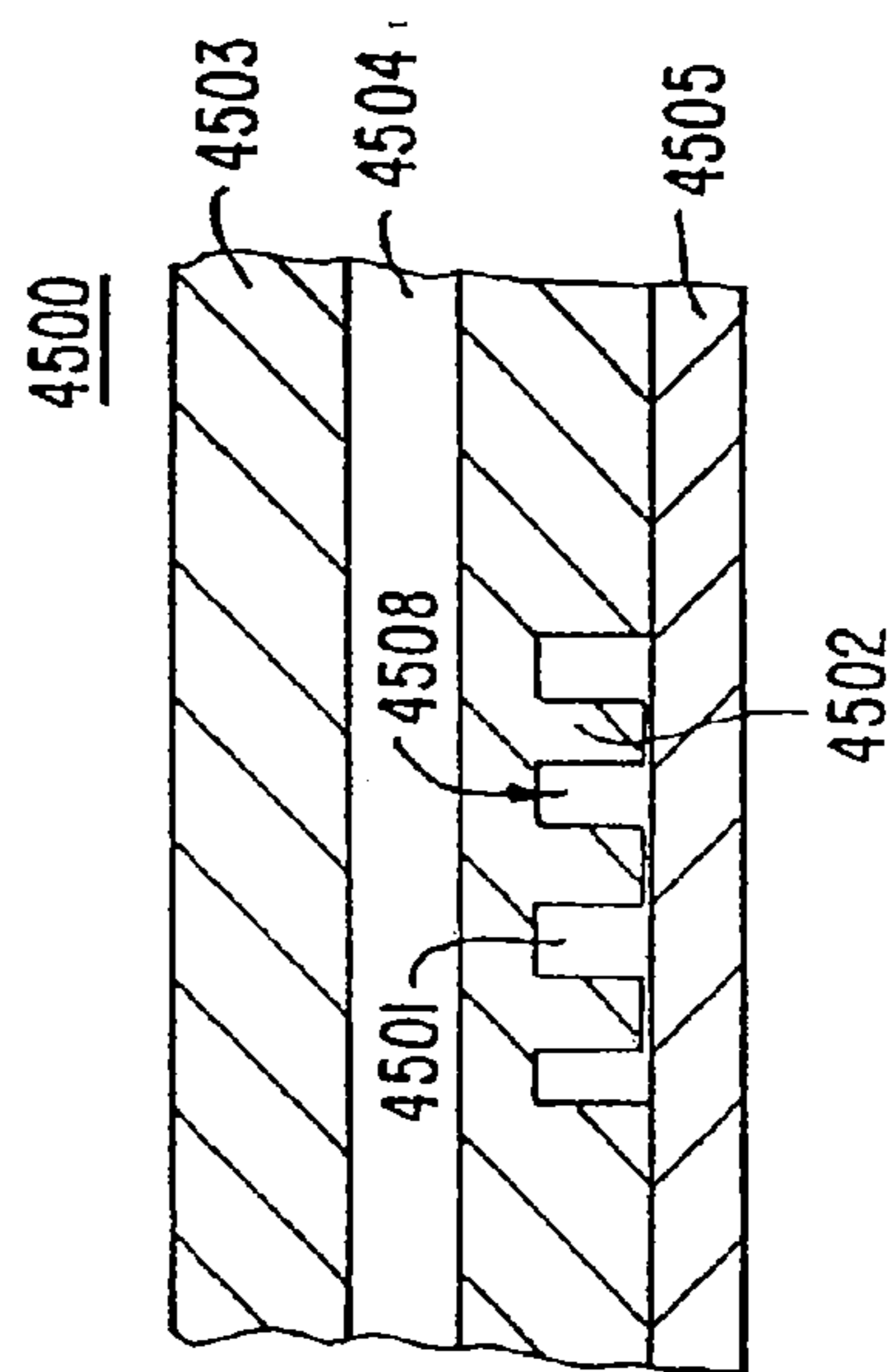
FIG. 45B.
