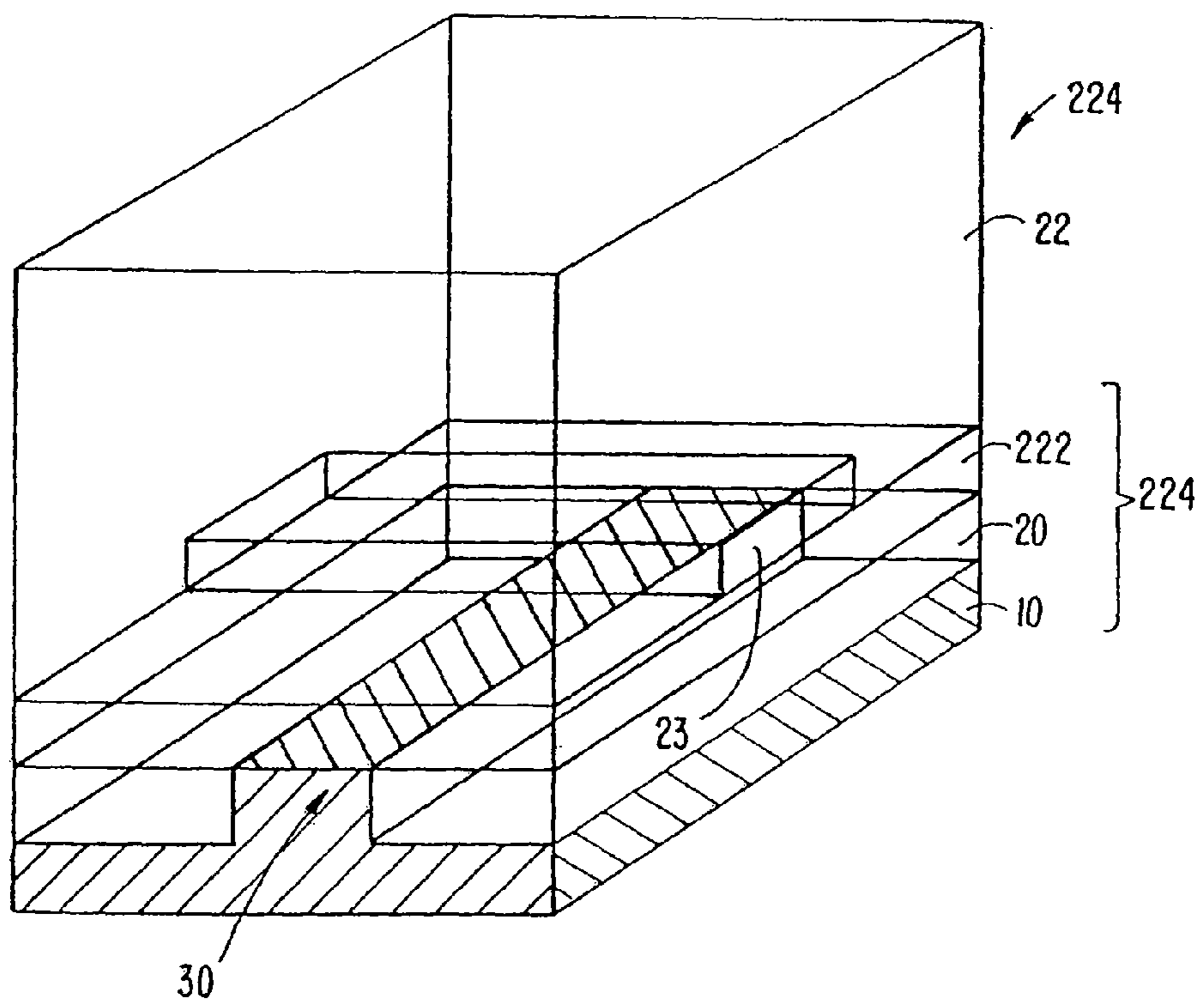
FIG. 7G.
