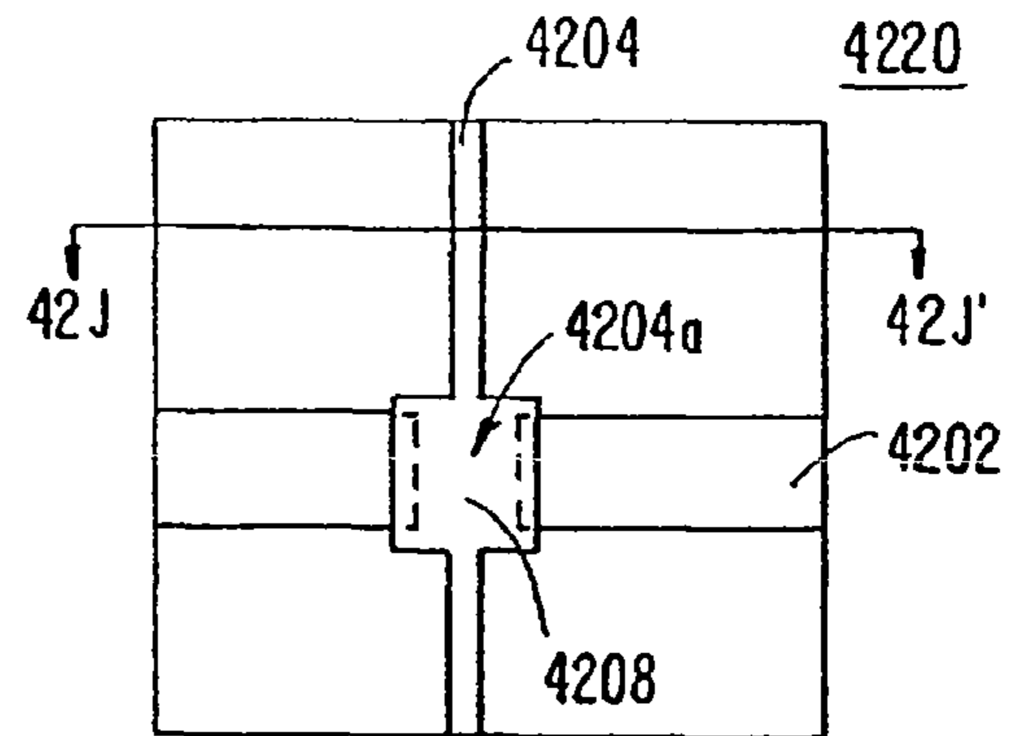
FIG. 42I.
