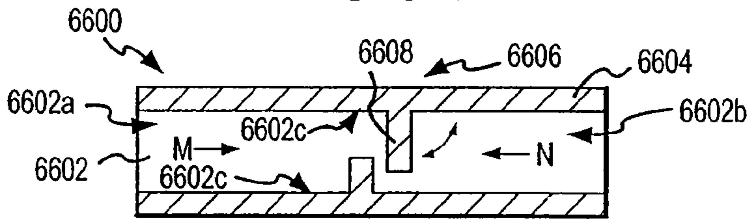
FIG. 61B
