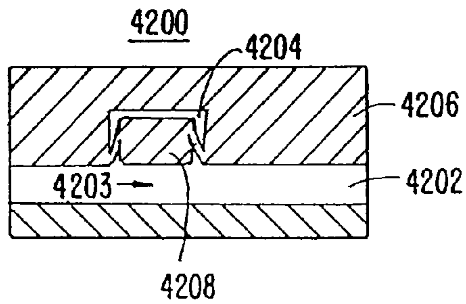
FIG. 42C.
