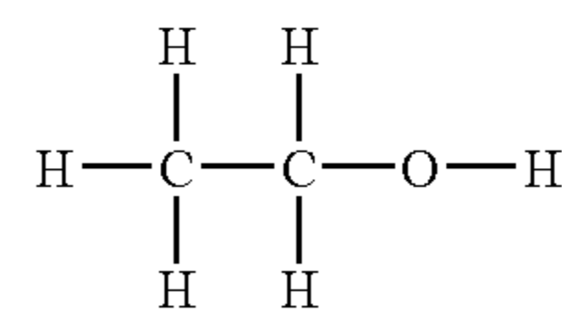
ETHANOL C 2 H 6 O
