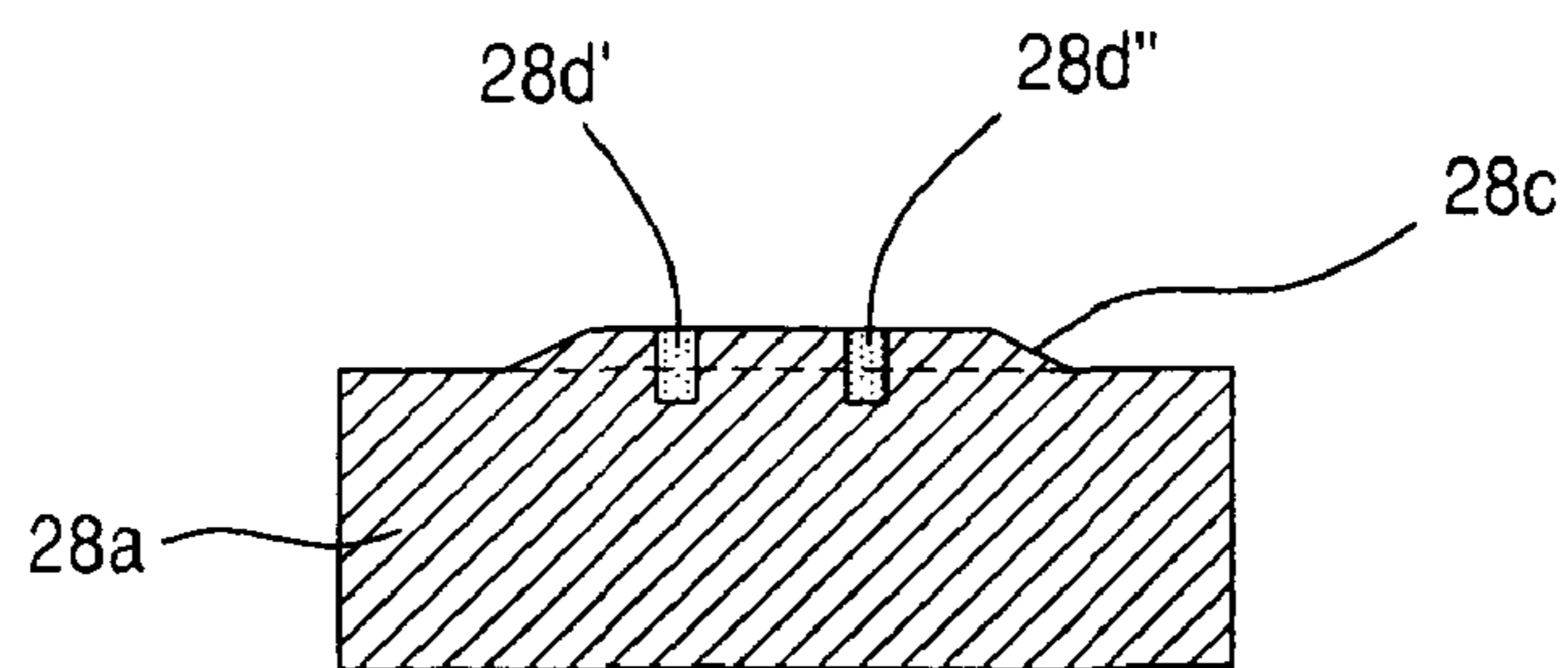
SECTION A-A
