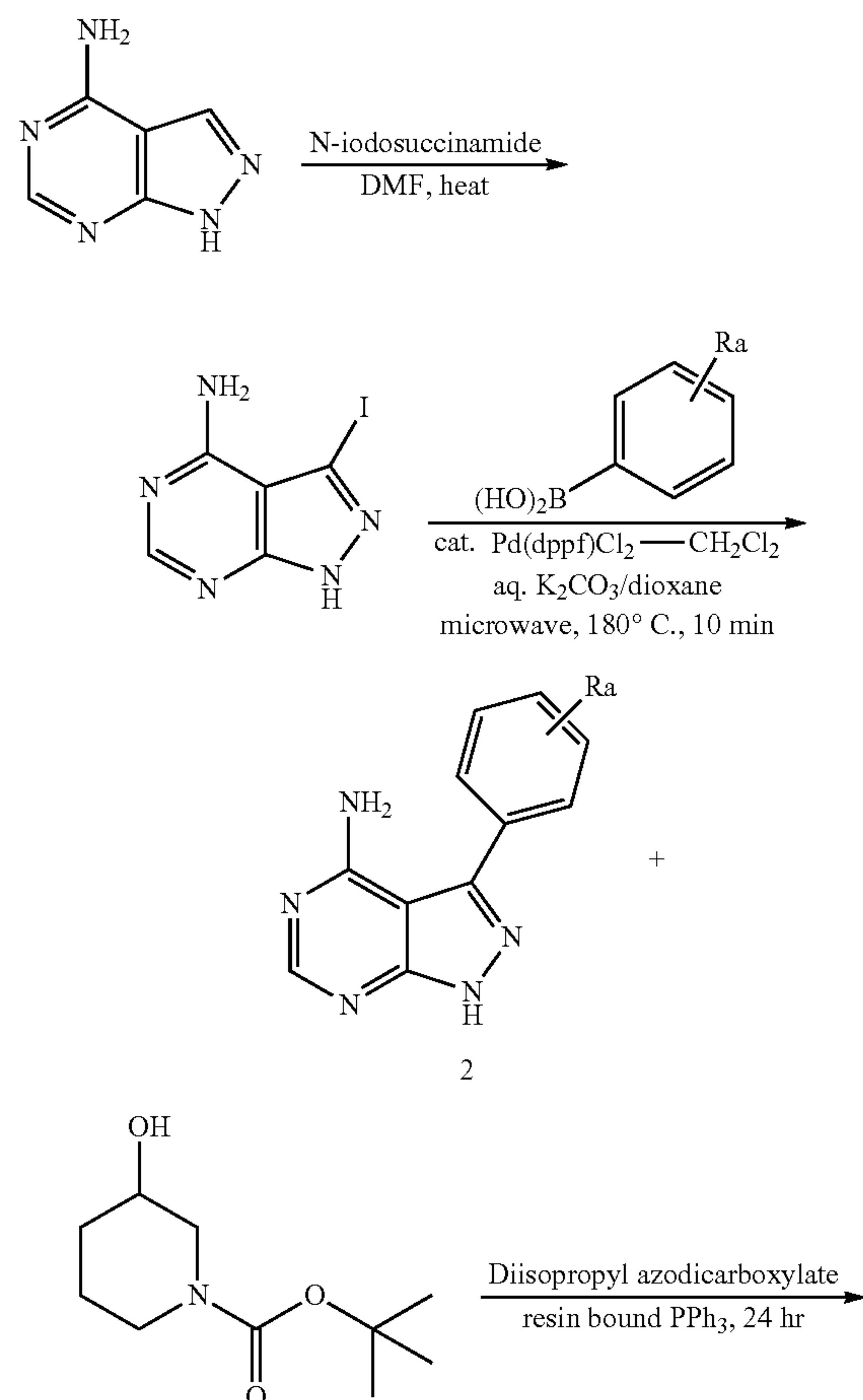
Scheme I.
