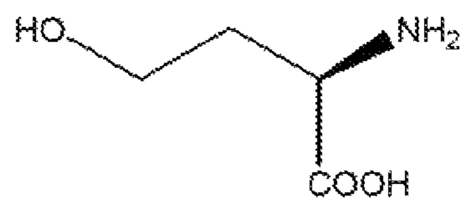
D-homoserine
