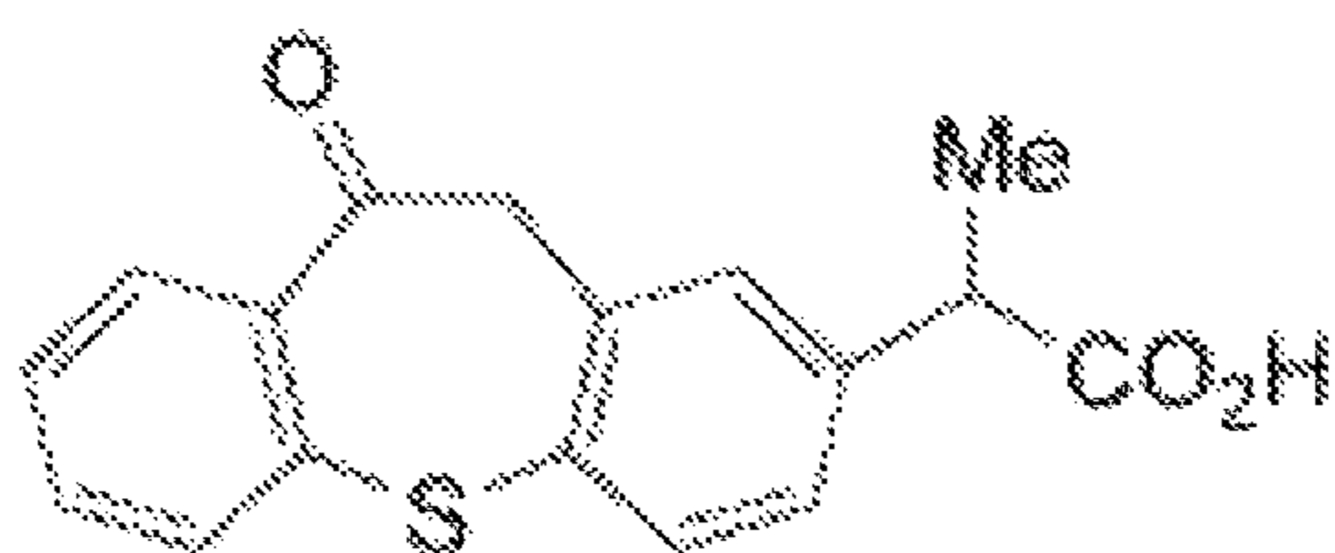
Zaltoprofen
