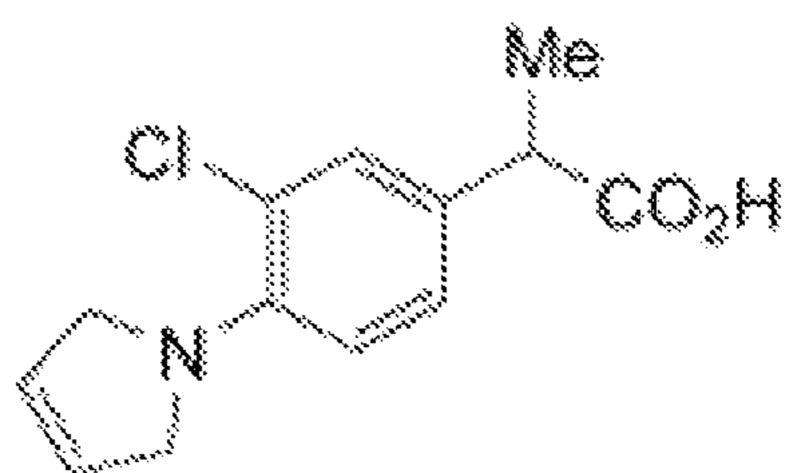
Pirprofen
