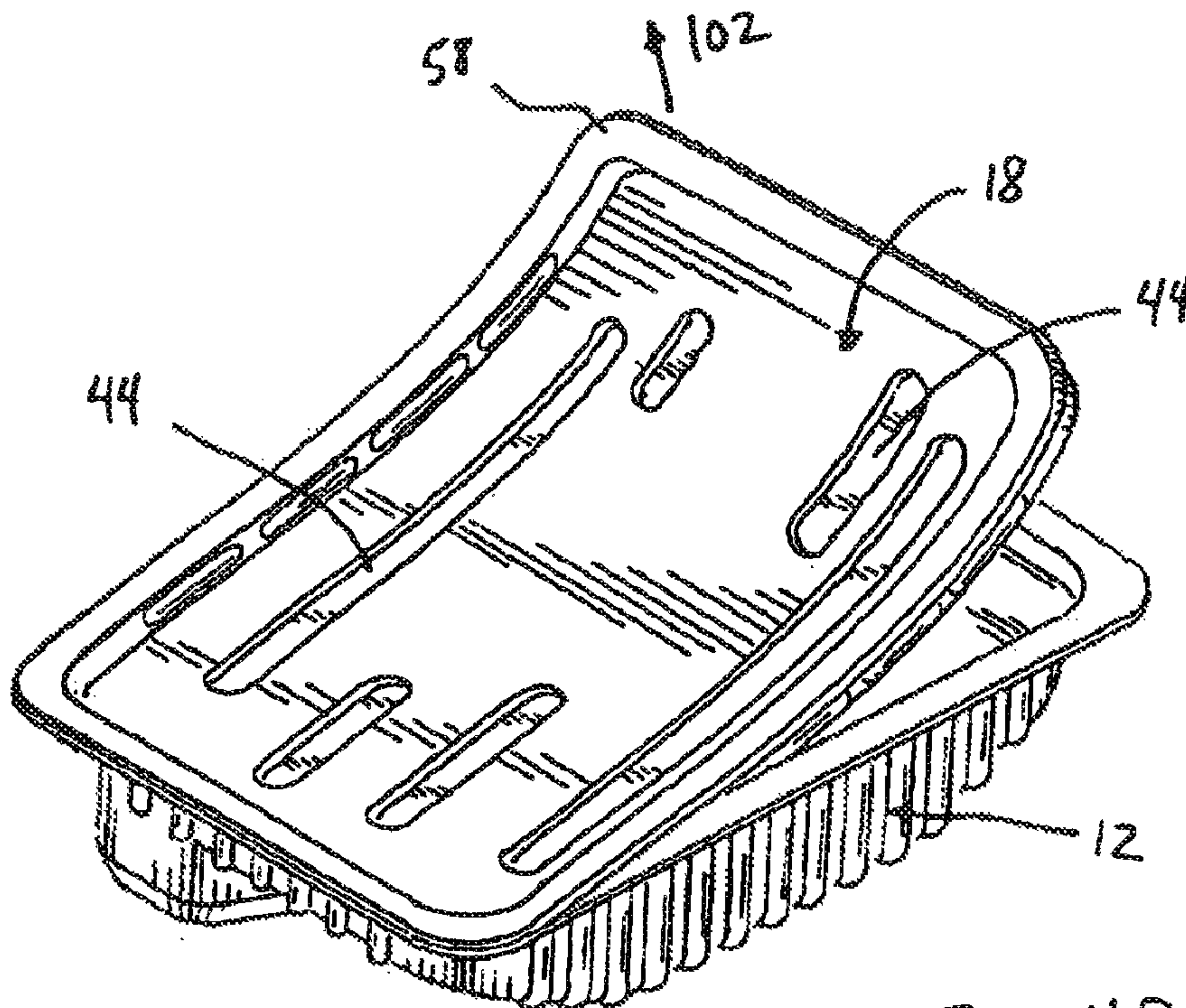
FIG. 14B
