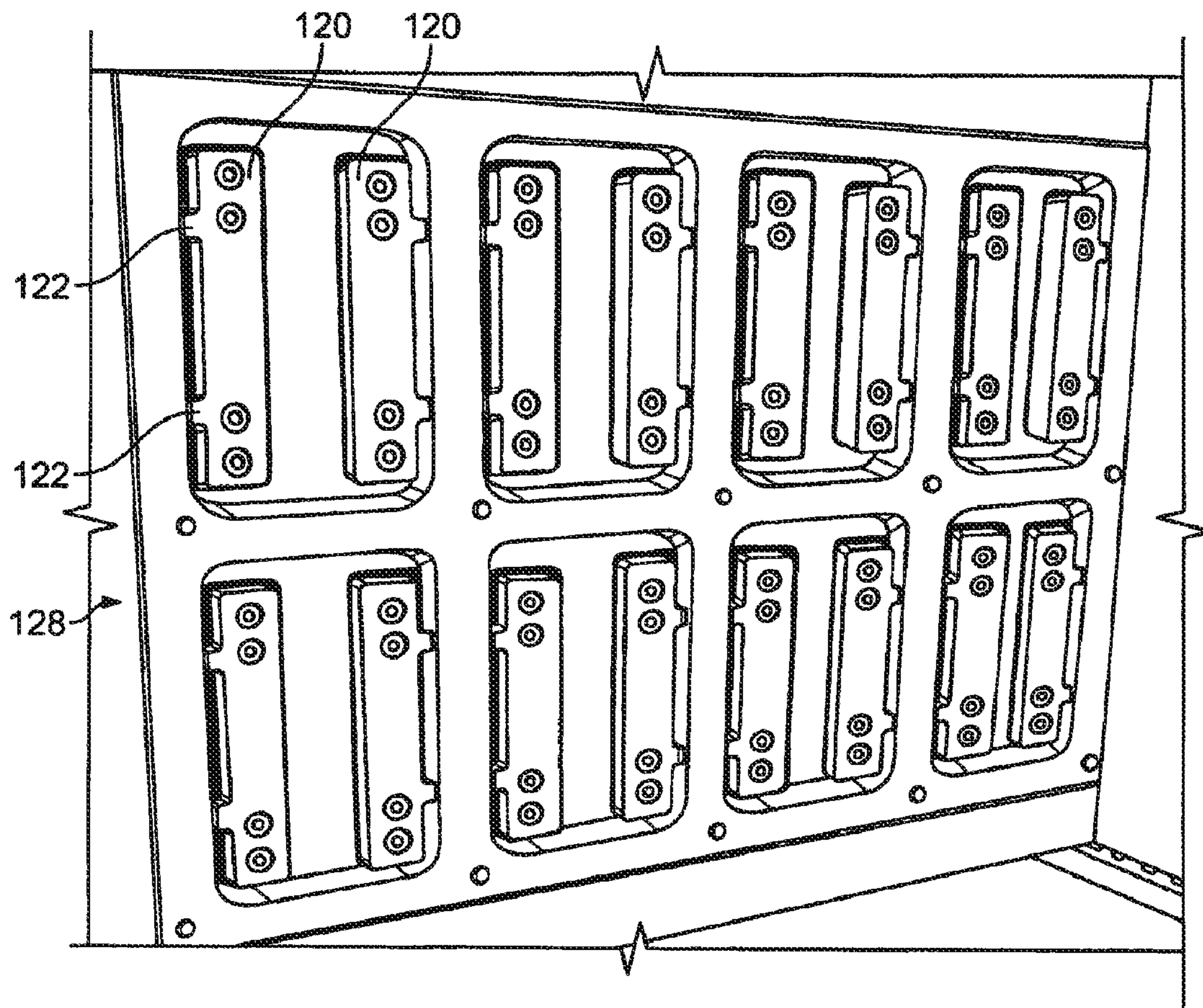
FIG. 21
