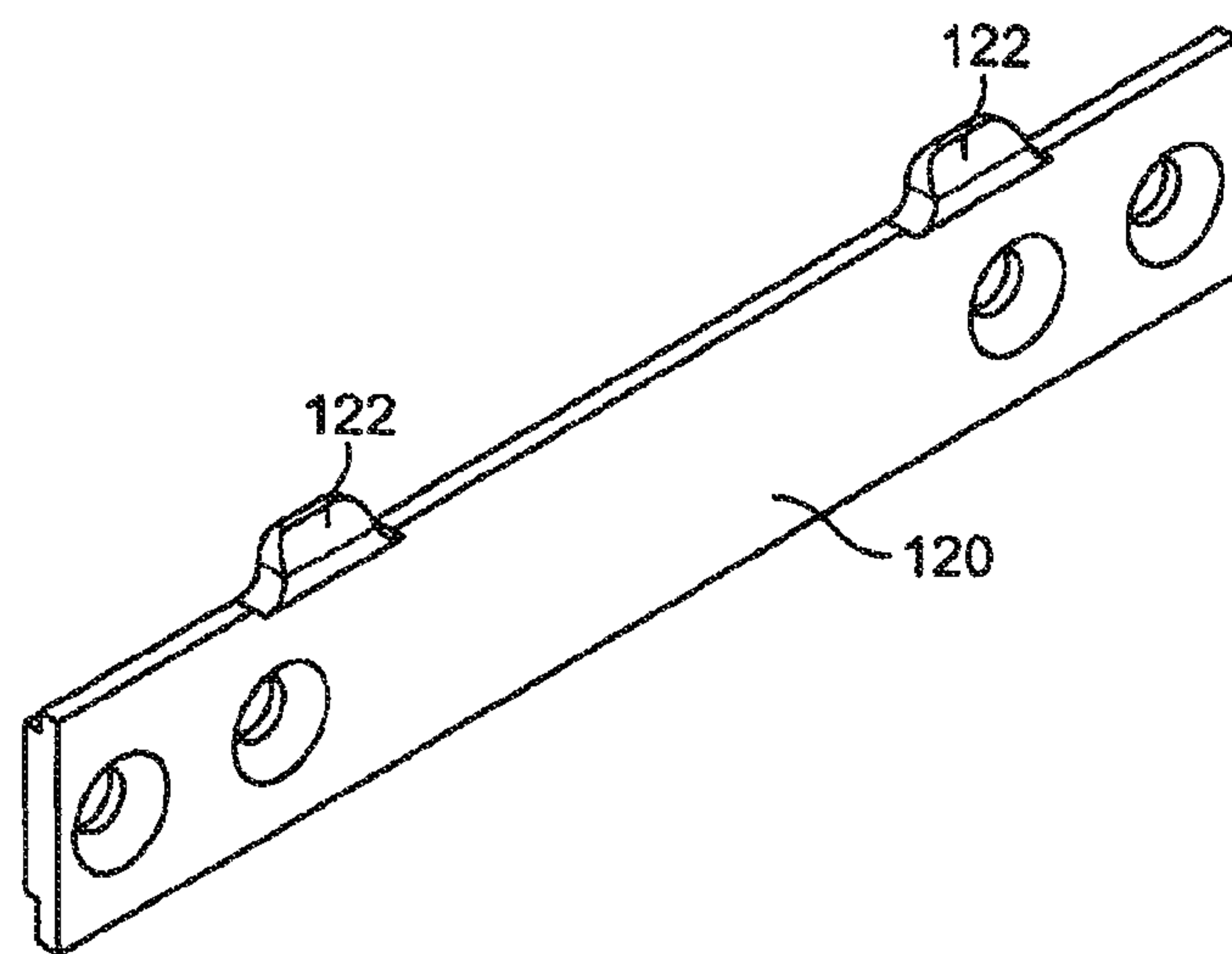
FIG. 23
