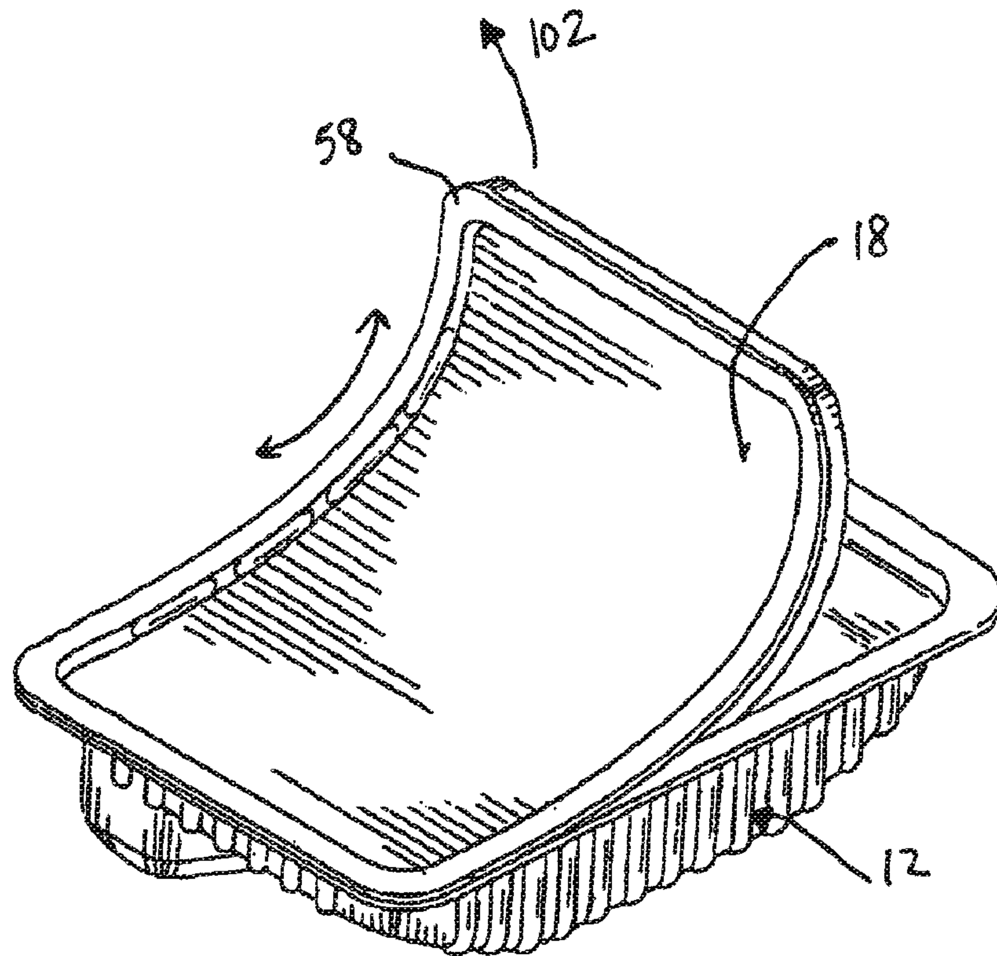
FIG. 14A
