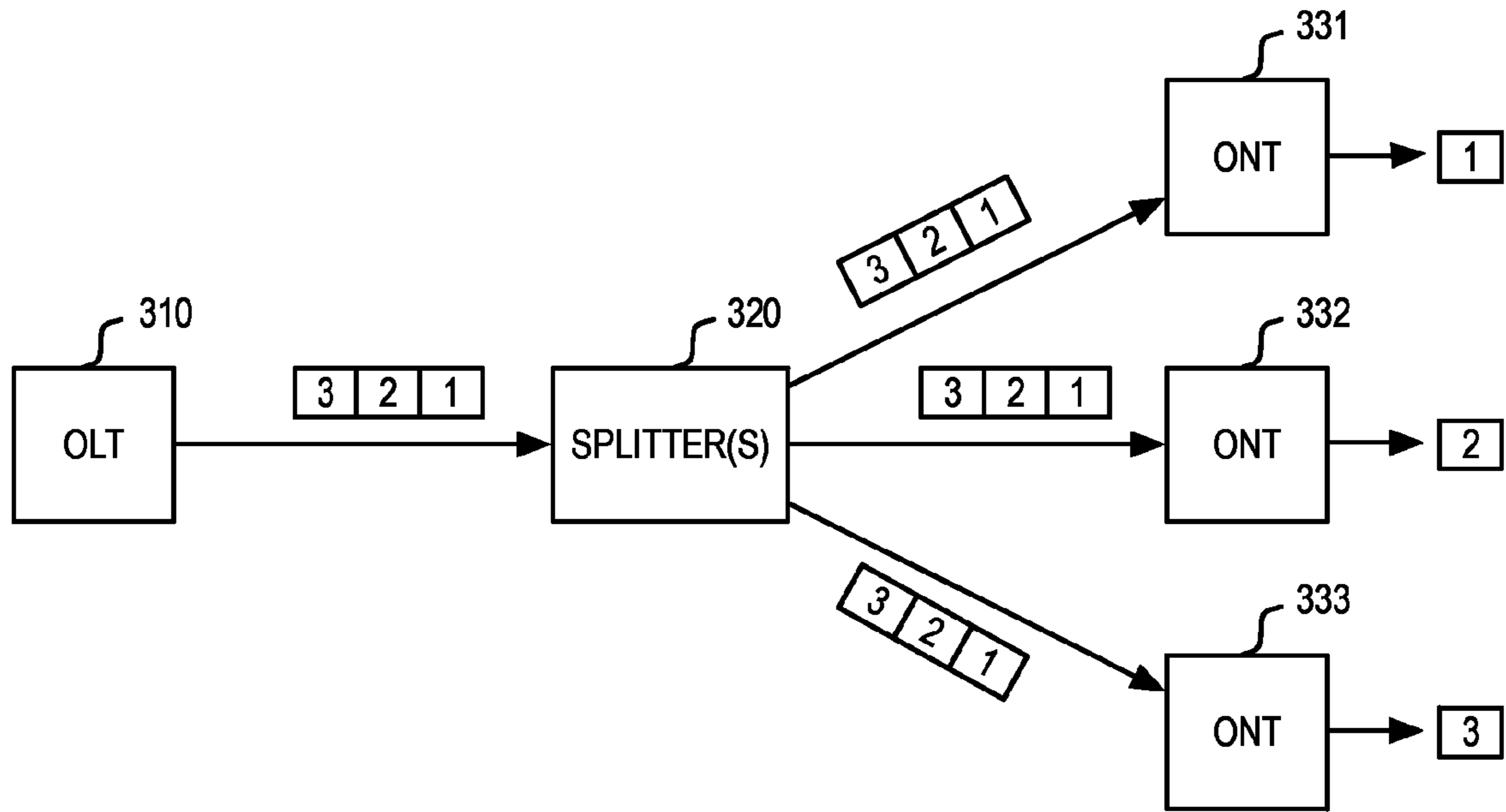
FIG. 3A
