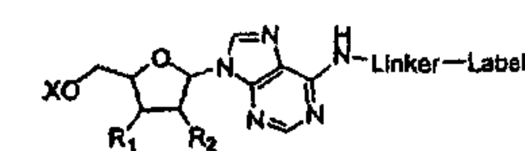
Adenosine N6-linker
