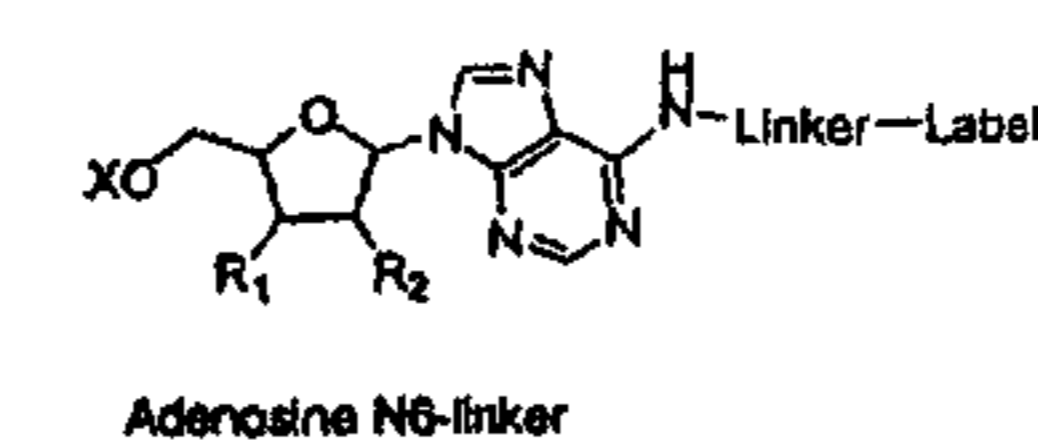
Adenosine N6-linker
