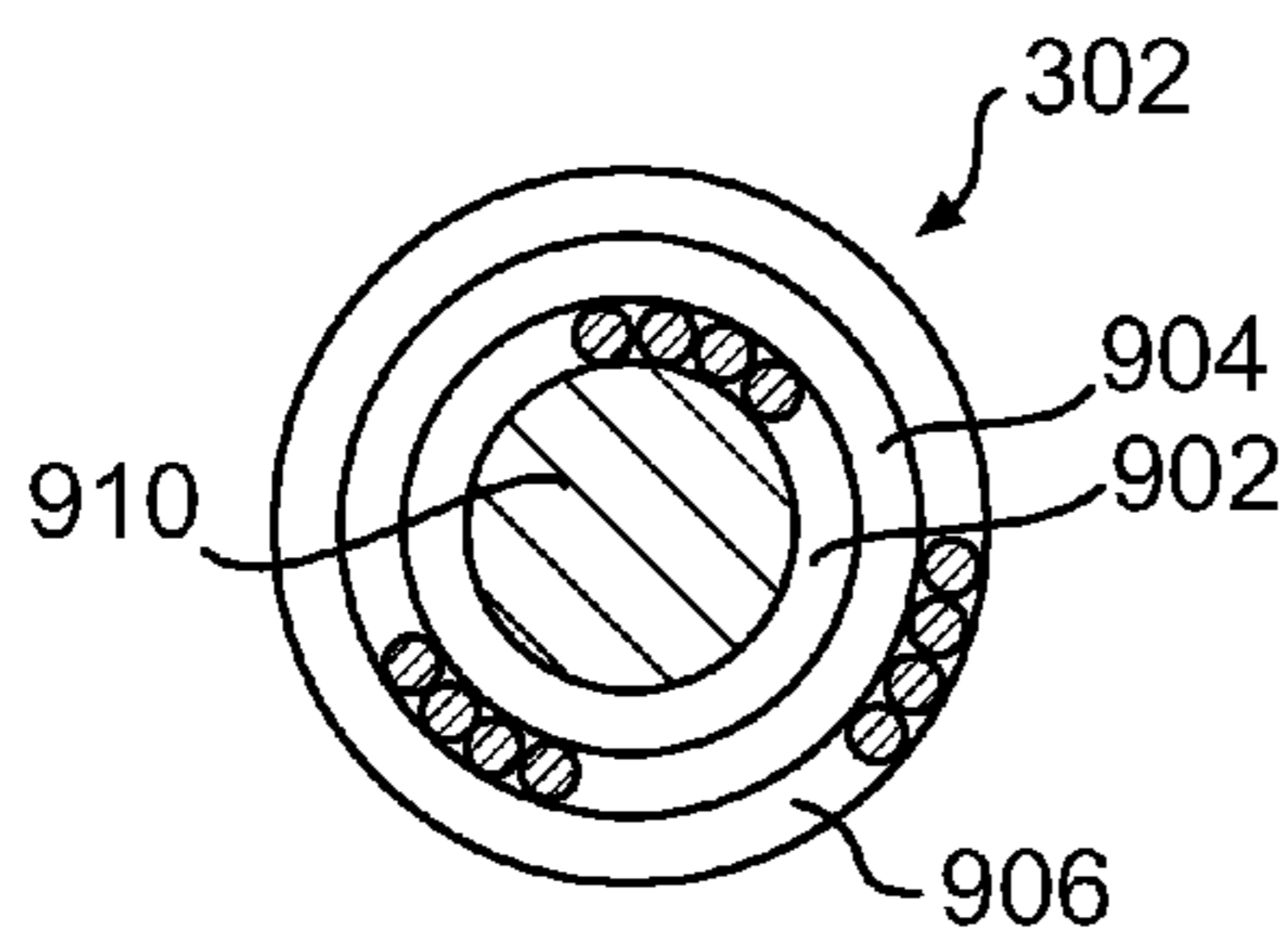
SECTION A-A FIG. 9B
