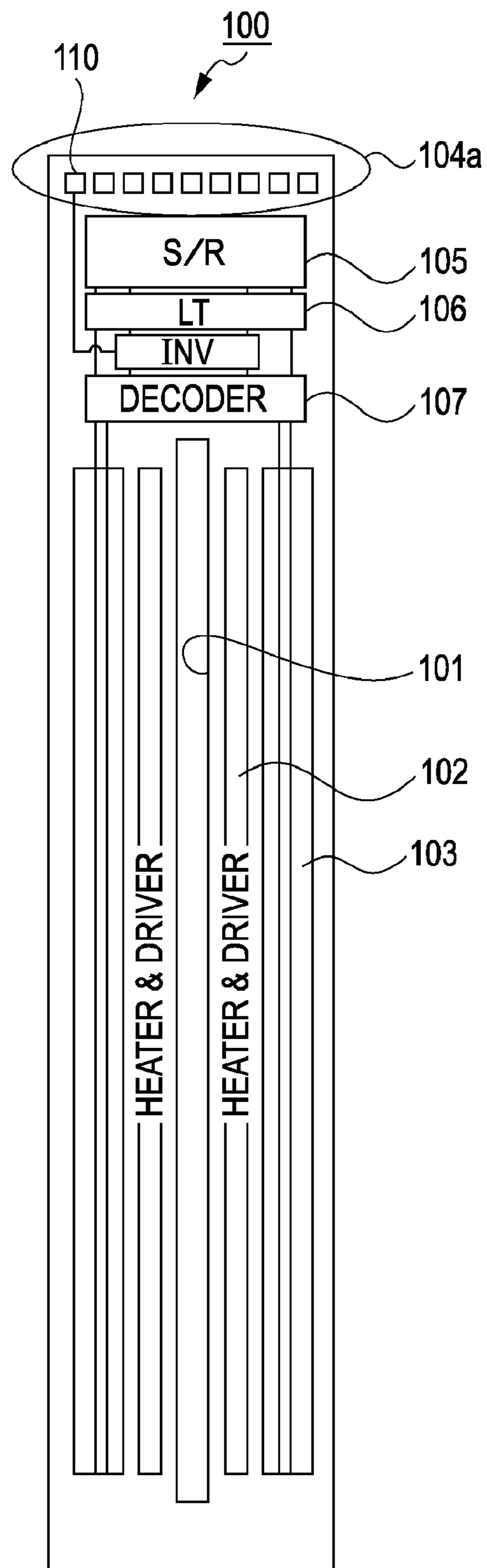
FIG. 5B
