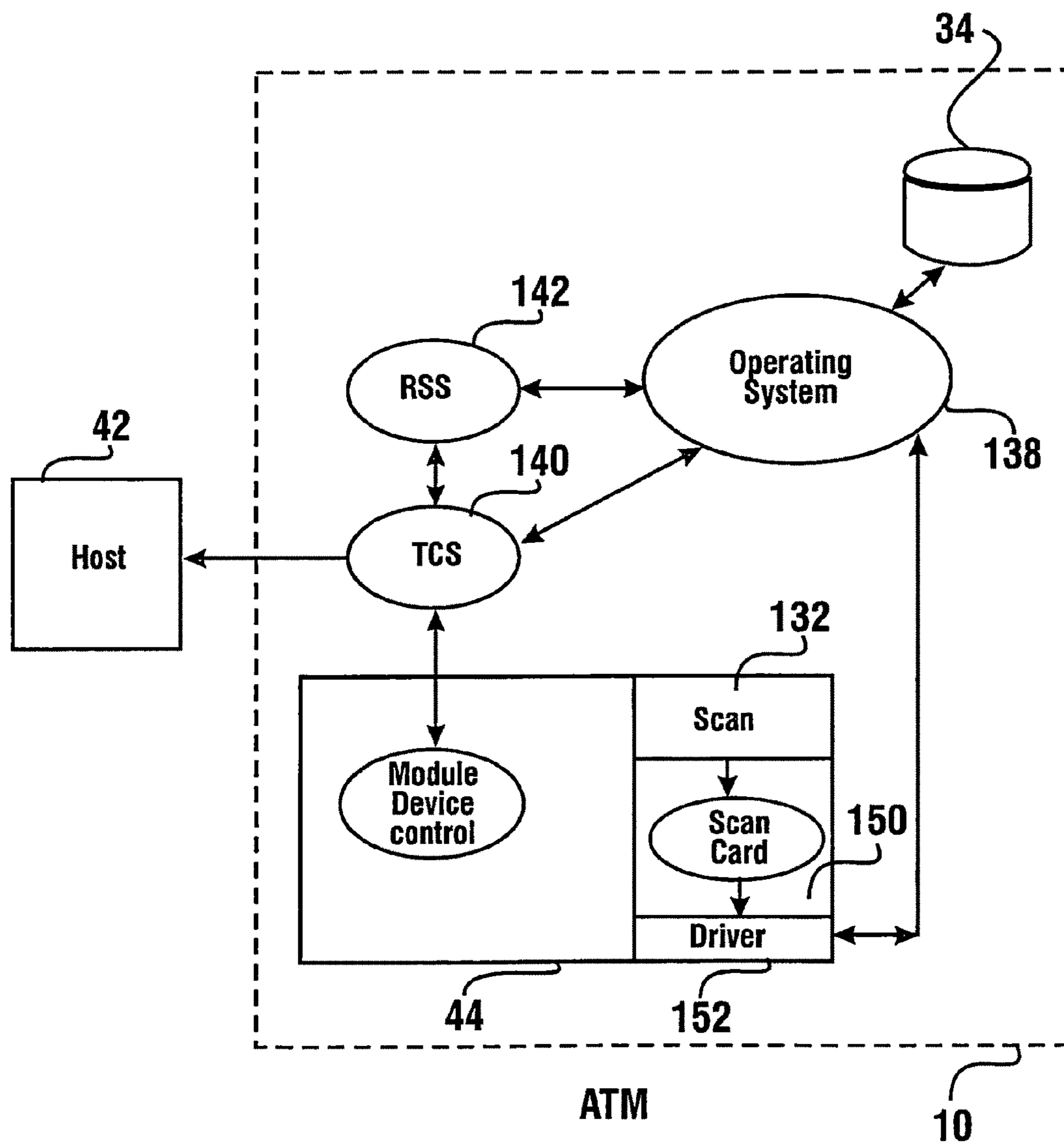
FIG. 8
