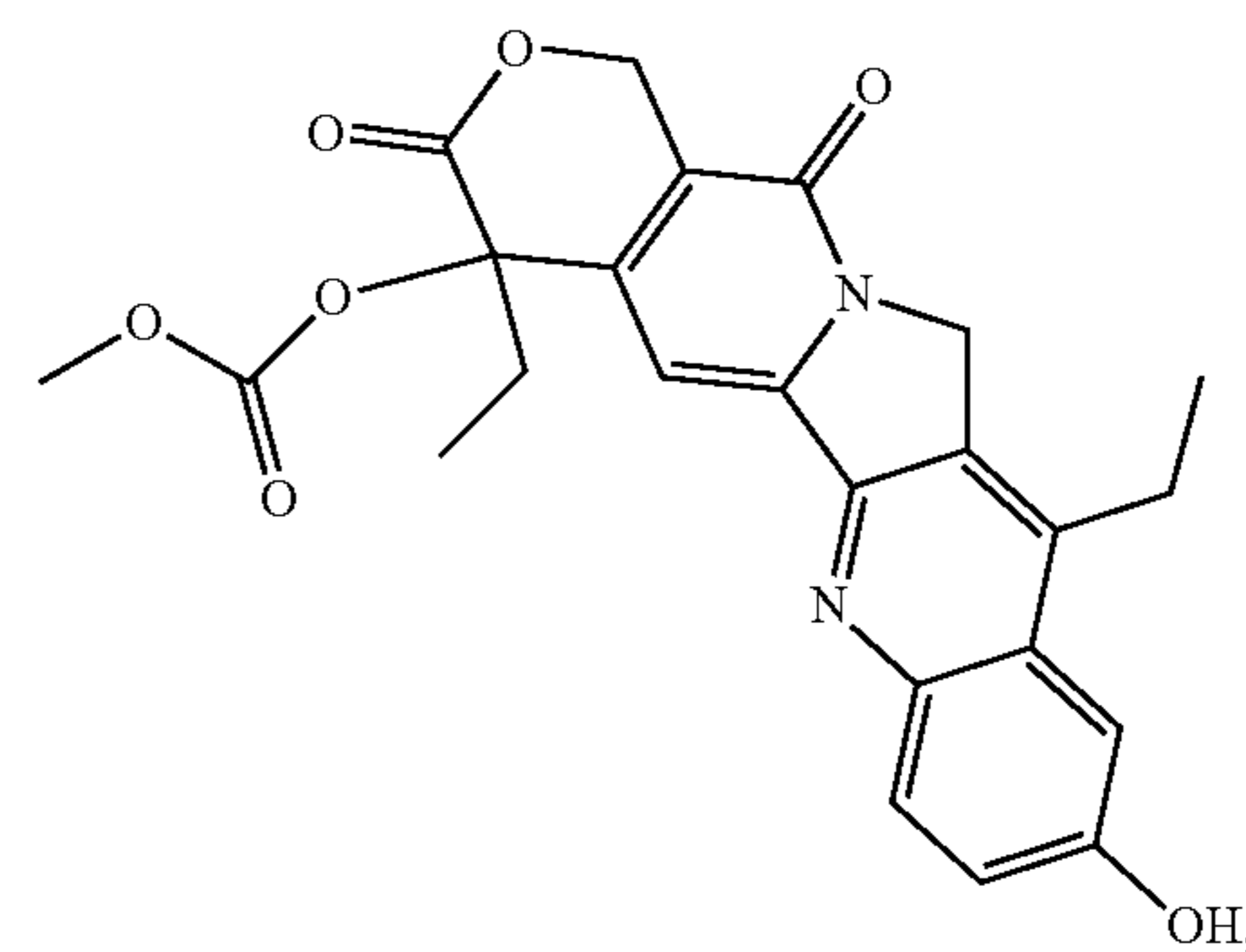
MAb-CL7-SN-38
