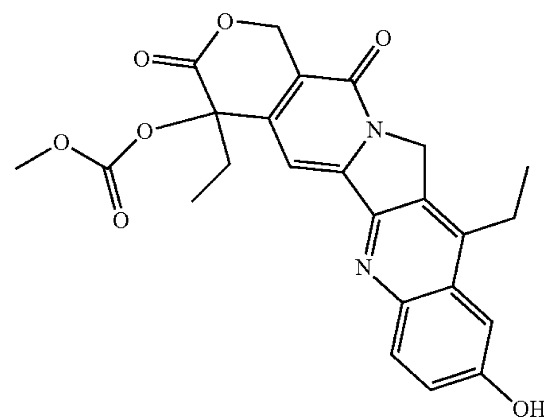
MAb-CL7-SN-38
