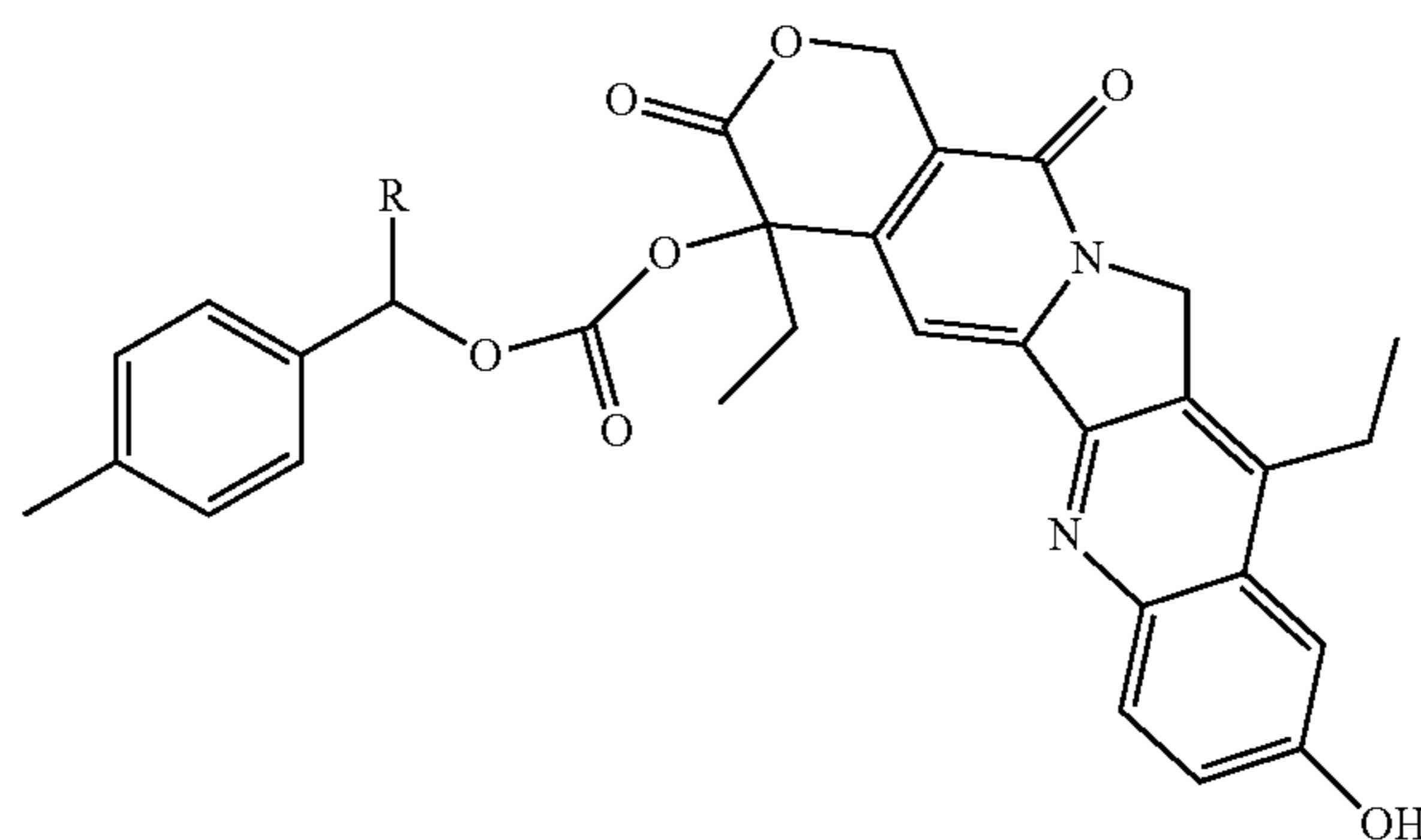
MAb-CLX-SN-38
