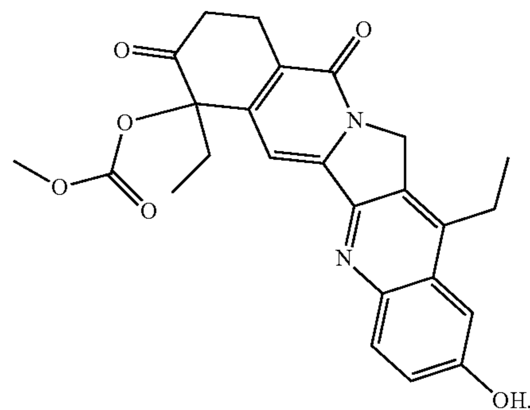
MAb-CLX-SN-38
