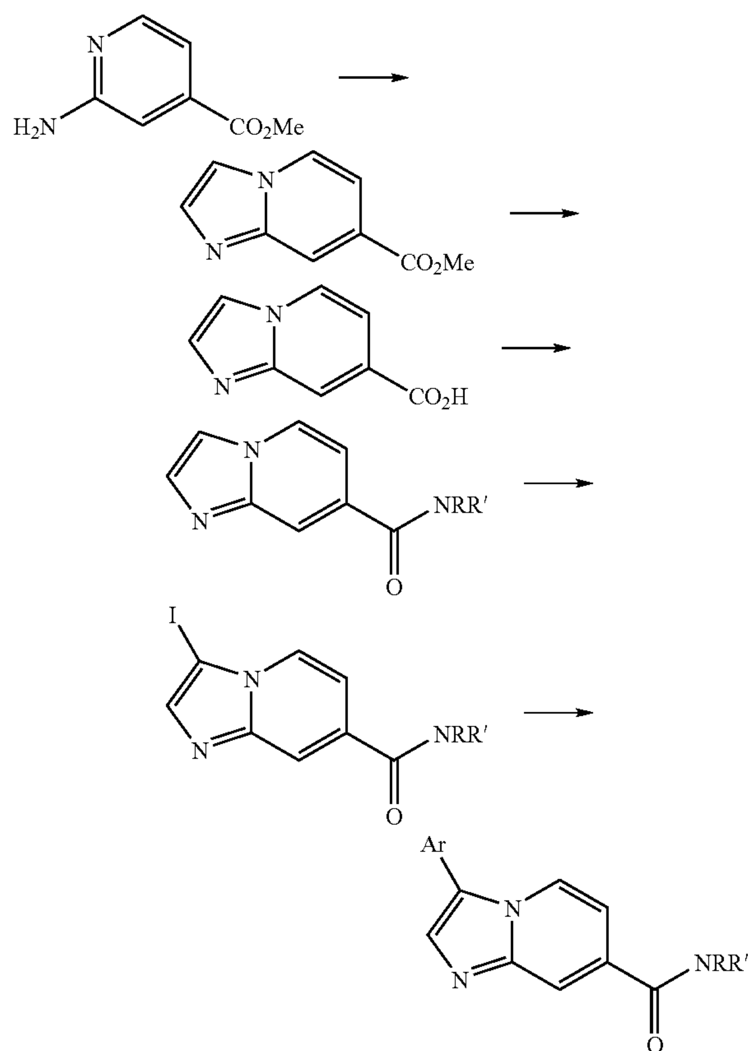
Scheme 1A
